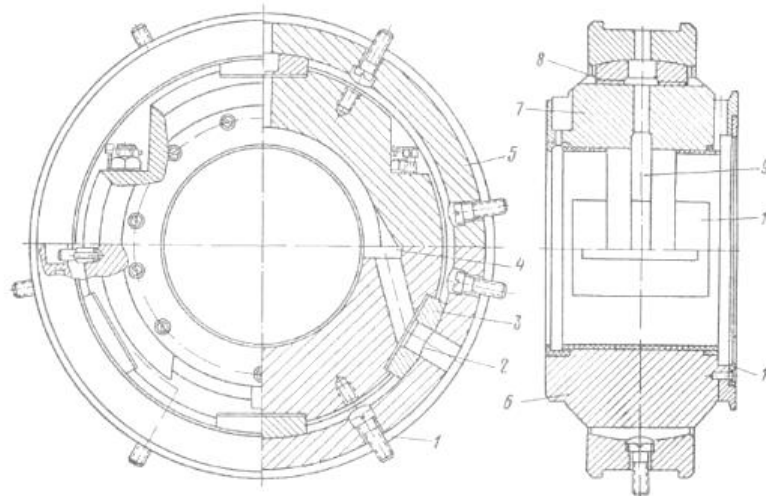
Рис. 2. Самоустанавливающийся подшипник
