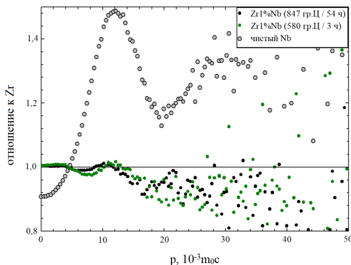
Рисунок 5. Относительные кривые спектров совпадающего ДУАЛ сплава Zr1%Nb, а также чистого Nb по отношению к чистому цирконию
