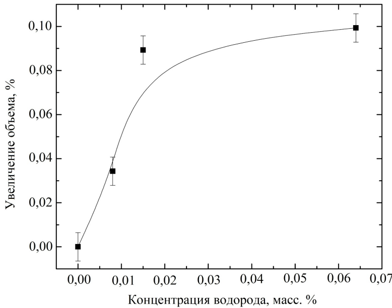
Рисунок 7. Зависимость относительного изменения объема элементарной ячейки ГПУ Zr от концентрации водорода в сплаве Zr1%Nb
