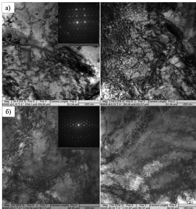
Рисунок 4. Изображения ПЭМ, полученные для образцов сплава Zr1%Nb, прокатанного до уровней деформации 2% (а) и 10% (б), соответственно
