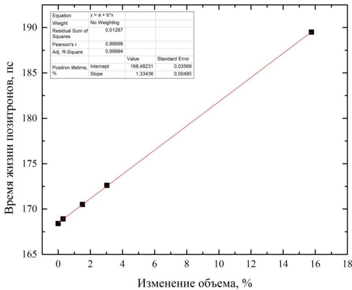
Рисунок 2. Зависимость времени жизни позитронов в решетке циркония от относительного увеличения объема решетки
