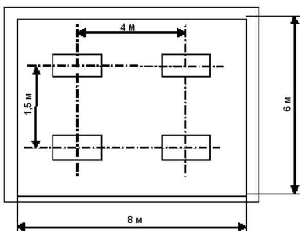
Рисунок 5.1 – Схема расположения светильников
