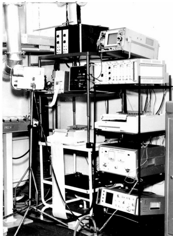
Рис. 2. Комплекс регистрирующей и измерительной аппаратуры сигналов АЭ при сварке изделий
