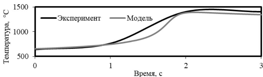
Рис. 1. Температурный режим протекания СВ-синтеза в системе В-С
