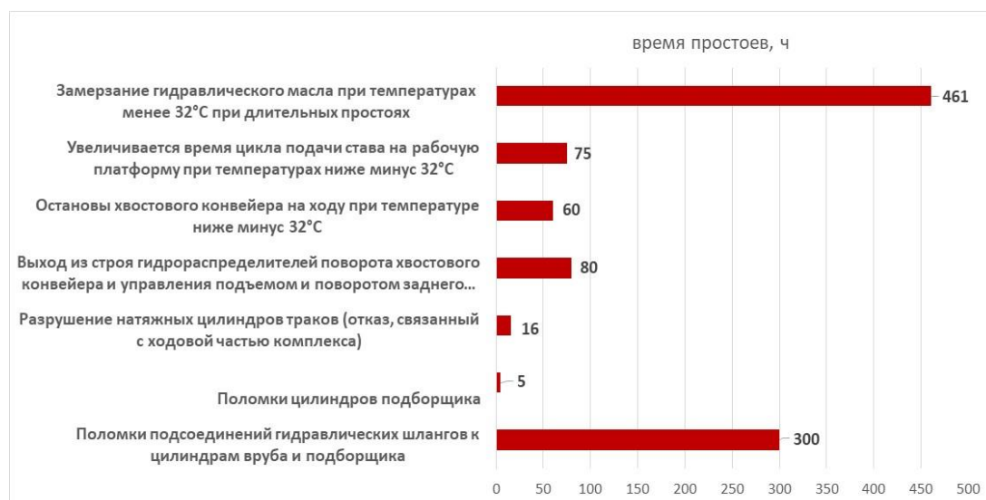
Рис. 2. Продолжительность простоев КГРП, связанных с ликвидацией отказов
