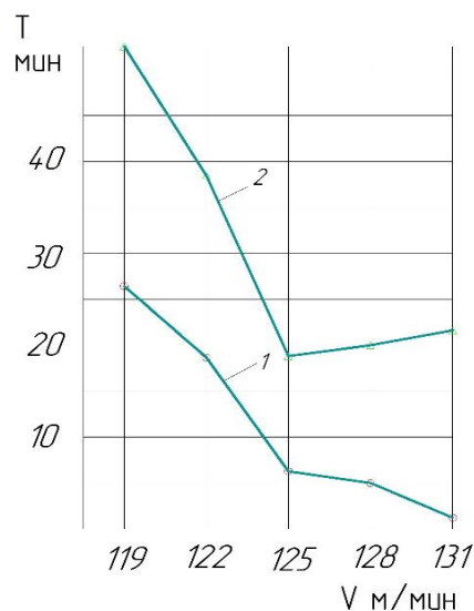
Рис.2. Влияние скорости резания и намагниченности резца на стойкость режущего инструмента при обработке стали 25, S = 0,15 мм/об 1. Ненамагниченный инструмент 2. Намагниченный инструмент
