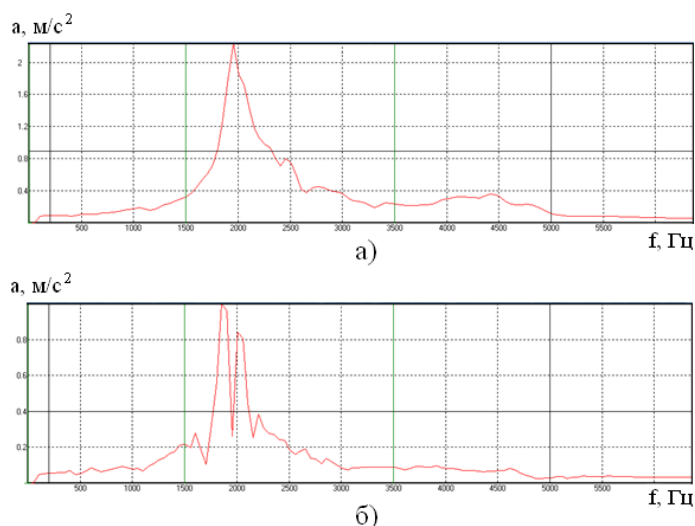
Рис. 2. Примеры спектров сигнала-отклика полученного при обследовании методом анализа возбужденных колебаний рамы бункера-перегрузателя БПС-25: а – дефект отсутствует; б – наличие трещины в металле
