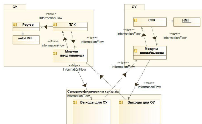
Рис. 1. Структура стенда
