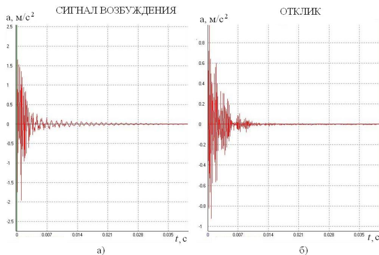
Рис. 1. Сигнал возбуждения (а), генерируемый импульсным источником колебаний, и отклик (б), регистрируемый датчиком пьезоакселерометром
