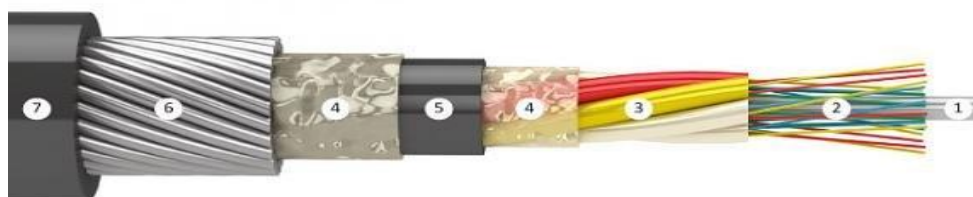
Рис.1. Структура оптоволоконного кабеля:
