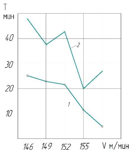
Рис.1. Влияние скорости резания и намагниченности резца на стойкость режущего инструмента при обработке стали 25, S = 0,11 мм/об 1. Ненамагниченный инструмент 2. Намагниченный инструмент
