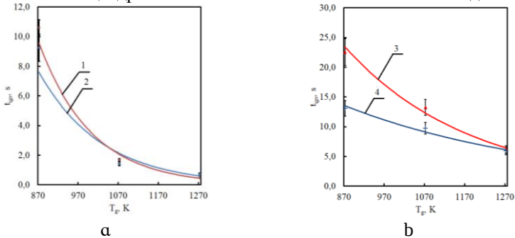
Рисунок 9 – Зависимости времен задержки зажигания от температуры окислителя: а - древесины (1 в составе топливной композиции, 2 – одиночной частицы); б - водоугольного топлива (3 – одиночной капли, 4 – в составе топливной композиции)
