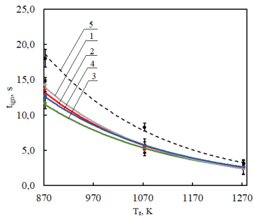
Рисунок 5 – Зависимости времён задержки зажигания био-водоугольных и водоугольных суспензий на основе длиннопламенного угля от температуры окислителя при начальном размере капель 2 мм (1 – с добавлением листьев березы, 2 – с добавлением хвои сосны, 3 – с добавлением хвои ели, 4 – с добавлением древесного угля, 5 – ВУТ без добавок)
