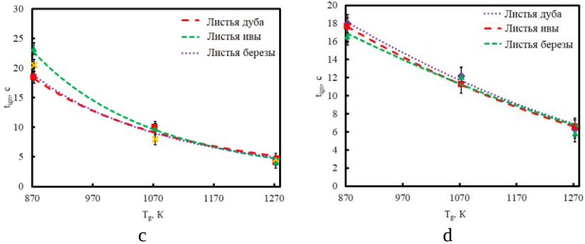
Рисунок 4 - Зависимости времён задержки зажигания капель био-водоугольного топлива от температуры внешней среды (а – тощий; б – бурый; в – длиннопламенный; д – антрацит)
