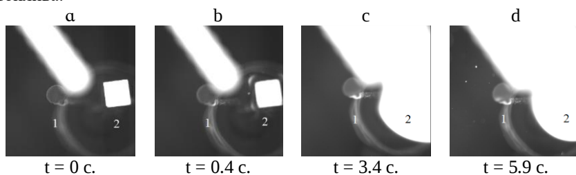
Рисунок 8 – Видеограмма процесса прогрева и последующего зажигания капли водоугольного топлива (1) и частицы древесины (2) в высокотемпературной среде ( T_g=1273K )
