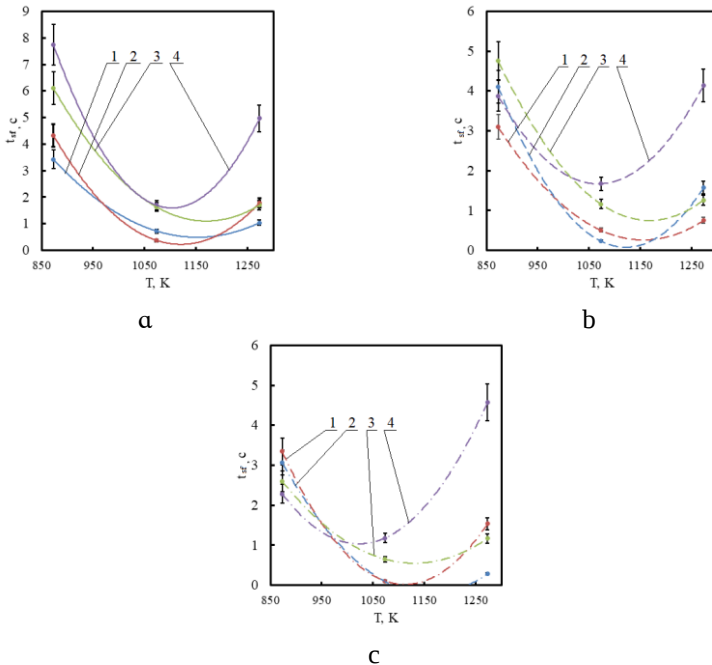
Рисунок 11 – Зависимость времени распространения пламени по поверхности частиц био-водоугольных суспензий с различными концентрациями биомассы (а - 5 %, b - 10 %, c - 15 %, ) на основе углей
