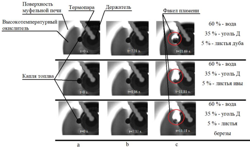
Рисунок 2 – Типичные кадры процесса воспламенения капель Био-ВУТ (на основе длинопламенного угля с добавлением листьев различных пород древесины) размером 2,5 мм при температуре окислителя T=1073 К (а - начало инертного нагрева капли Био-ВУТ, b – кадр, характеризующий окончание процесса влагоудаления с поверхности частицы био-водоугольного топлива, с – загорание частицы Био-ВУТ)
