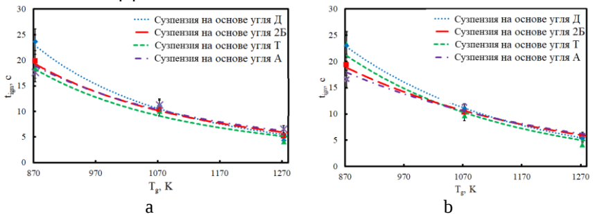
Рисунок 3 - Зависимости времён задержки зажигания капель био-водоугольных топлив, выполненных на основе углей различной степени метаморфизма с добавлением (а - листьев дуба, b - листьев ивы) от температуры окислительной среды
