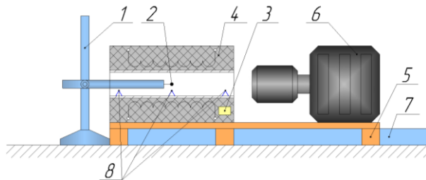
Рисунок 1 - Экспериментальный стенд
