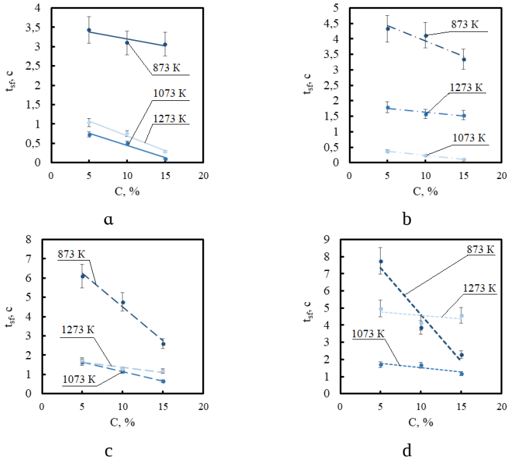
Рисунок 12 – Зависимость времени распространения пламени по всей поверхности частиц био-водоугольных суспензий на основе углей различных марок (а - бурый, б – длиннопламенный, с – тощий, d - антрацит) от концентрации лесного горючего материала
