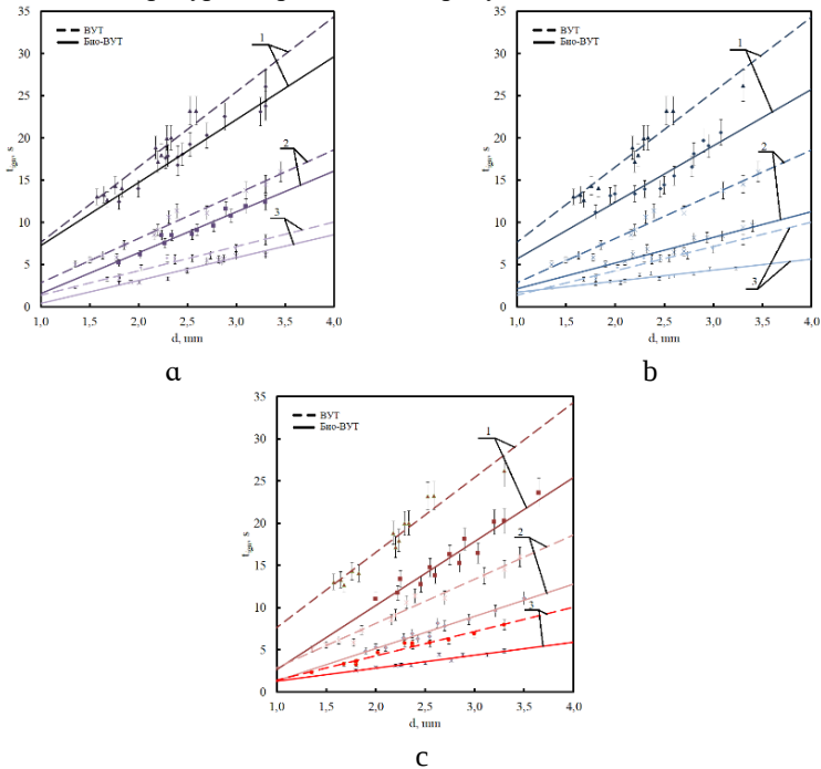
Рисунок 6 – Зависимости времени задержки зажигания капель Био-ВУТ на основе угля марки Д (а – смесь с добавлением листьев дуба, б – смесь с добавлением листьев ивы, с – смесь с добавлением листьев березы) от размера при разных температурах (1 – T = 873 K, 2 – 1073 K, 3 – 1273 K)
