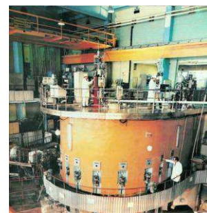
Исследовательский ядерный реактор ТПУ
