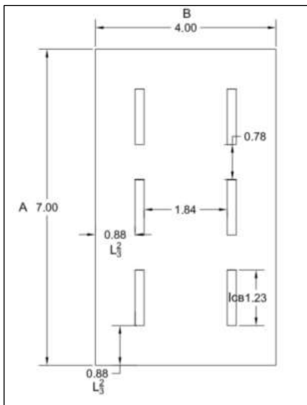
Рис. 30 План помещения и размещения на нем светильников
