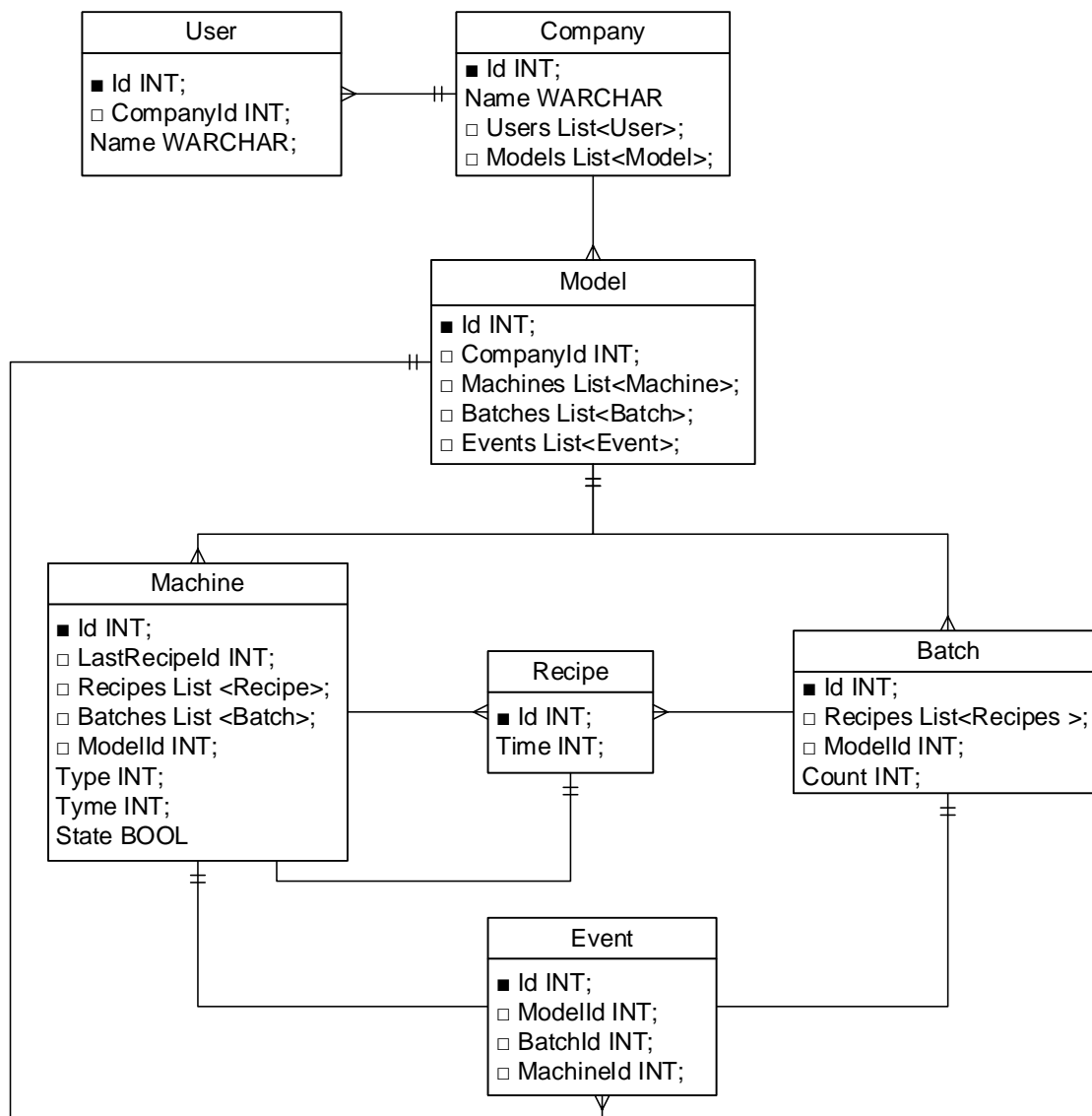
Рисунок 6 – Структурная схема БД
