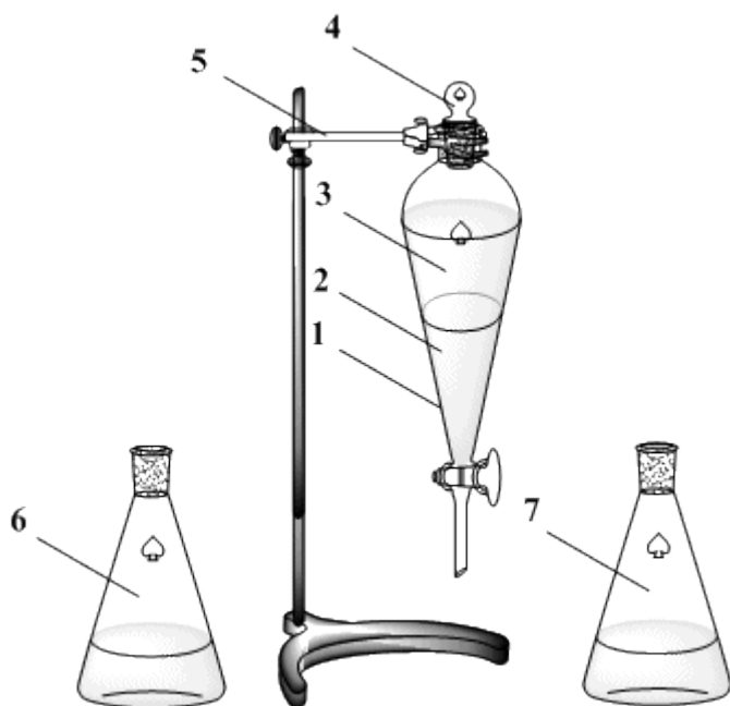
Рисунок 2.2.1 – Установка для проведения экстракции
