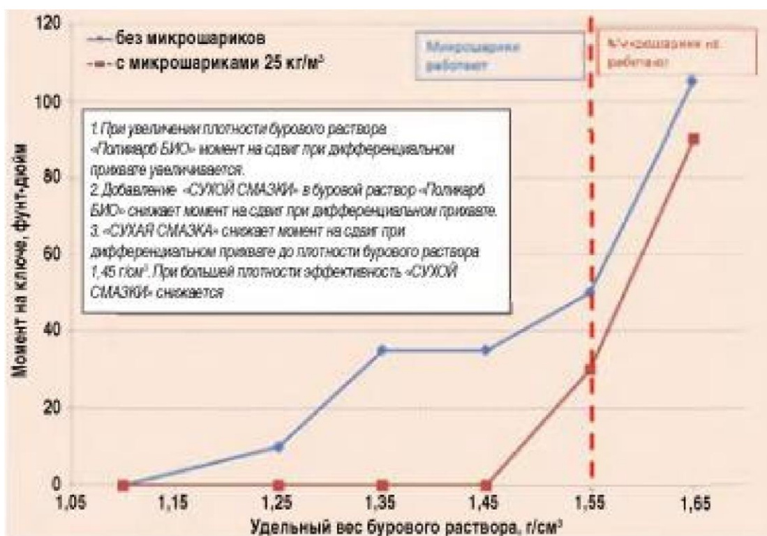
Рисунок 36 – Измерение момента на сдвиг при дифференциальном приводе с бурильным раствором "Поликарб БИО" без загрязнения активной твердой фазой
