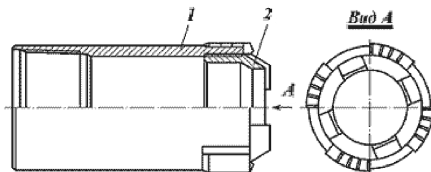
Рисунок 16 – Башмак-коронка:
