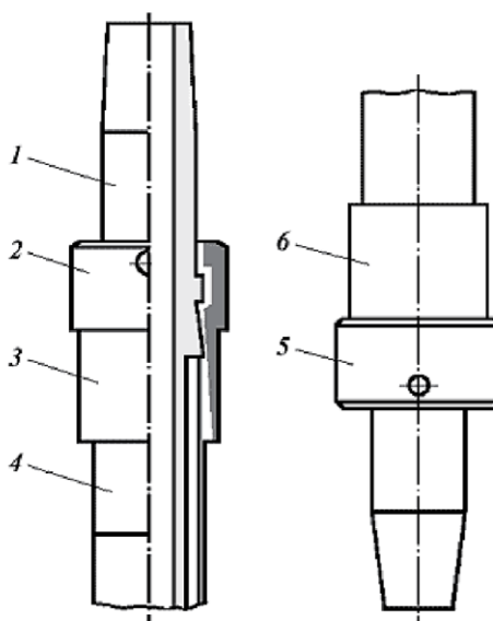
Рисунок 28 – Пакер заколонный типа ПЗ-168Ц:
