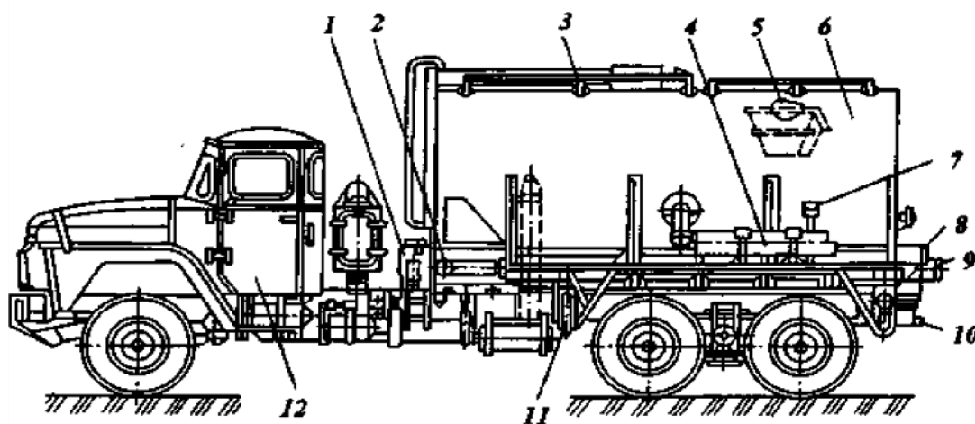
Рисунок 9 – Схема смесительной установки УС6-30Н:
