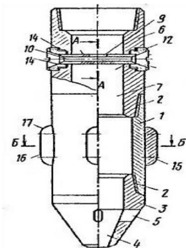
Рисунок 45 – Башмак обсадной колонны:
