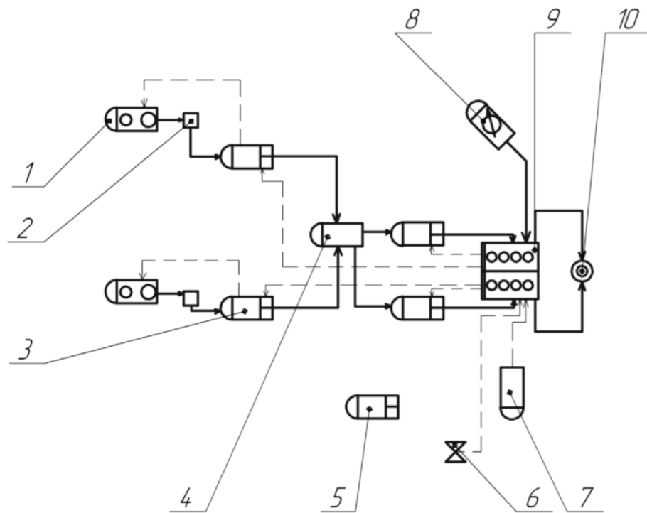
Рисунок 14 – Схема обвязки цементировочной техники с применением осреднительной установки:
