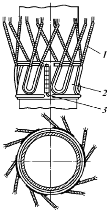
Рисунок 24 – Скребок корончатый типа СК:
