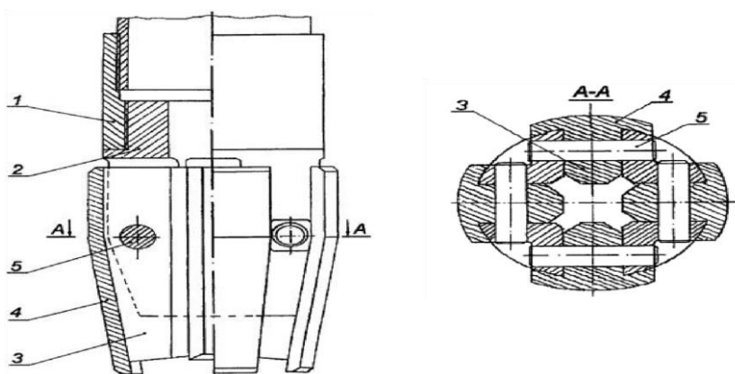
Рисунок 46 – Башмак обсадной колонны:
