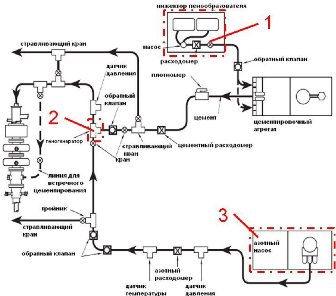
Рисунок 52 - схема пенного цементирования и дополнительное оборудование:
