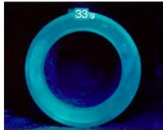
Пеноцемент после цикла опрессовок на 610 атм.
