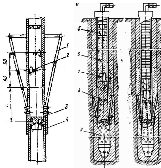
Рисунок 4 – Схема манжетного цементирования:
