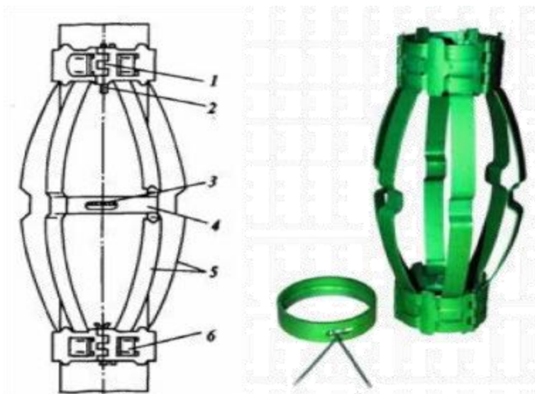
Рисунок 19 – Жёстко-упругий центратор:
