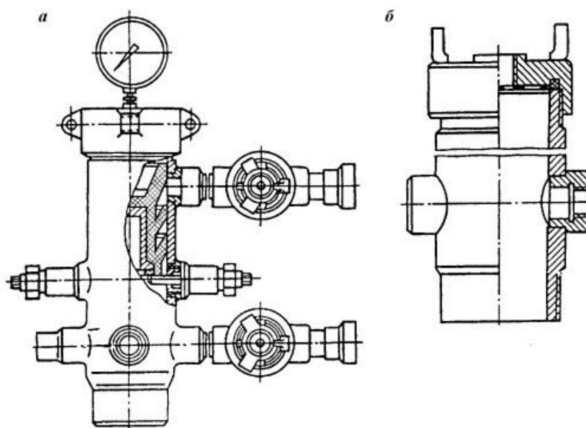
Рисунок 26 – Цементи́ровочные головки:
