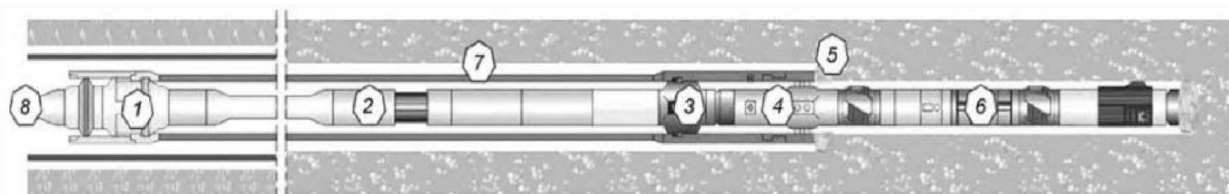
Рисунок 31 – Схема БХВ с применением РУС:
