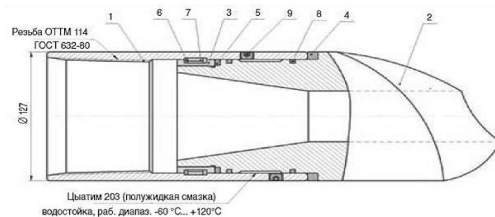
Рисунок 17 – Башмак колонный с возможностью вращения БК-Вр:
