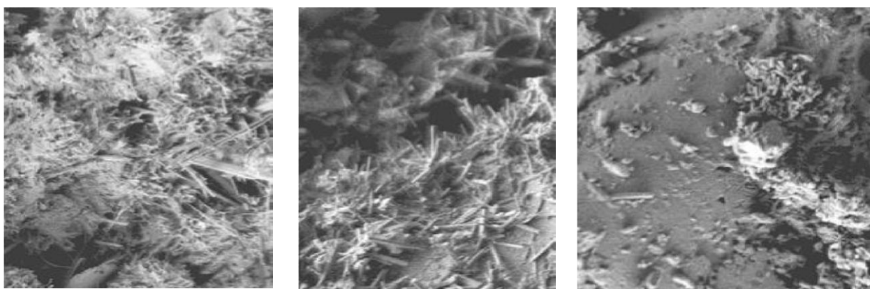
Рисунок 41– Микроструктура цементного камня, полученного из портландцемента:
