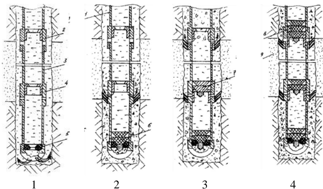
Рисунок 5 – Схема компоновки низа эксплуатационной колонны и технология селективного цементирования скважины:
