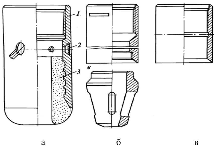
Рисунок 15 – Башмаки колонные:
