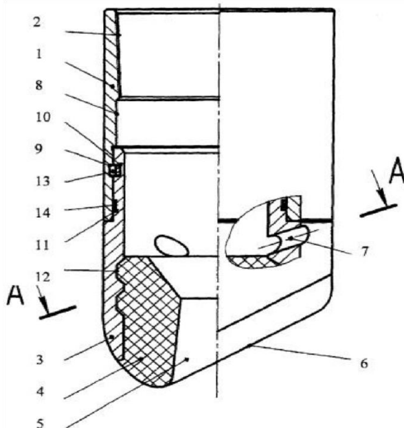
Рисунок 47 – Колонный башмак:
