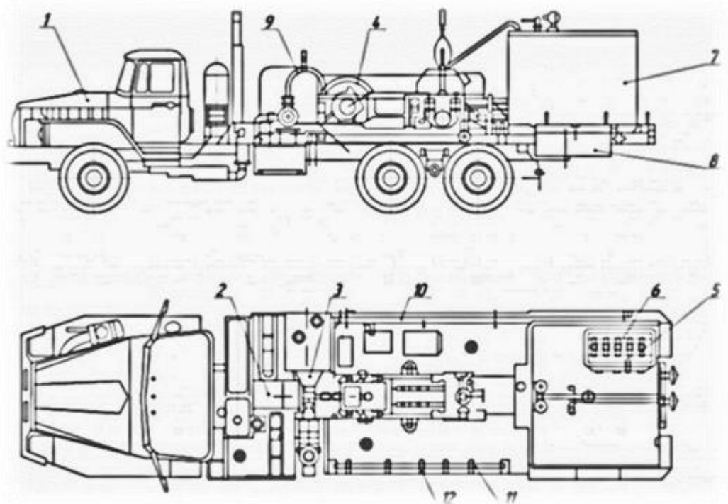
Рисунок 8 – Схема ЦА:
