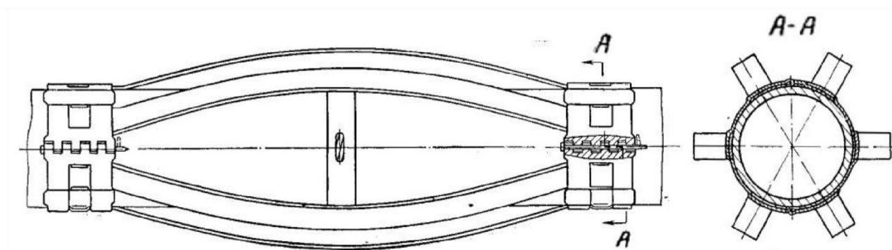
Рисунок 37 – Центрирующий фонарь
