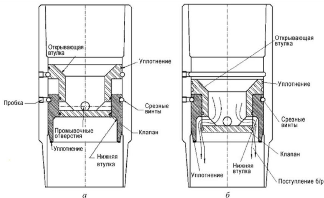
Рисунок 29 – Флотационная муфта:
