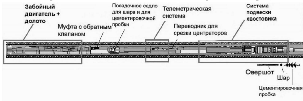
Рисунок 32 – Схема системы для направленного бурения на хвостовике
