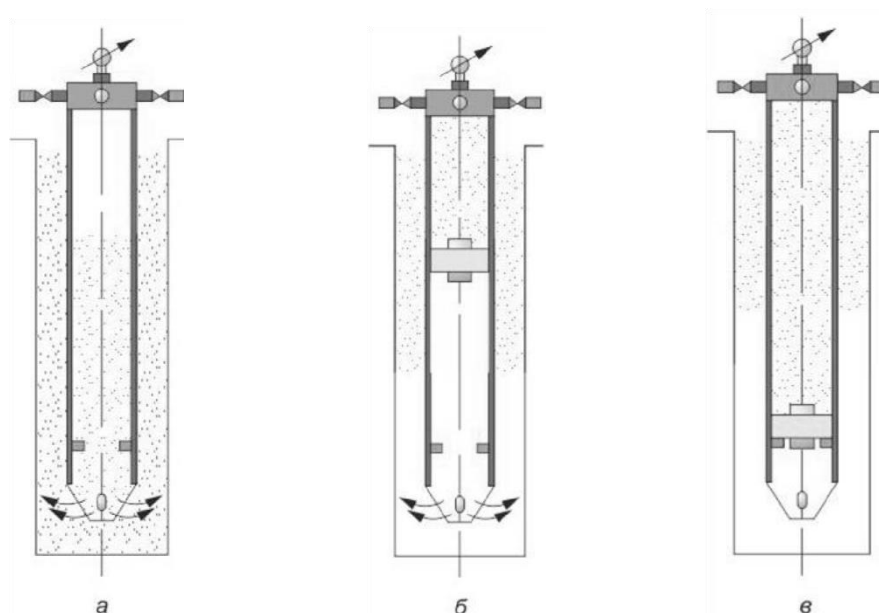
Рисунок 1 – Схема прямого одноступенчатого цементирования с одной пробкой:
