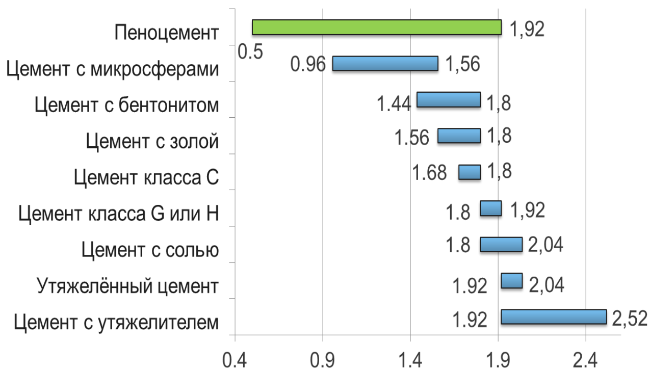
Рисунок 51 – диапазоны плотностей цементных систем, г/см 3
