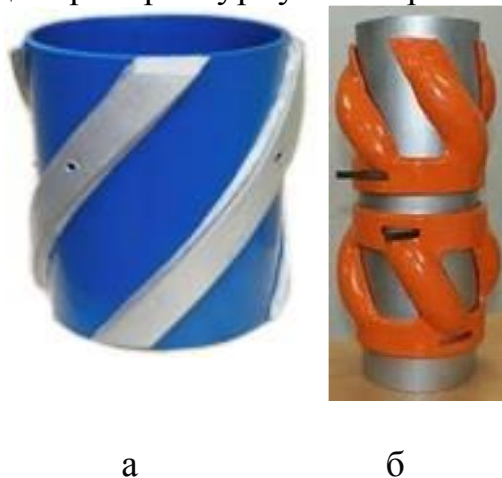
Рисунок 23 – Центраторы-турбулизаторы:
