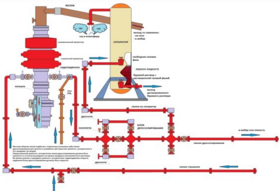
Рисунок 54 – Схема дросселирования
