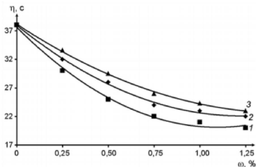
Рисунок 40 – Изменение условной вязкости \eta тампонажного раствора от содержания моносахаридов \omega , :
