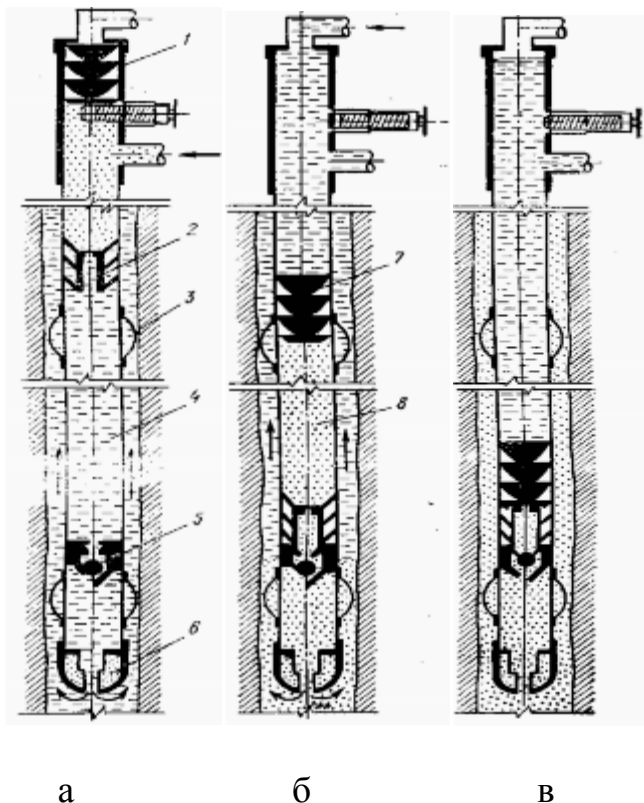
Рисунок 2 – Схема прямого одноступенчатого цементирования с двумя пробками:
