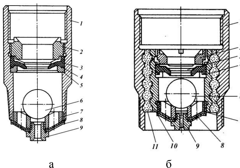
Рисунок 18 – Клапаны обратные:
