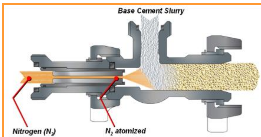
Рисунок 49 – технология получения пеноцемента
