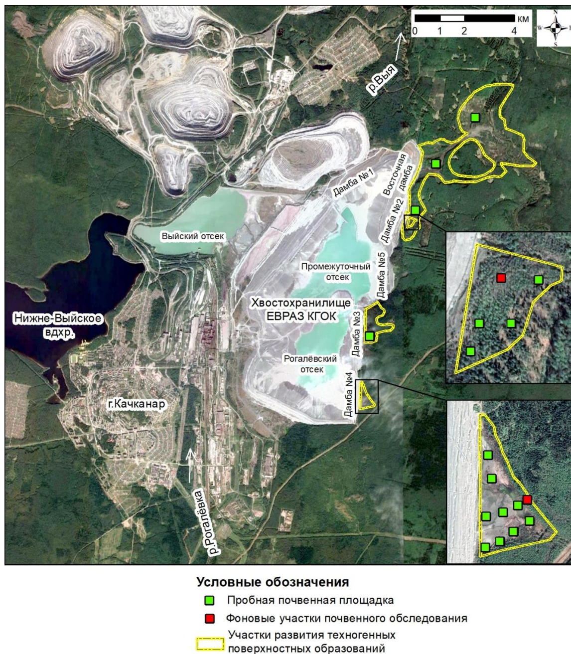
Рис. 1. Схема хвостохранилища АО «ЕВРАЗ КГОК»
