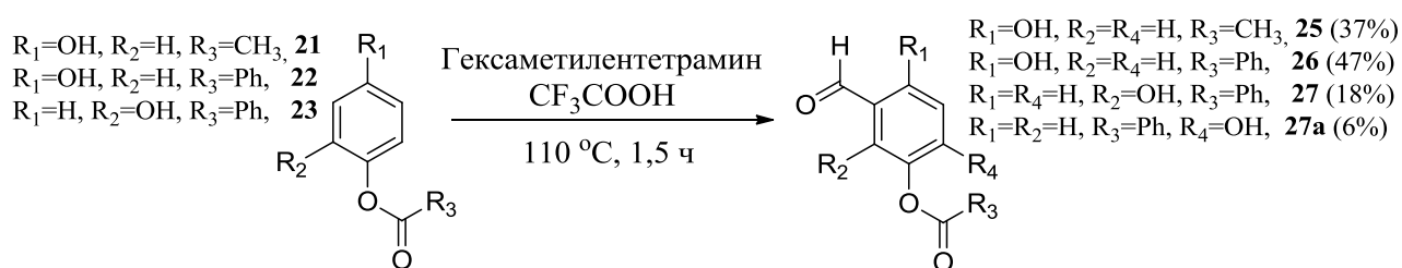
Схема 2 – Формилирование моноацилированных дифенолов
