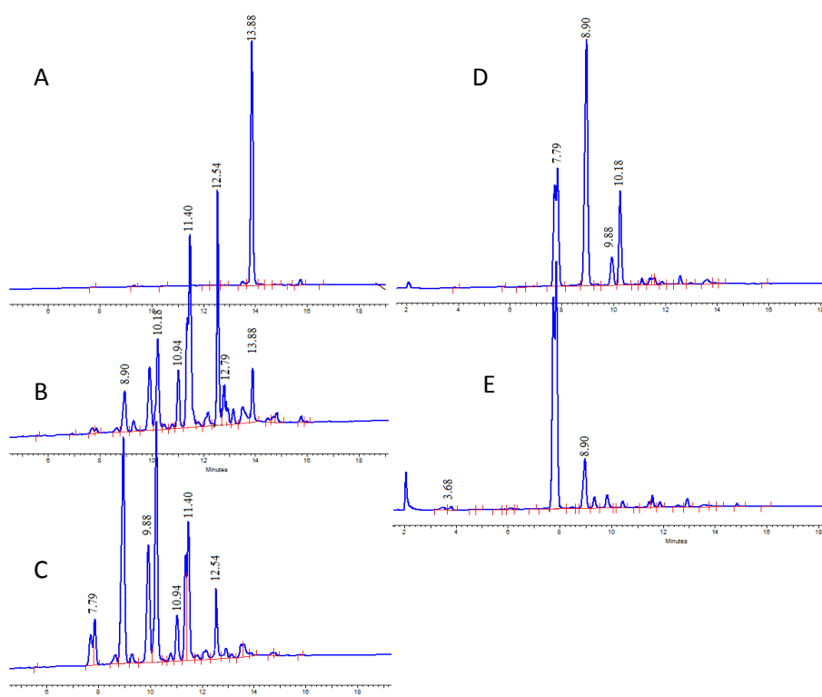
Рисунок 3 - ВЭЖХ анализ реакции гидролиза пентаацетилсалирепозида 43 при 16 °С А – 0ч, В – 1ч, С – 2ч, D – 4.5ч, E – 30ч.
