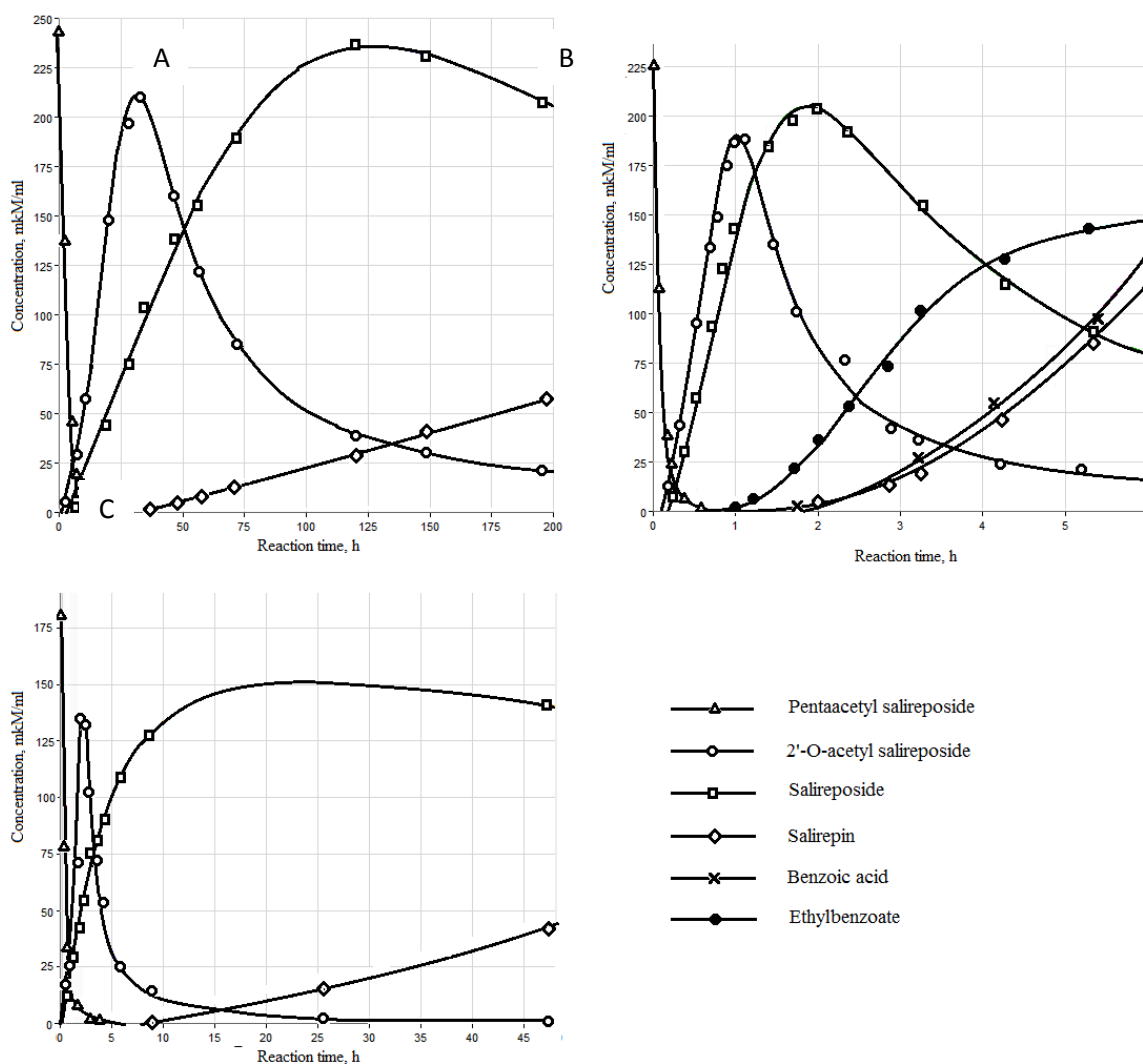
Рисунок 7 - Кинетические кривые реакции снятия ацетильных групп пентаацетилсалирепозида 43 , 16 °С (А), 30 °С (В), 50 °С (С). Концентрацию веществ в реакционной массе определяли методом ВЭЖХ при сравнении с предварительно построенными калибровочными графиками по каждому веществу.
