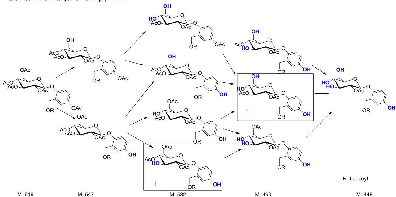
Схема 11 – Предполагаемые пути гидролиза ацетильных групп пенаацетилсалирепозида 43
