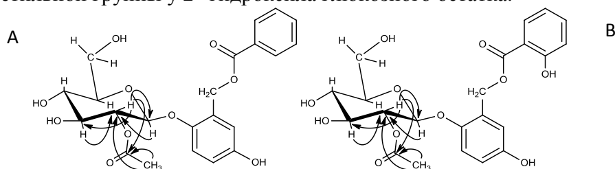
Рисунок 4 – HMBC анализ 2'-О-ацетил-салирепозидов 67 (A) и 2'-О-ацетил-салицилоил-салирепина 69 (B)
