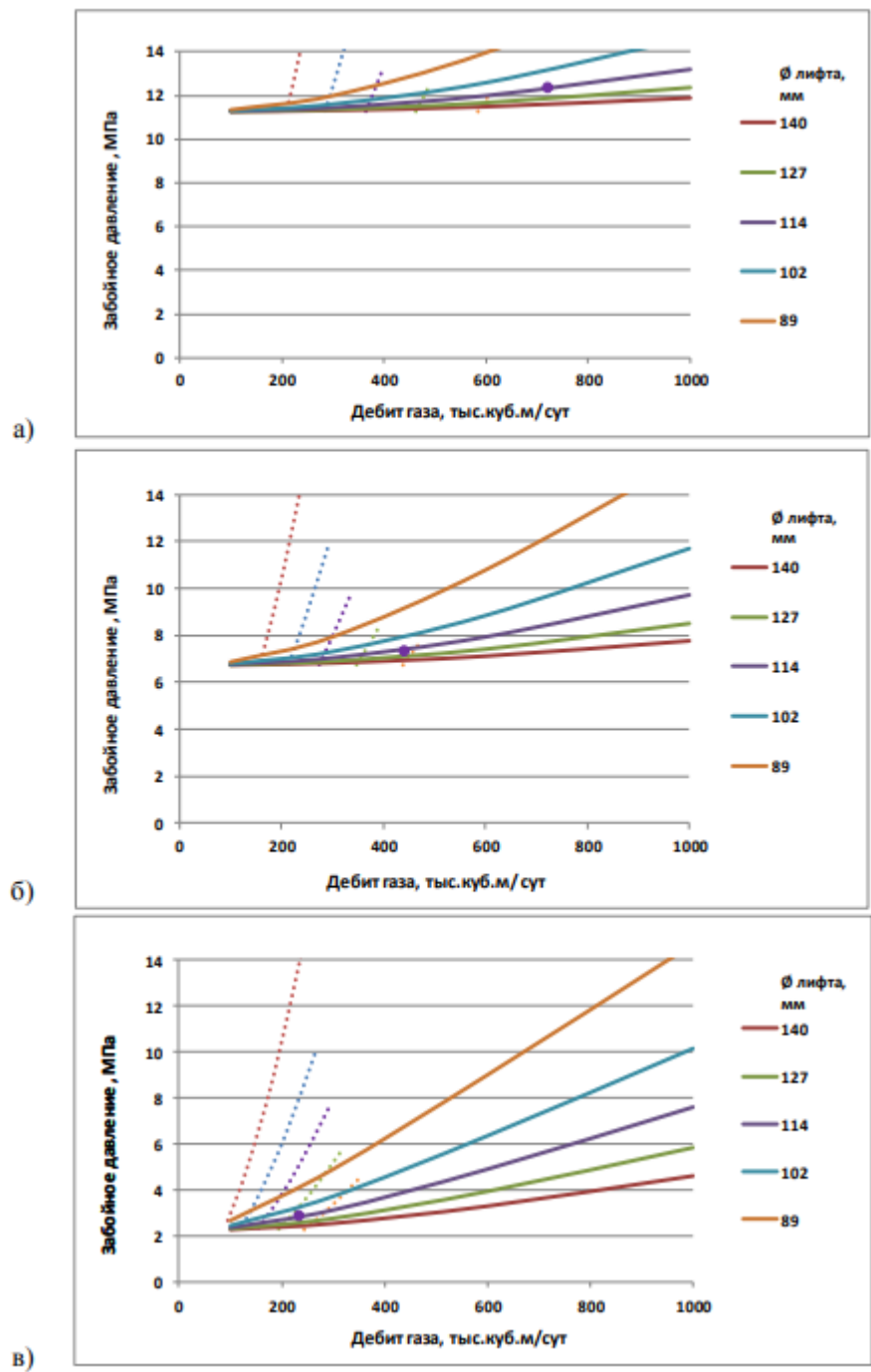
Рисунок 30 – Зависимость «забойное давление – дебит газа» при разных диаметрах лифта и устьевых давлениях (а – 10 МПа, б – 6 МПа, в – 2 МПа)
