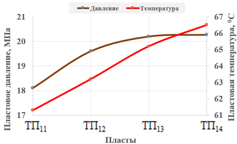
Рисунок 29 – Термобарические значения пластов танопчинской свиты
