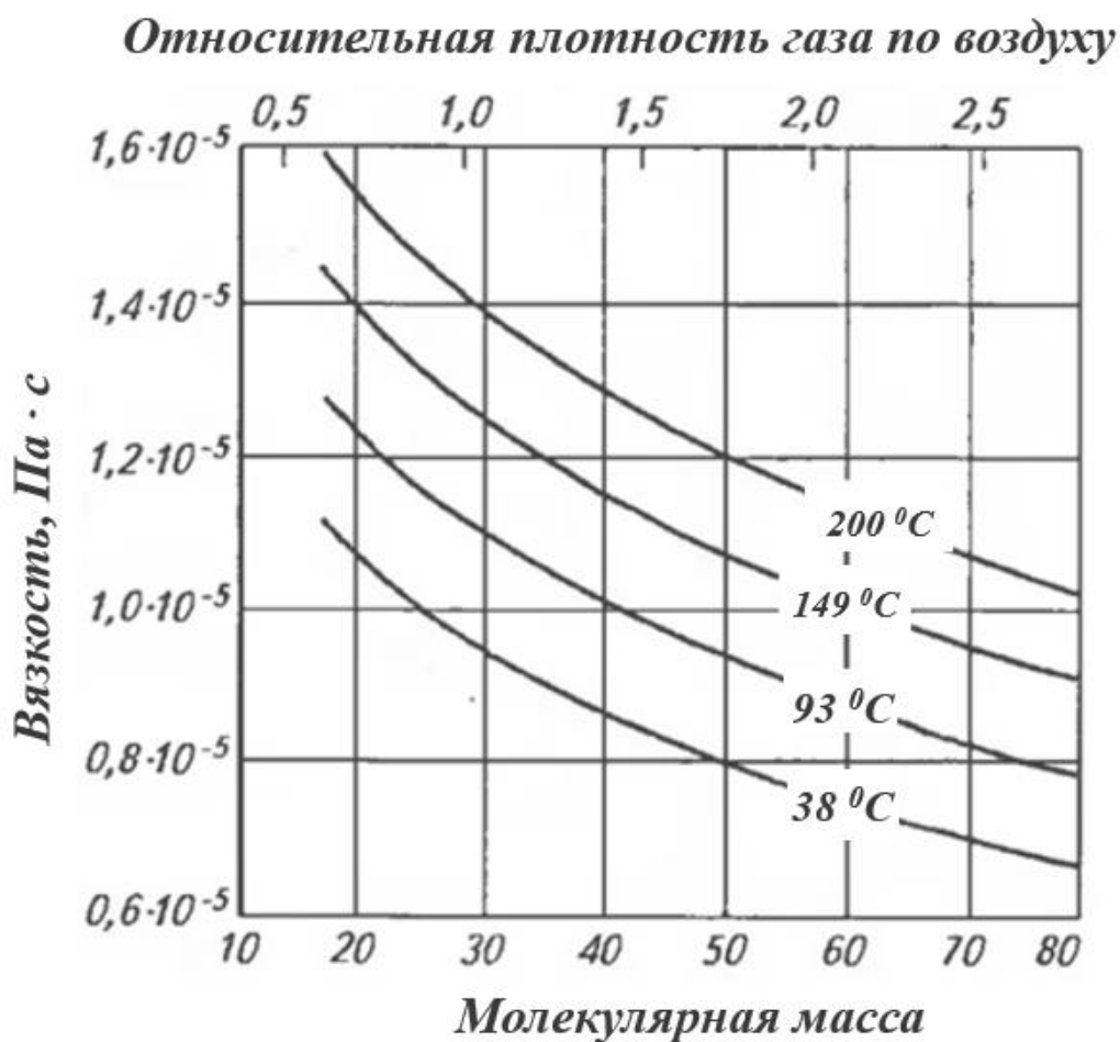
Рисунок 5 – Зависимость значения вязкости от температуры для природного газа при давлении ниже 11 МПа
