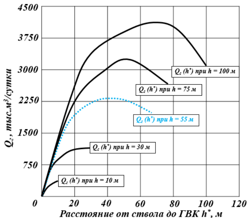
Рисунок 40 – Интерполяционная графическая зависимость для безводного дебита от h^* при h = 55 м
