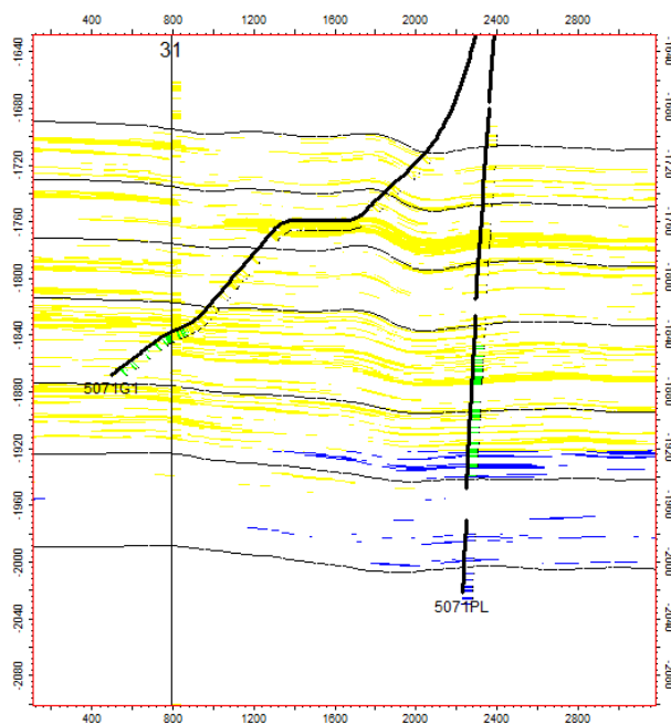
Рисунок 37 – Вскрытие пластов ТП 11 -ТП 14 с горизонтальным окончанием проектной скважиной 5071
