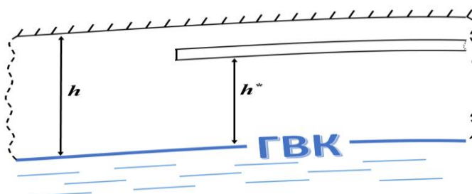
Рисунок 38 – Пример вскрытия горизонтальной скважиной пласта с наличием подошвенной воды
