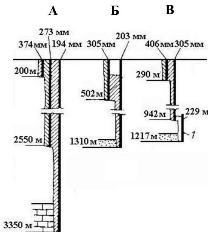
Рисунок 25 – Конструкции газодобывающей скважины месторождений Западной Сибири: А – Вуктыльское НГКМ, Б – Уренгойское ГМ, В – Медвежье ГМ; 1 - хвостовик
