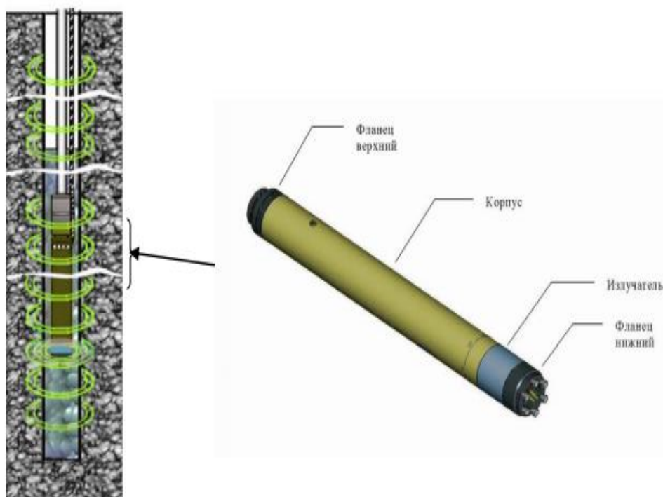
Рисунок 26 – Резонансно-волновая технология
