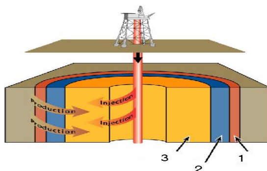
Рисунок 25 – Схема закачки ингибирующего состава [10]
