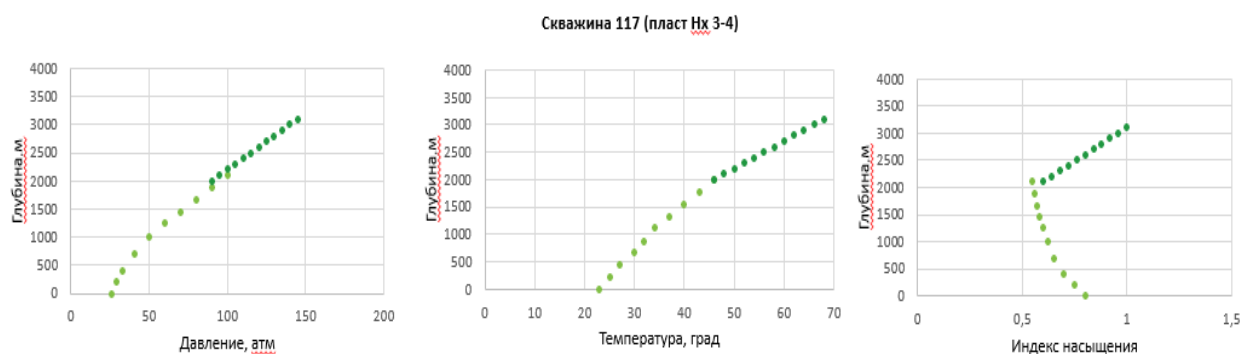
Рисунок 14 – Изменения давления, температуры и индекса насыщения по стволу скважины и НКТ
