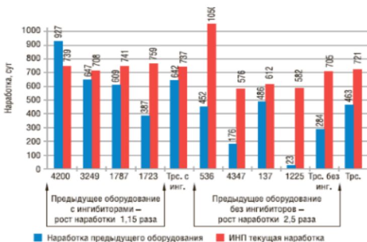
Рисунок 34 – Текущая наработка по восьми ЭЦН ТПП «Когалымнефтегаз», продолжающим работать
