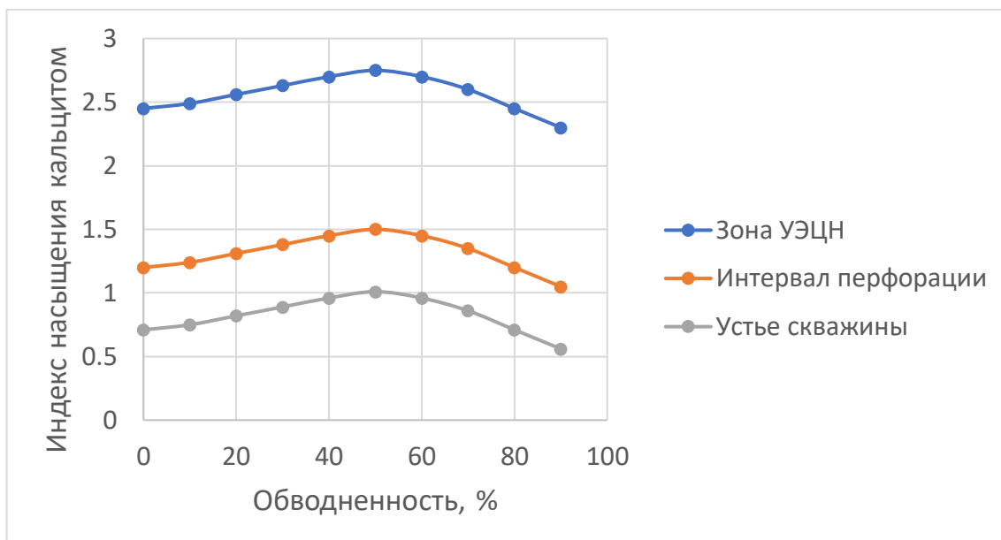
Рисунок 11 – Зависимость индекса насыщения добываемой воды кальцитом от обводнённости продукции для пласта НХ в ПЗП, на УЭЦН и на устье скважины
