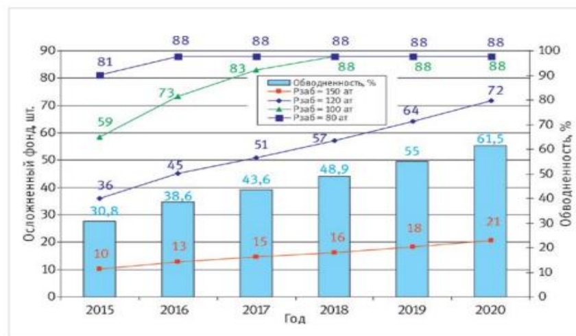
Рисунок 17 – Прогноз динамики осложненного фонда скважин по пласту Нх3-4
