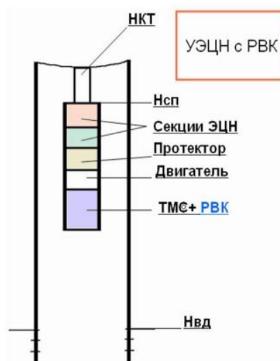
Рисунок 27 – Схема компоновки с УЭЦН
