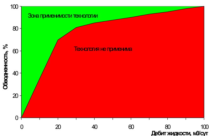
Рисунок 22 – Карта применимости технологии периодического дозирования [10]
