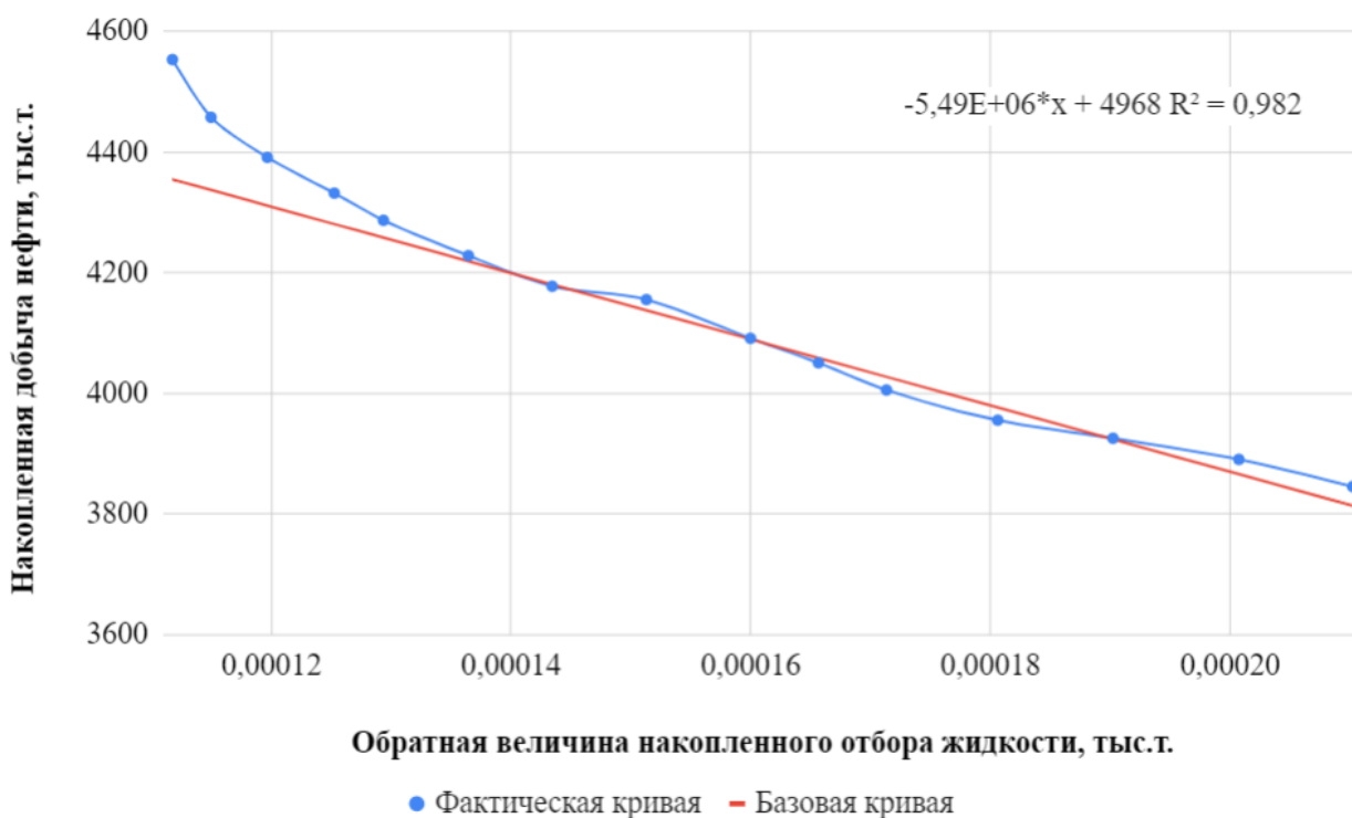
Рисунок 3 - Характеристика вытеснения по методу Камбарова Г.С.
