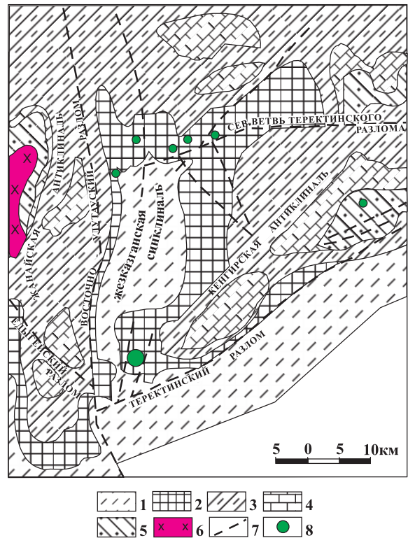
Рис. 2. Жезказганский металлогенический комплекс. Схема геолого-тектонического строения Жезказганского района (по С.Ш. Сейфулину, Н.Н. Нуралину, Л.В. Копятевич, К.Д. Джамину): 1) красные алевролиты, песчаники и известняки P; 2) серые и красные песчаники и алевролиты жезказганской продуктивной толщи C 2 -C 3 ; 3) серые известняки, песчаники, алевролиты и аргиллиты C 1 v-s; 4) серые известняки, доломиты, мергели C 1 t; 5) красные песчаники и сланцы, конгломераты D; 6) гранодиориты; 7) разломы; 8) месторождения и рудопроявления меди
