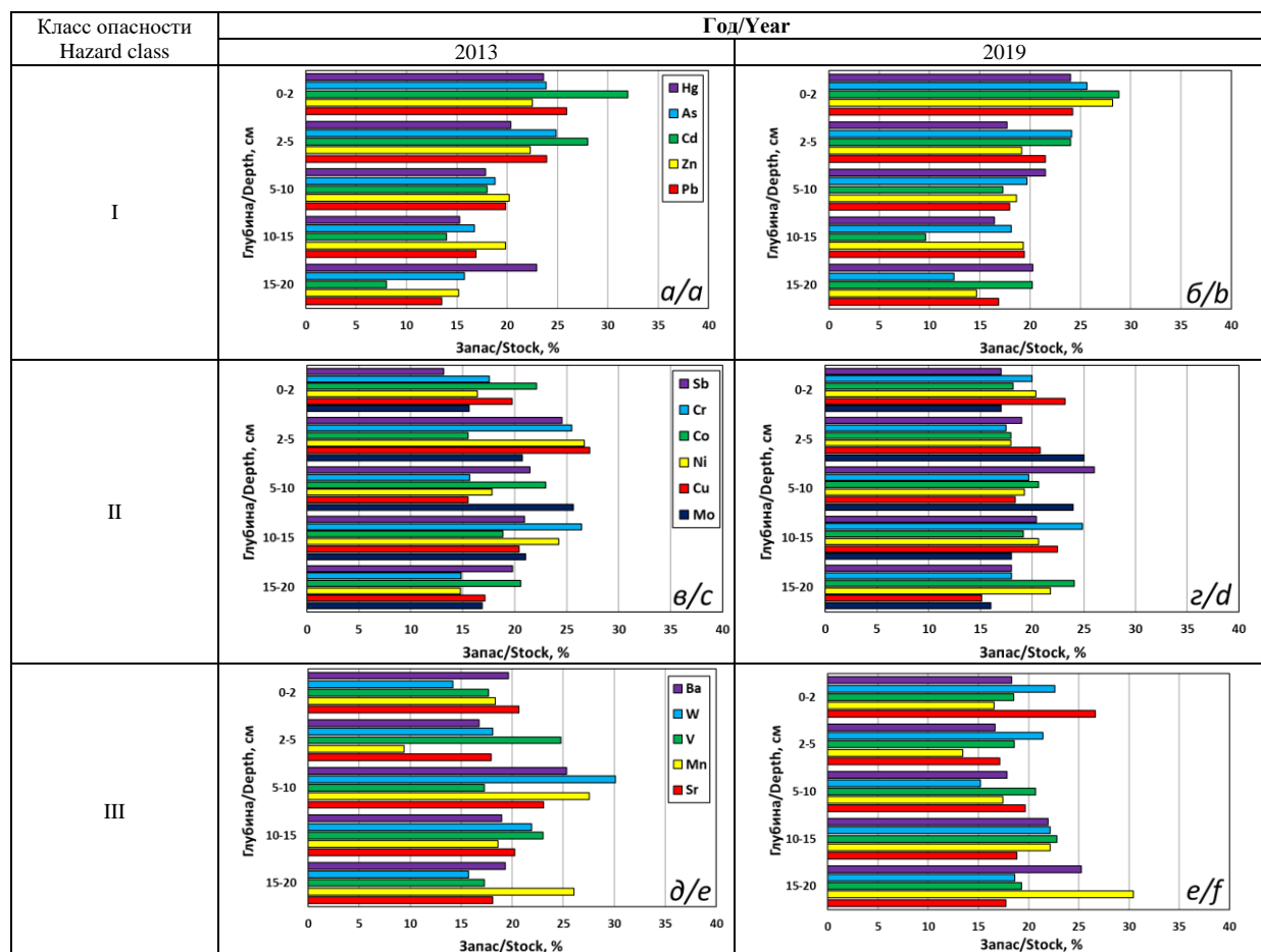
Рис. 2. Запас элементов I (а, б), II (в, г) и III (д, е) классов опасности в 20-см почвенном профиле природных экосистем в районе Белоярской АЭС в 2013 и 2019 гг., %
