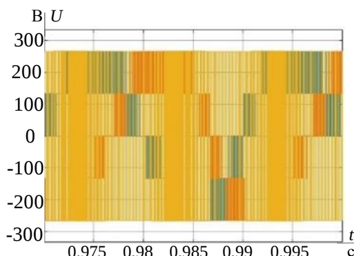
Рис. 19. Фазные напряжения при безаварийном варианте работы и двухполярном алгоритме управления Fig. 19. Phase voltages during fault-tolerant operation and bipolar control algorithm
