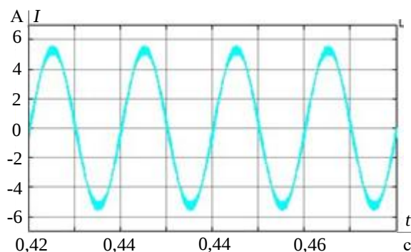
Рис. 4. Осциллограмма тока при f=50 Гц и f_{on}=10 кГц и треугольном опорном сигнале
