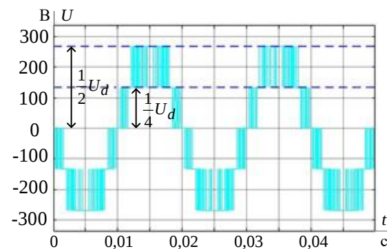
Рис. 9. Фазное напряжение для пятиуровневой ШИМ при f=50 Гц
