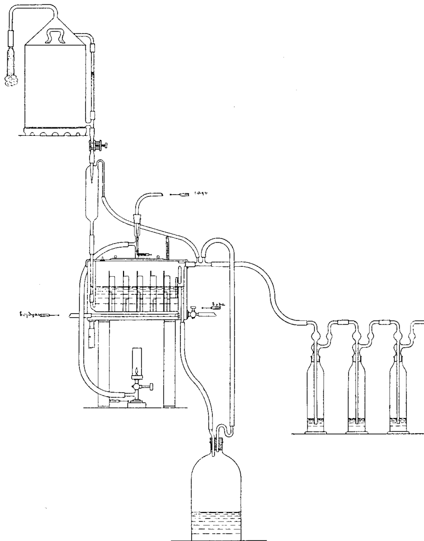
Непрерывно дѣйствующій бродильный аппаратъ системы С. В. Лебедева въ собранномъ видѣ.
