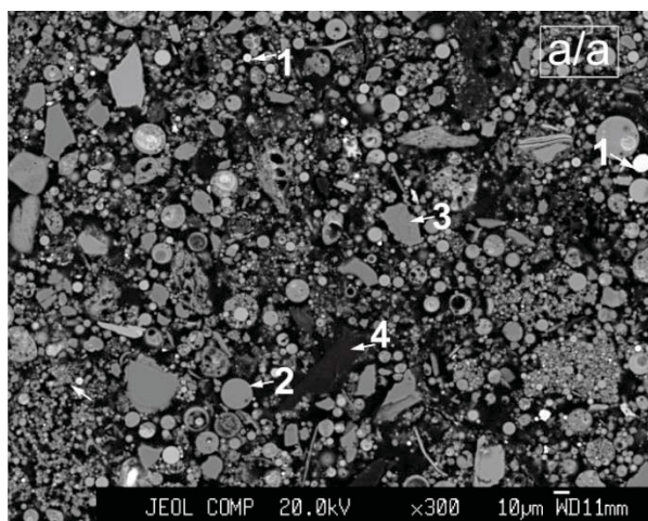
Рис. 4. Вид твердого осадка снежного покрова, отобранного на промышленной зоне г. Усолье-Сибирское (а) и в районе городской зоны (б). Изображение в обратно рассеянных электронах. Увеличение 300×. 1 – металлические сферулы ( 3Al_2O_3 \cdot 2SiO_2 с примесями Fe, Ti), 2 – алюмосиликатные микросферулы, муллит ( Fe_2O_3 ), 3 – кальцит и доломит ( CaCO_3 , CaMgCO_3 ), 4 – сажистая фаза, уголь (C), 5 – кварц ( SiO_2 )
