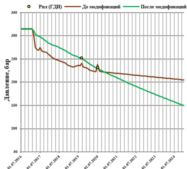
Рис. 4. Результаты адаптации пластовых давлений по скважинам
