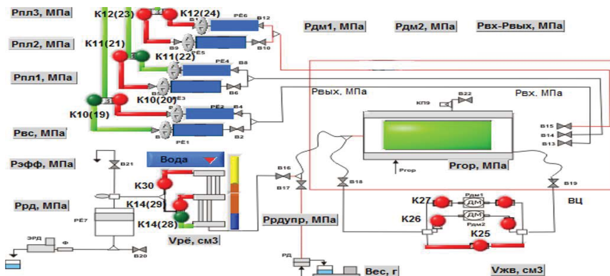
Рис. 1. Схема проведения лабораторных исследований водогазового воздействия на ядре
