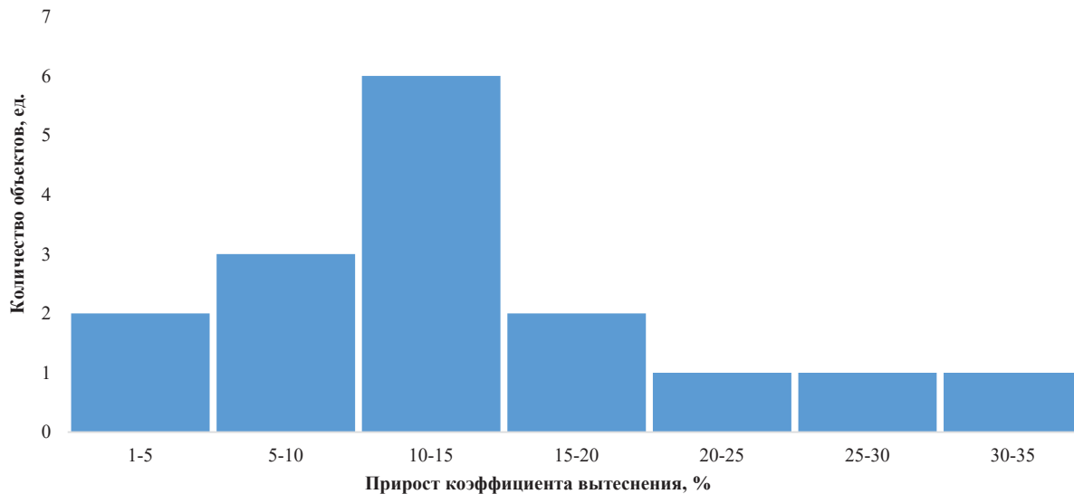
Рис. 6. Распределение прироста коэффициента вытеснения при заводнении растворами полимеров на объектах аналогов
