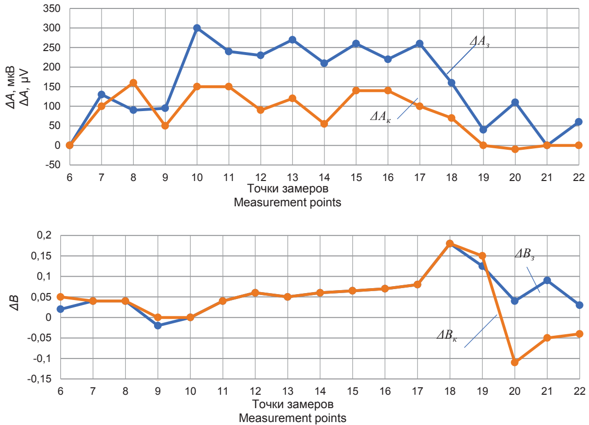
Рис. 6. Графики изменения разностных параметров по длине лавы 25-101 Fig. 6. Graphs of changes in the difference parameters along the length of the lava 25-101
