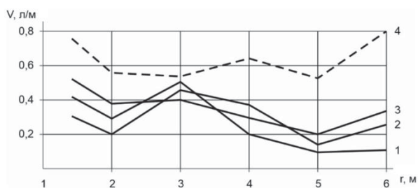
Рис. 9. Результаты измерений методом выхода штыва: 1–3 – вне зоны ПГД; 4 – в зоне ПГД; 1 – забой лавы в 30 м от конвейерной печи; 2, 3 – вентиляционная печь в борт лавы; 4 – забой лавы в 7 м от конвейерной печи
