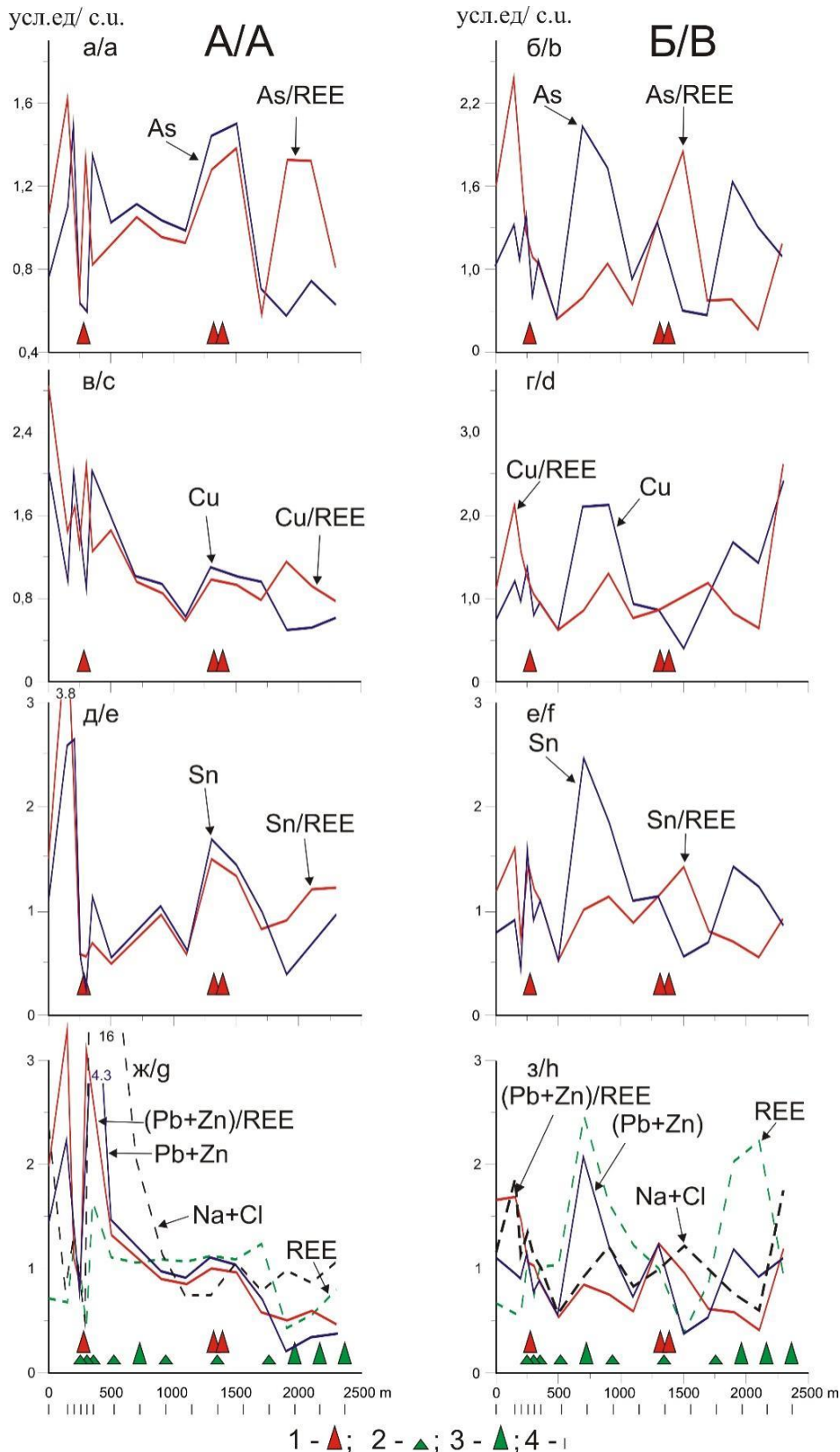
Рис. 4. Распределение концентраций рудных элементов и комплексных показателей над центральной залежью Турунтаевского полиметаллического рудопроявления по результатам опробования почвенного воздуха (А) и снежного покрова (Б): 1 – рудная скважина; 2 – редкий кустарник; 3 – лес; 4 – пункты опробования снежного покрова и почвенного воздуха
