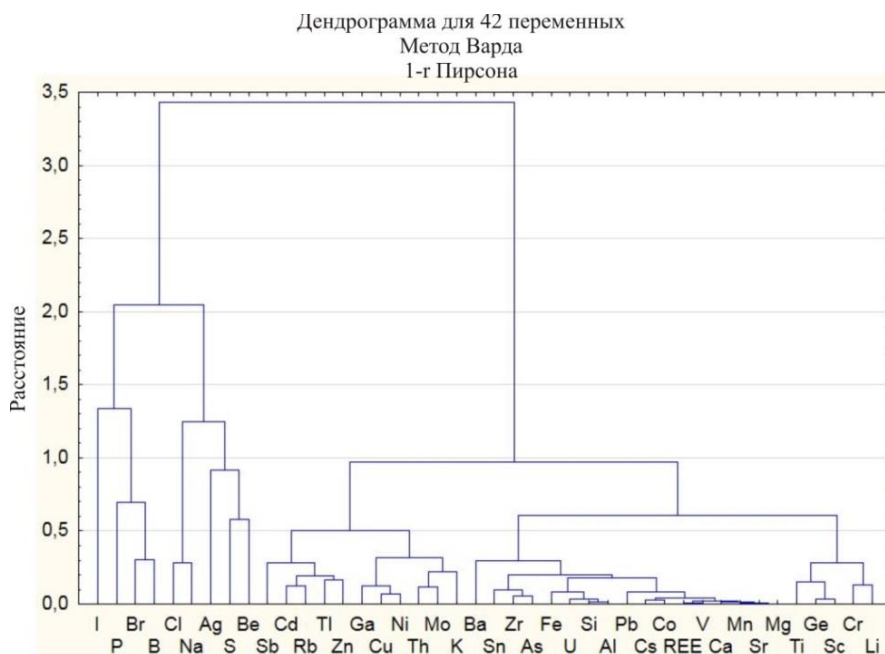
Рис. 3. Результаты кластер-анализа по снеготалой воде Fig. 3. Results of cluster analysis for snow melted water
