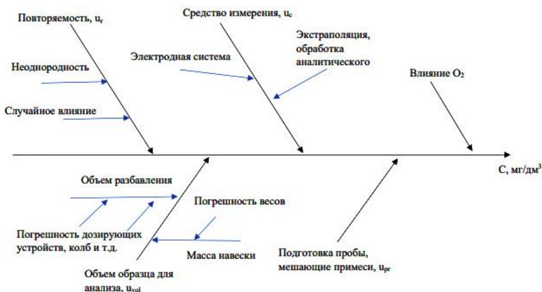
Рисунок 17 - Причино-следственная диаграмма факторов, влияющих на точность измерения селенит-иона методом вольтамперометрии
