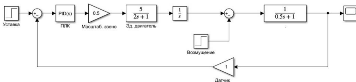
Рисунок 18 – Структурная схема автоматического регулирования расхода с возмущением
