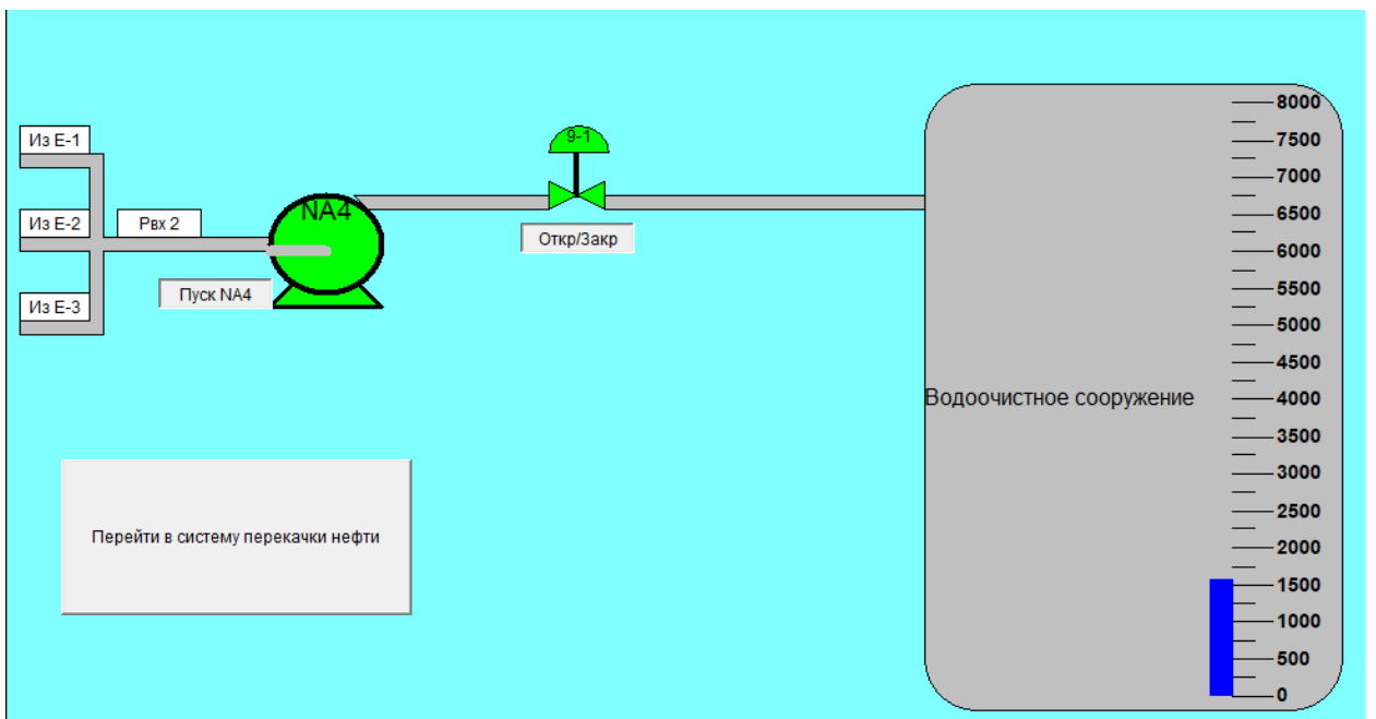
Рисунок 16 - Процесс разделения
