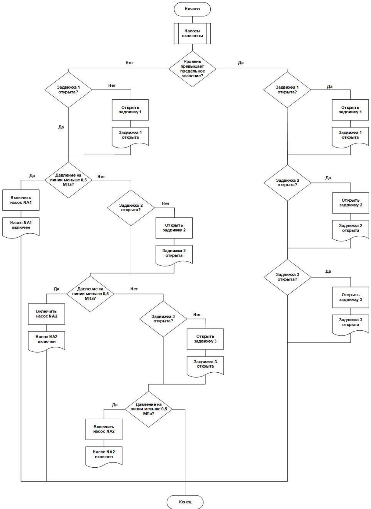
Рисунок 17 - Алгоритм пуска/остановы насоса АС ДНС
