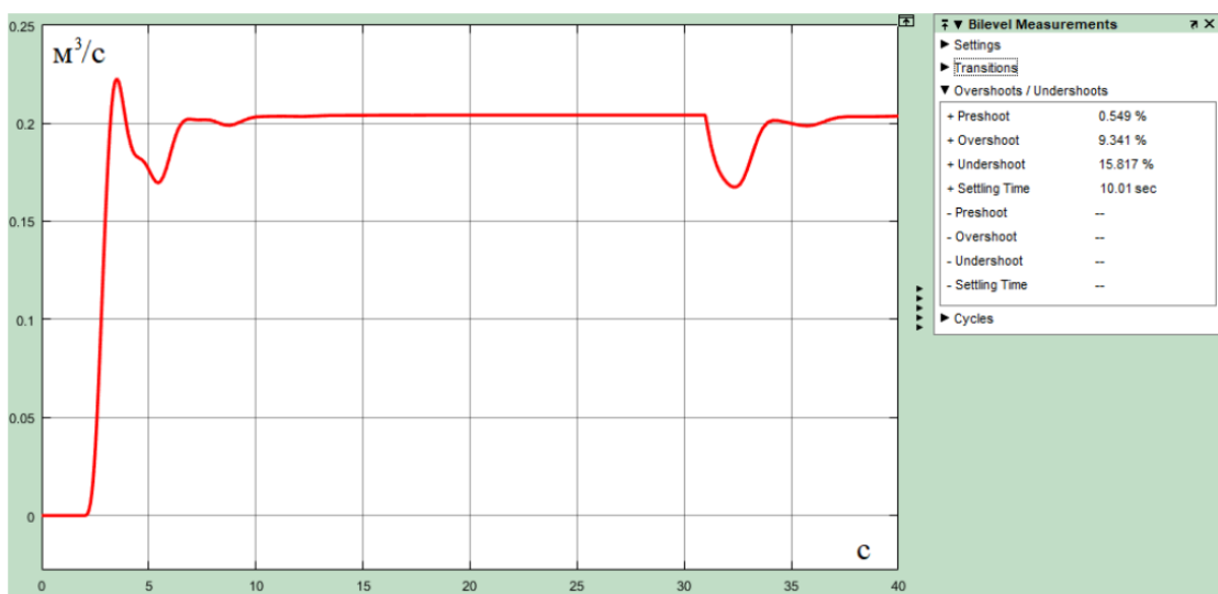
Рисунок 19 – График переходного процесса
