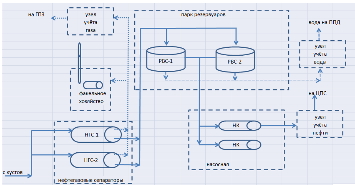
Рисунок 1 – Общая схема ДНС
