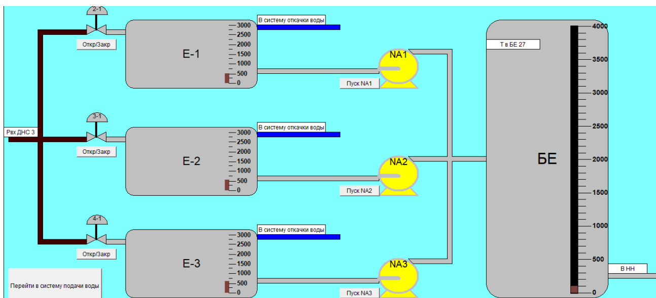
Рисунок 14 – Общая мнемосхема ДНС с УПСВ
