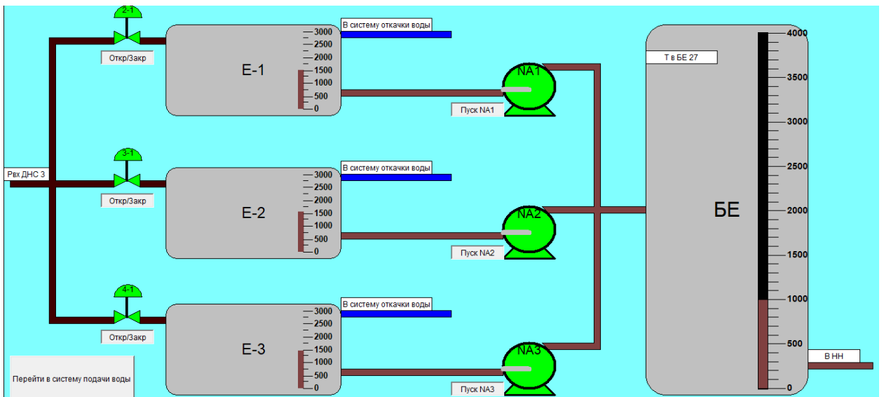
Рисунок 15 - Процесс разделения
