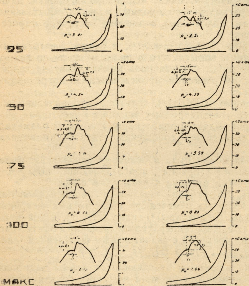
Фиг. 15. Индикаторные диаграммы дв-ля ЮМТ.
