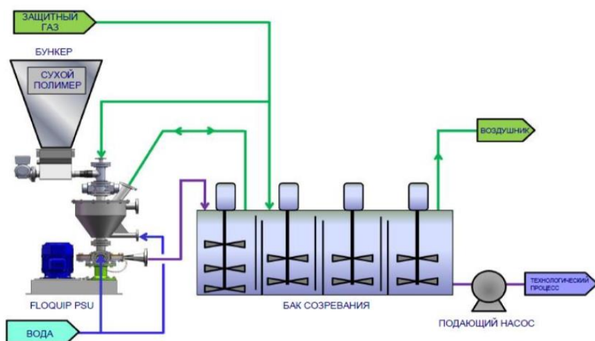
Рисунок 15 – Схема установки для растворения порошка полимера
