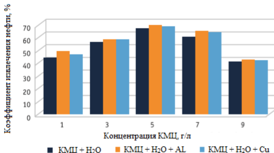
Рисунок 3 – Влияние концентрации карбоксиметилцеллюлозы на коэффициент извлечения нефти
