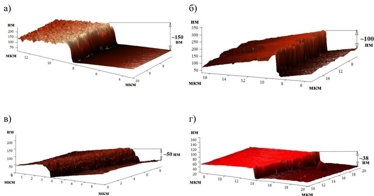
Рисунок 1 а), б), в), г) – 3D-профили сформированных на SiO 2 -подложках углеродных пленок после отжига при температурах от 650 °C, 700 °C, 750 °C и 800 °C соответственно
