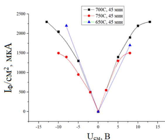
Рисунок 4 – Зависимости I_{\Phi}(U_{см}) от T отжига в пленках, сформированных на подложках: а) SiO 2 , б) Si
