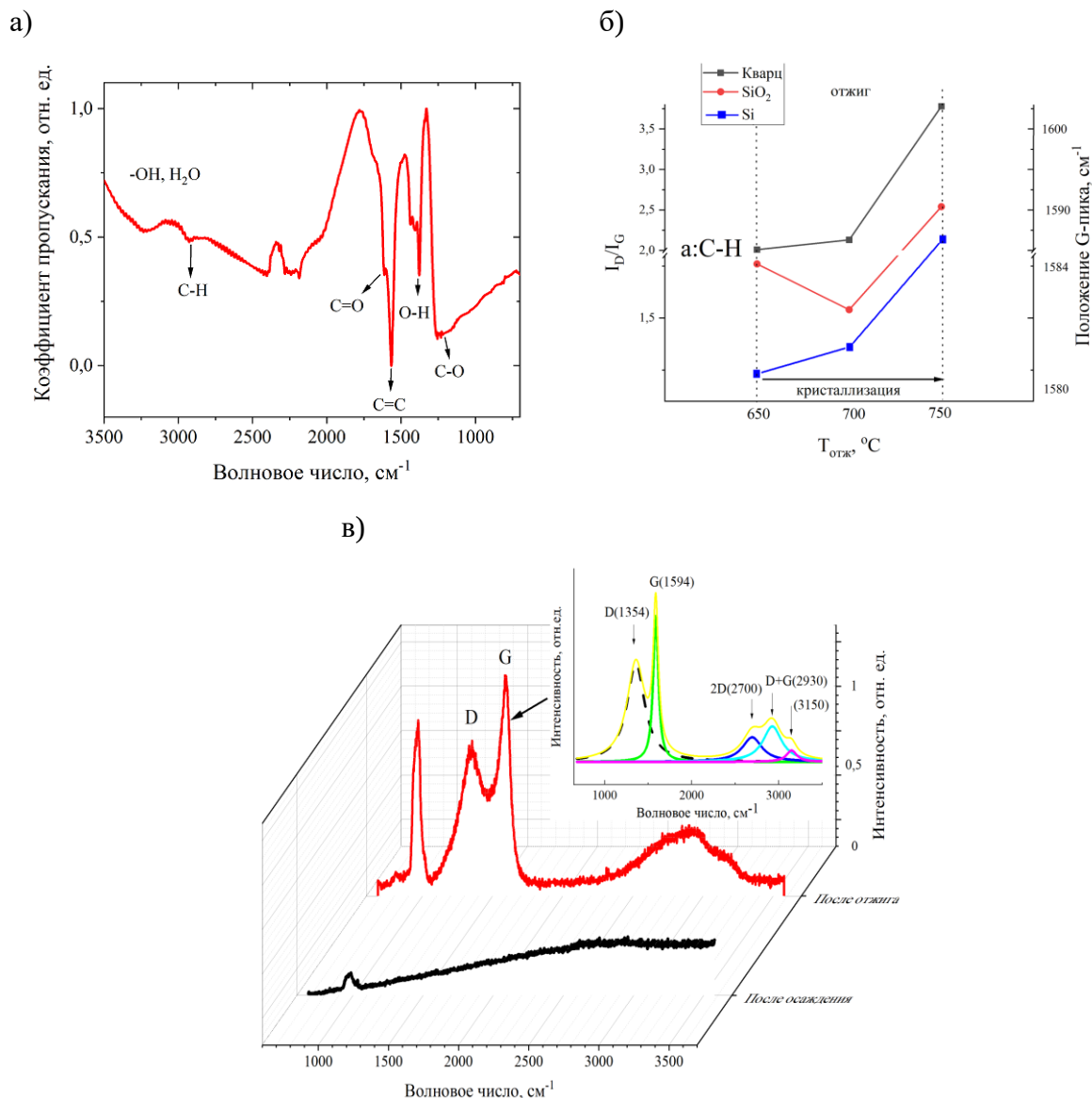
Рисунок 3 – а) Зависимость коэффициента пропускания от волнового числа в углеродных пленках, осажденных в плазме метана (200 Вт, 9 мин) на кварцевую подложку; б) зависимость отношений интегральных интенсивностей основных пиков I_D/I_G углеродных пленок от температуры отжига; в) спектры КРС углеродных пленок: после осаждения в плазме ( P = 200 Вт, 12 мин) и после отжига (650 °С, 30 мин). Во вставке: разложение сформированной углеродной пленки по лоренцианам после отжига
