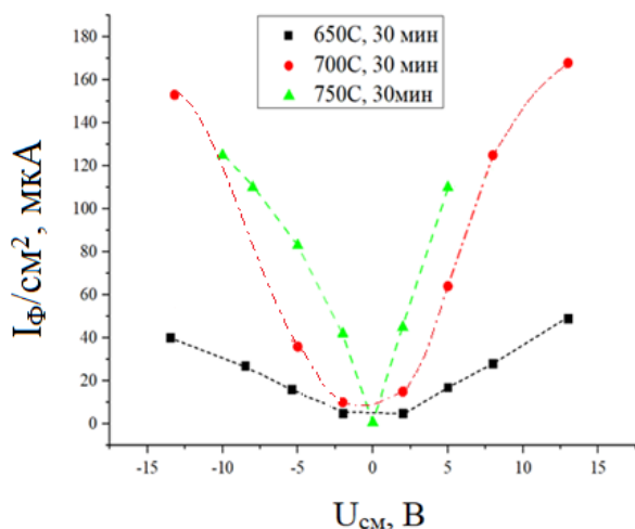
Рисунок 4 – Зависимости I_{\Phi}(U_{см}) от T отжига в пленках, сформированных на подложках: а) SiO 2 , б) Si
