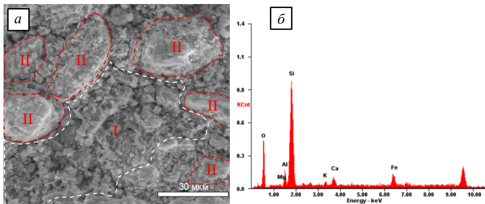
Рисунок 7 – Микрофотография (а) и элементный анализ (б) образца с содержанием глины 80 масс.% и шлака доменного 20 масс. %
