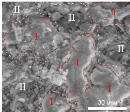
Рисунок 3 – Микрофотография структуры продукта обжига глины Верхового месторождения при 1050 °С
