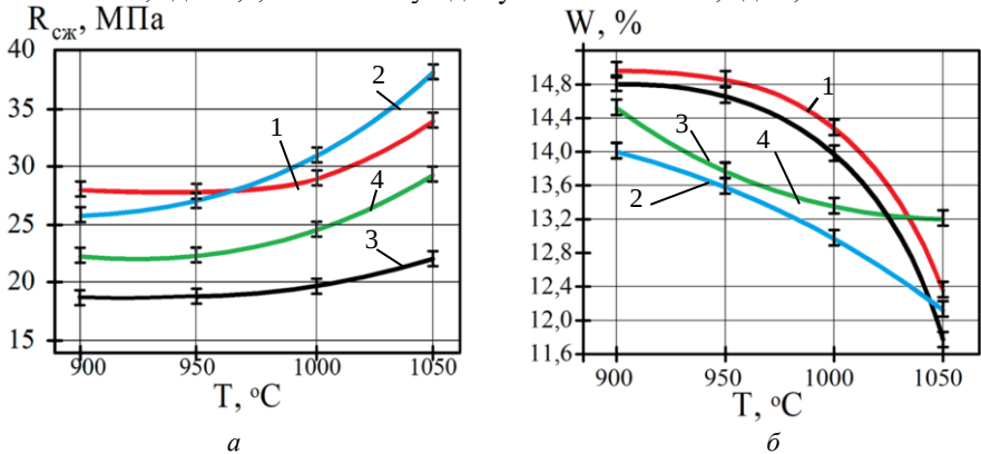
Рисунок 1 – Влияние температуры на свойства продуктов обжига шихт:
