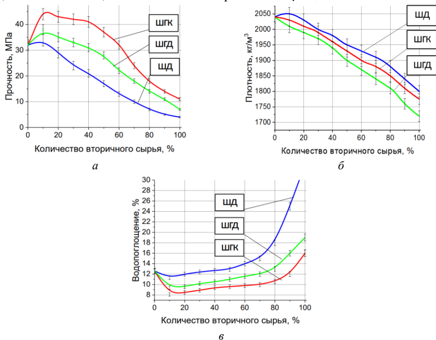
Рисунок 9 – Зависимость физико-механических свойств керамических образцов от количества вторичного сырья в компонентной шихте
