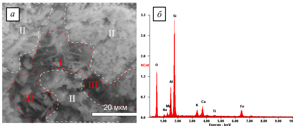
Рисунок 8 – Микрофотография (а) и элементный анализ (б) образца с содержанием глины 80 масс.% и шлама газоочистки доменного 20 масс. %
