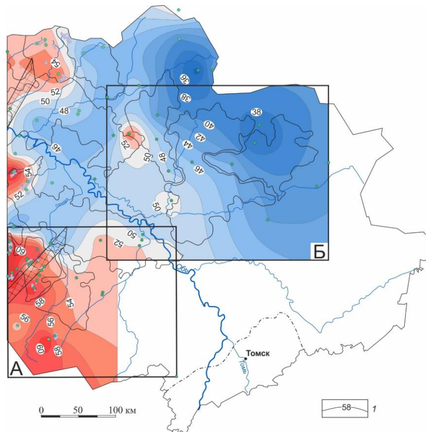
Рисунок 2 – Карта распределения плотности теплового потока восточной части Томской области на тектонической основе В. А. Конторовича (2002): 1 – изолинии теплового потока на кровле фундамента, \text{мВт/м}^2 . Остальные условные те же что на рисунке 1
