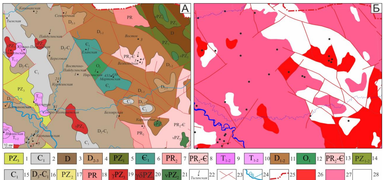
Рисунок 3 – Восточно-Пайдугинская мегавпадина. А – фрагмент геологической карты доюрского основания с дополнениями: формации с указанием возраста формирования (1-21): 1-8 – осадочные (1-4 – терригенные, 5-6 – терригенно-карбонатные, 7 – карбонатная, 8 – доломитовая); 9-14 – эффузивно-осадочные (9-10 – базальтовая, 11 – андезитово-базальтовая, 12-14 – эффузивно-карбонатные); 15-18 – метаморфические (15-16 – аспидные, 17-18 – глинисто-кремнистые); 19-21 – магматические (19-20 – гранитоиды, 21 – базиты); 22 – скважина, вскрывшая палеозойские отложения, её номер, площадь бурения; 23 – разрывные нарушения; 24 – речная сеть; 25 – административная граница Томской области; Б – схема распределения групп петротипов палеозойского фундамента по потенциалу формирования коллекторов в верхних горизонтах палеозоя (областей весовых коэффициентов 0, 1 и 2): 26 - первая группа петротипов; 27 – вторая группа петротипов; 28 – третья группа петротипов
