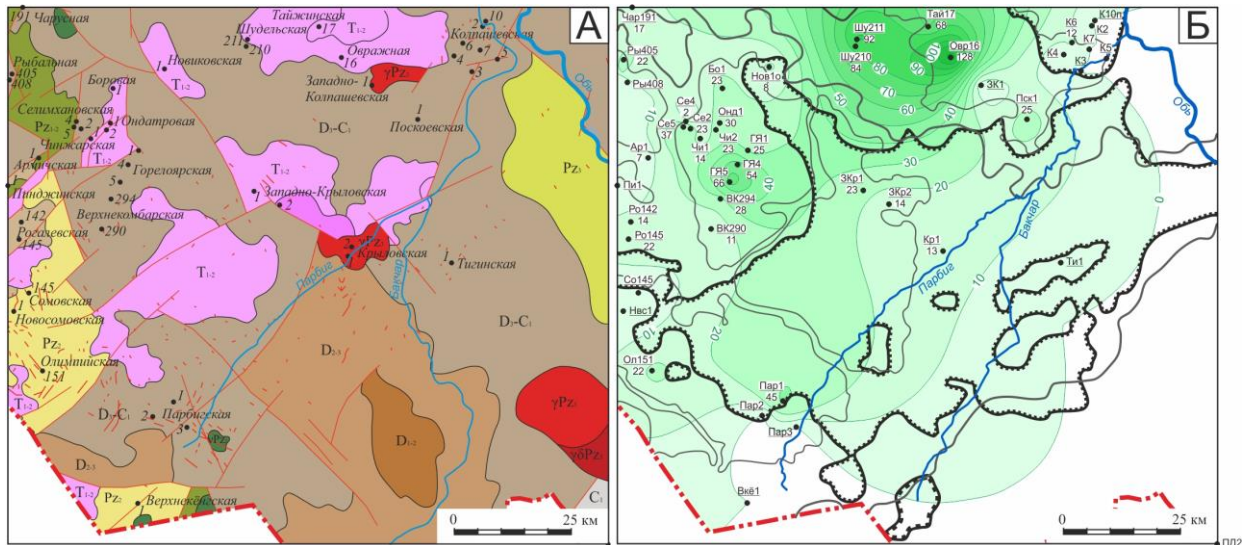
Рисунок 7 – Бакчарская мезовпадина. А – фрагмент геологической карты доюрского основания с дополнениями: формации с указанием возраста формирования. Б – схема изопакхит коры выветривания. Остальные условные те же, что на рисунках 4 и 5
