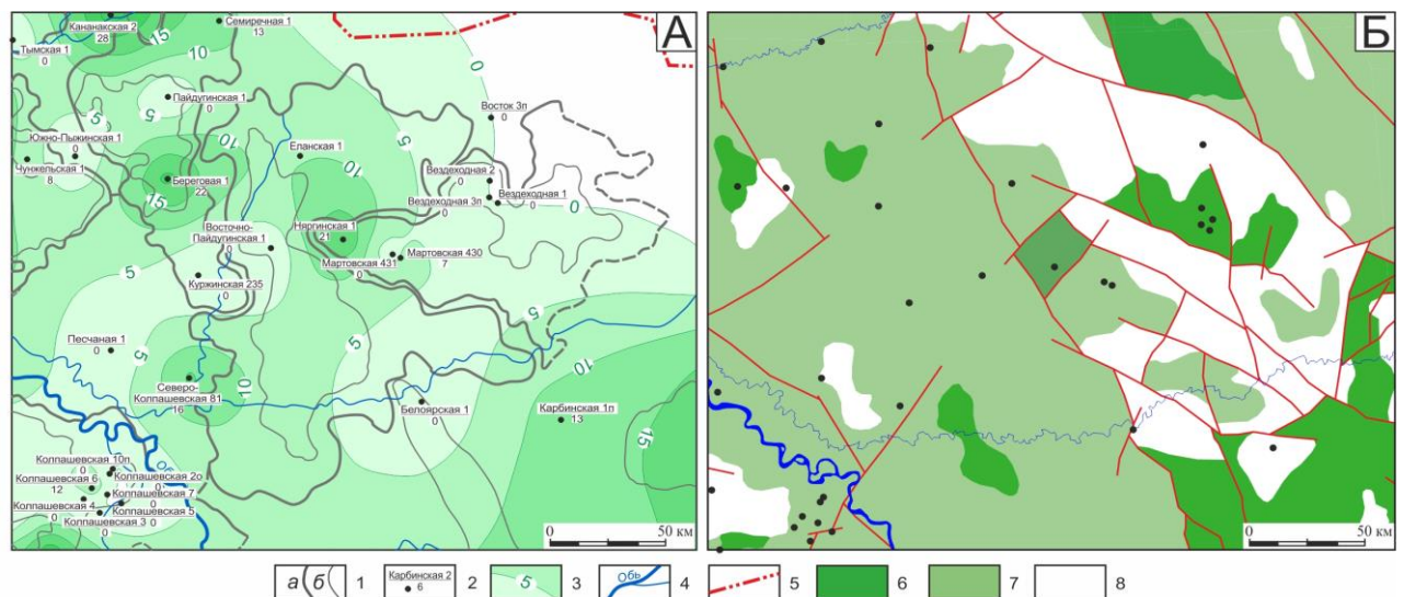
Рисунок 4 – Восточно-Пайдугинская мегавпадина. А – схема изопакит коры выветривания: 1 – границы тектонических структур I-го (а) и II-го (б) порядка; 2 – скважина (в числителе – площадь, номер; в знаменателе – мощность коры выветривания, м); 3 – изопакита, сечение 5 м; 4 – гидросеть; 5 – административная граница Томской области; Б – схема распределения групп петротипов палеозойского фундамента по потенциалу формирования коллекторов в коре выветривания (областей весовых коэффициентов 0, 1 и 2): 6 - первая группа петротипов; 7 – вторая группа петротипов; 8 – третья группа петротипов
