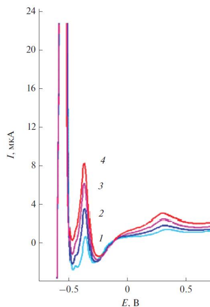
Рисунок 2 – Анодные вольтамперные кривые электроокисления бинарной системы свинец–платина
