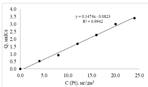
Рисунок 5 – Зависимость площади под пиком селективного электроокисления Pb из ИМС от концентрации ионов Pt (IV), C_{Pb(II)} = 25 \text{ мг/дм}^3
