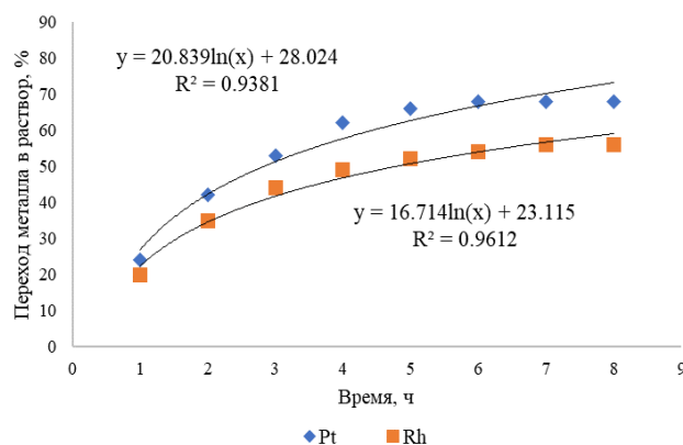
Рисунок 9 – Кинетика растворения сплава №1
