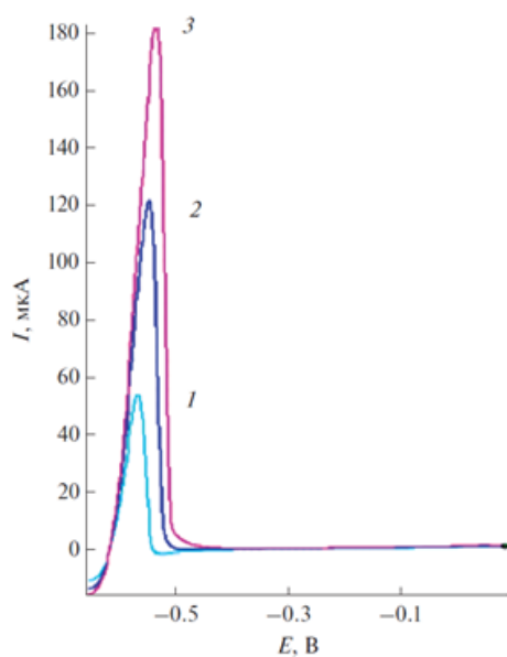
Рисунок 1 – Анодные вольтамперные кривые электроокисления свинца
