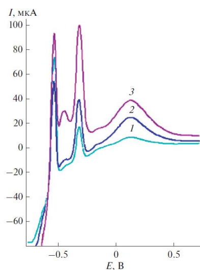
Рисунок 7 – Вольтамперные кривые электроокисления осадка свинец-платина-родий (кривая 1 – 60 \text{ мг/дм}^3 \text{ Pb (II)} + 0,5 \text{ мг/дм}^3 \text{ Pt (IV)} ; кривая 2 – 60 \text{ мг/дм}^3 \text{ Pb (II)} + 1,0 \text{ мг/дм}^3 \text{ Pt (IV)} ; кривая 3 – 60 \text{ мг/дм}^3 \text{ Pb (II)} + 1,0 \text{ мг/дм}^3 \text{ Pt (IV)} + 1,0 \text{ мг/дм}^3 \text{ Rh (III)} )
