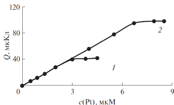
Рисунок 4 – Зависимость площади под анодным пиком при потенциале -0,3 В в системе Pt-Pb от концентрации ионов Pt (IV) при концентрациях ионов Pb (II) в растворе
