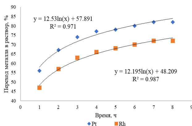
Рисунок 13 – Кинетика растворения сплава №3
