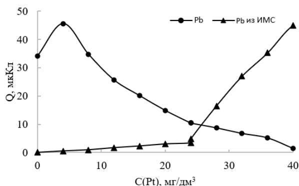
Рисунок 3 – Зависимость площади пиков электроокисления Pb и пика селективного электроокисления Pb из ИМС от концентрации ионов Pt (IV) при C_{Pb(II)} = 25 \text{ мг/дм}^3
