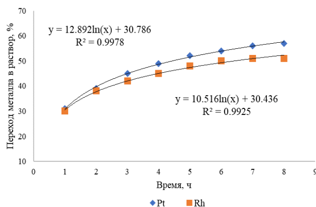
Рисунок 11 – Кинетика растворения сплава №2
