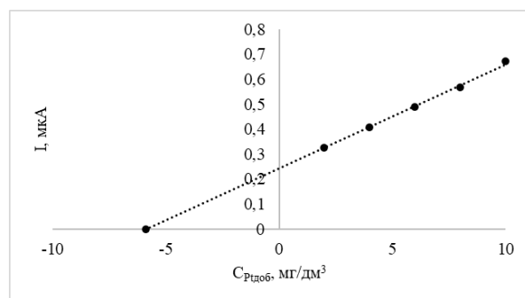
Рисунок 6 – Графическое отображения метода добавок для определения ионов Pt (IV)
