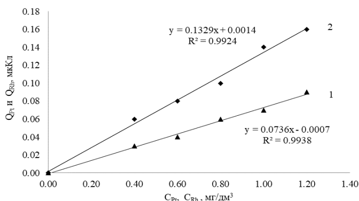
Рисунок 8 – Градуировочные прямые для определения платины (1) и родия (2) методом инверсионной вольтамперометрии по пику селективного электроокисления свинца из ИМС
