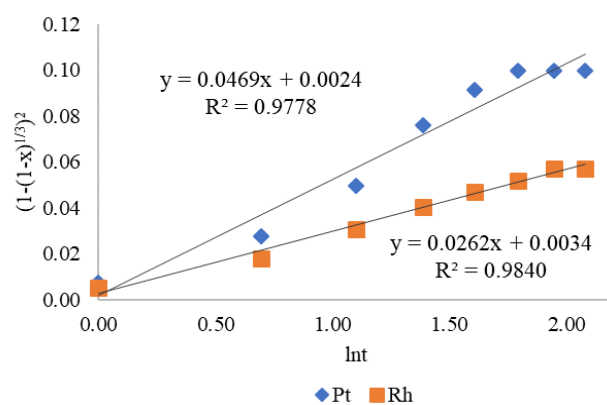
Рисунок 10 - График зависимости параметра кинетического уравнения от времени растворения сплава №1
