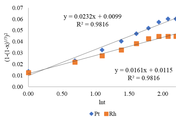
Рисунок 12 - График зависимости параметра кинетического уравнения от времени растворения сплава №2
