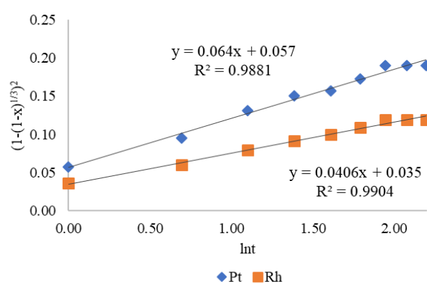
Рисунок 14 - График зависимости параметра кинетического уравнения от времени растворения сплава №3
