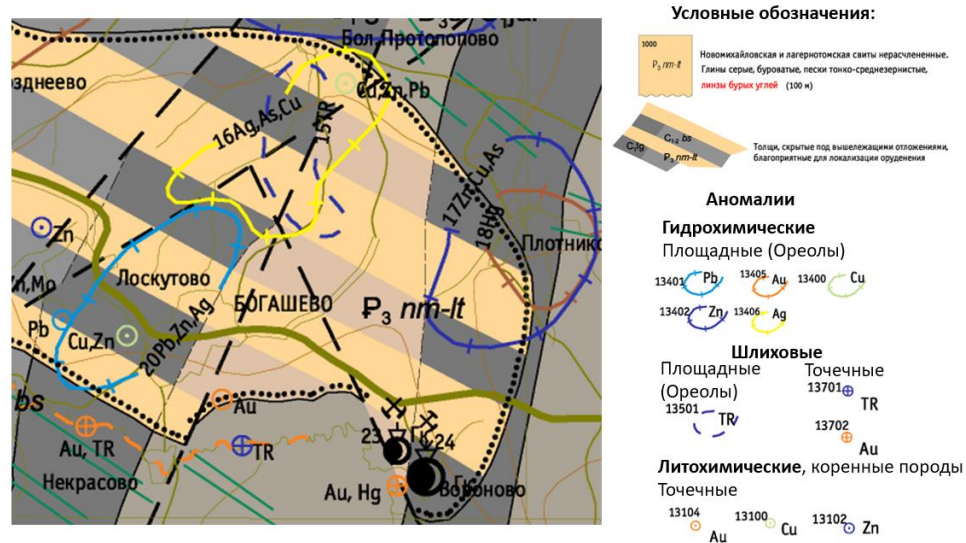
Рисунок 3.2 Фрагмент государственной геологической карты Российской Федерации, масштаба 1:200 000, Кузбасская серия, Карта полезных ископаемых и закономерностей их размещения (О-45-XXXII (Тайга)) (Черникова и др., 2007)
