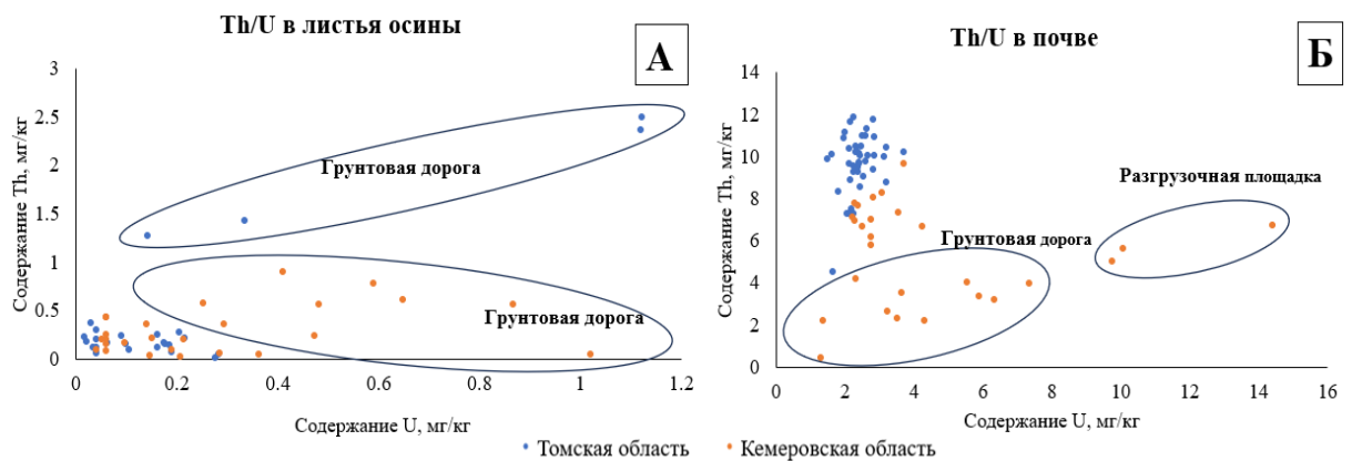
Рисунок 4.2 Распределение проб листьев осины и почвы в полях отношения Th и U
