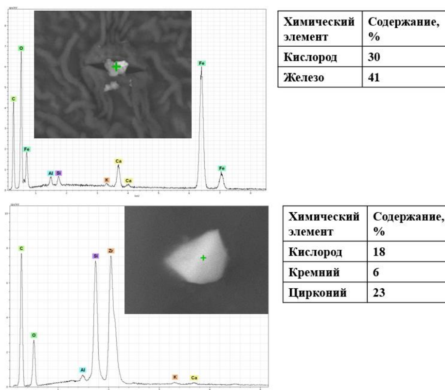
Рисунок 4.16 Частицы оксида железа и циркона на поверхности листа осины
