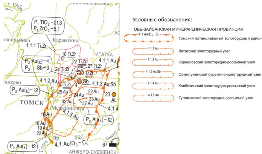
Рисунок 3.3 Фрагмент государственной геологической карты Российской Федерации. Третье поколение. Серия Западно-Сибирская. Лист О-45 – Томск. Схема прогноза полезных ископаемых масштаба 1:2 500 000 (ВСЕГЕИ, 2021)
