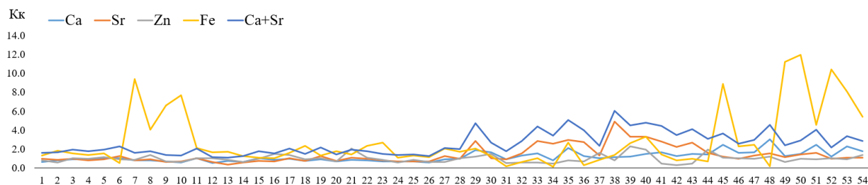
Рисунок 4.9 Графики изменчивости биогеохимических и литохимических параметров
