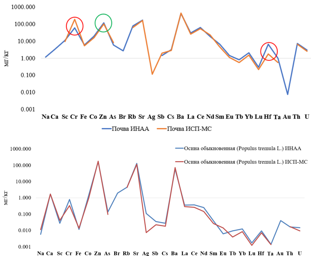
Рисунок 2.4 Сопоставление результатов ИНАА и ИСП-МС
