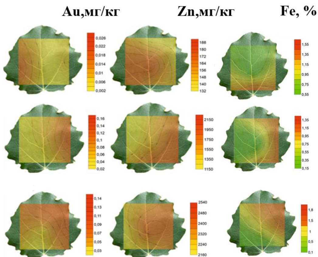
Рисунок 3.19 Карты распределения Au, Zn и Fe в листовой пластике осины по данным ИНАА
