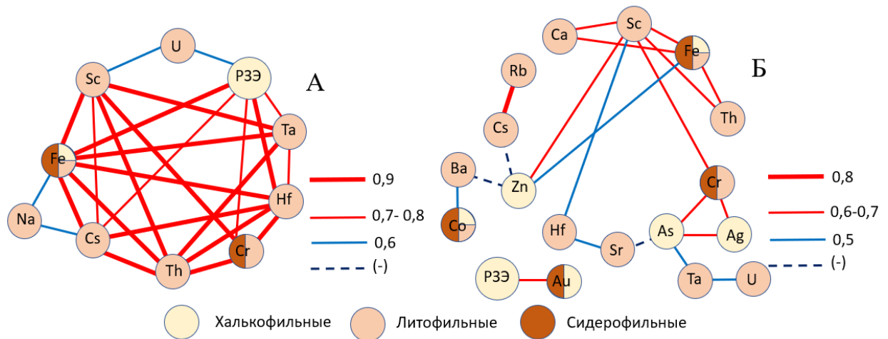
Рисунок 4.7 Корреляционные взаимосвязи химических элементов в составе золы листьев осины: А) Томская область; Б) Кемеровская область
