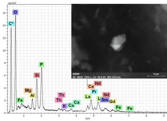
Рисунок 5.10 Частицы на поверхности листа осины и его энергодисперсионный спектр: А- монацит (н.п. Пчелка, ТО); Б- редкоземельный карбонат (н.п. Таштагол)
