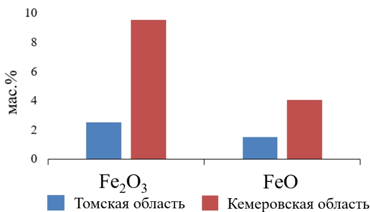
Рисунок 4.15 Содержания FeO выполнено методом титриметрии (ДВГИ ДВО РАН, 2023)
