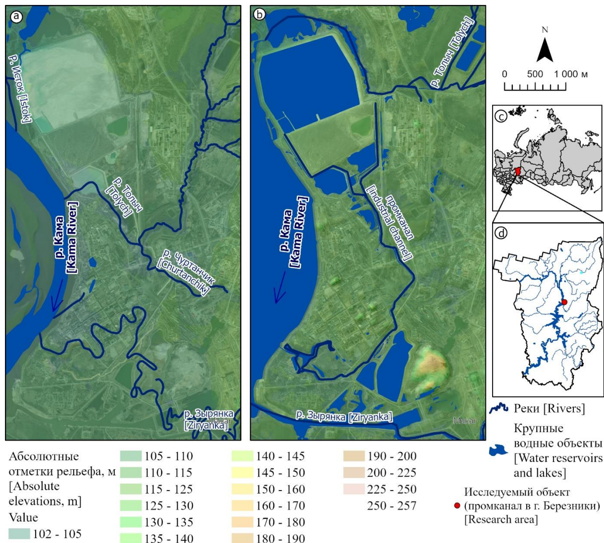
Рис. 1. Структура гидросети изучаемой территории до (а) и после (б) заполнения Камского водохранилища; с, d – обзорная карта расположения изучаемого объекта
