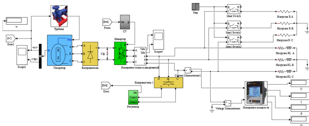
Рис. 4. Имитационная модель системы электроснабжения с инверторной микроГЭС
