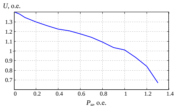
Рис. 6. Зависимость действующего значения напряжения гидрогенератора от активной мощности нагрузки
