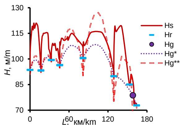
Рис. 5. Профиль АР–ОР и уровни подземных вод в настоящее время и в период начального заболачивания: H_s – поверхность водосбора или дна рек; H_r – среднедолгосрочный уровень речных и озерных (озеро у с. Мельниково) вод; H_g – среднесреднегодный уровень воды в скважине 63р в с. Мельниково; H_g^* – расчетный среднегодовой уровень подземных вод в среднем за 1967–2005 гг.; H_g^{**} – расчетный уровень подземных вод при условии, что все болота низинного типа с глубиной не более 0,3 м, а их площадь в 2 раза меньше, чем в настоящее время (ориентировочно 4 тыс. лет назад)
