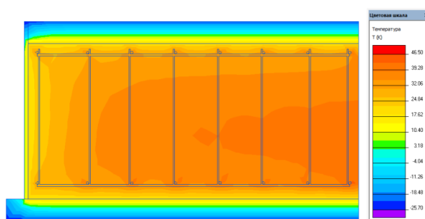
Рис. 4. Распределение температур после 46 часов прогрева при t_{н.в.} = -5\text{ }^{\circ}\text{C} ; t_{б} = 10\text{ }^{\circ}\text{C}
