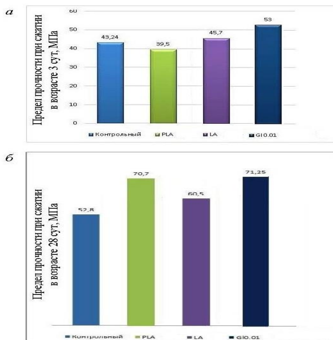
Рис.1 Прочностные показатели цементного камня с комплексными модификаторами
