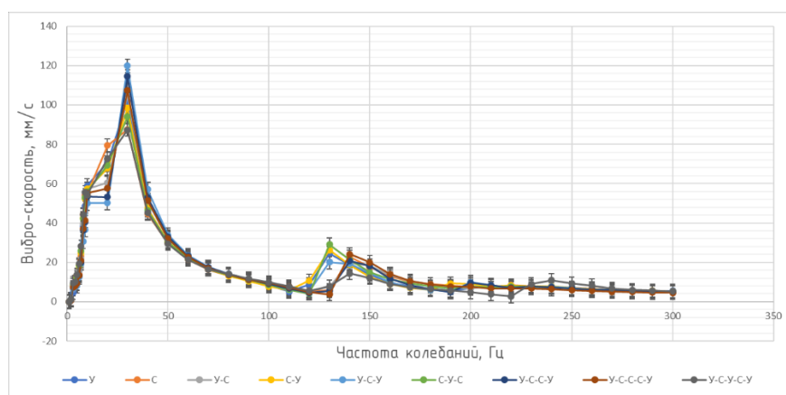
Рис. 3. График зависимости виброскорости от частоты колебаний вибродинамика
