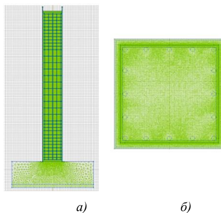
Рис. 1. Расчетная модель колонны в ПК «ELCUT PRO 6.3» с построением сетки конечных элементов а) – продольное сечение; б) – поперечное сечение
