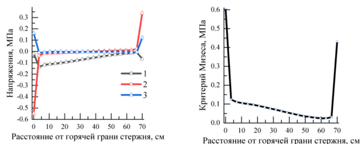
Рис. 2. Результаты моделирования твердения пескоцемента в условиях градиентов температуры: зависимости напряжений \sigma_{xx} (1), \sigma_{yy} (2) и \sigma_{xy} (3) и критерия Мизеса от расстояния вдоль контура стержня
