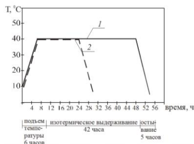
Рис. 3. Режим тепловой обработки стен и перекрытия до достижения распалубочной прочности бетона класса В20 (40 и 70 % от R_{28} ): 1 – работа газовой горелки; 2 – электрообогрев нагревательными проводами
