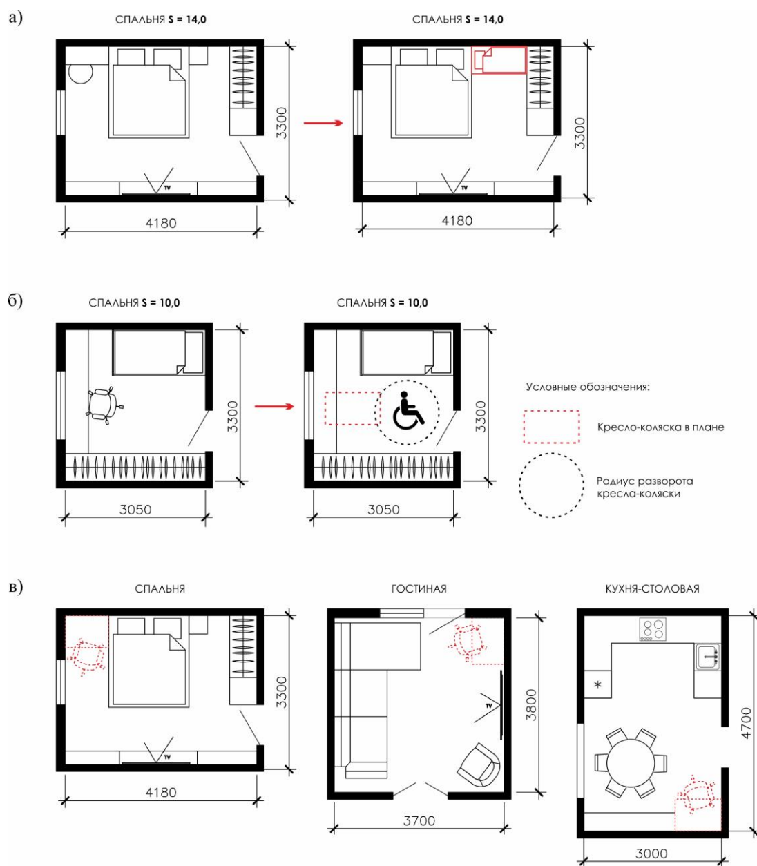
Рис. 1. Варианты адаптации жилых ячеек с учетом жизненного цикла семьи.
