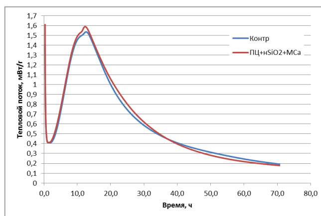
Рис. 1. Изменение теплового потока контрольного состава и состава 3
