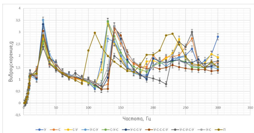
Рис. 2. График зависимости виброускорения от частоты колебаний вибродинамика
