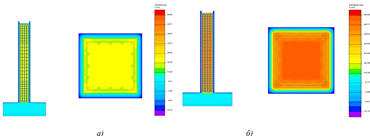
Рис. 2. Температурные поля в сечении бетонируемой колонны спустя:
