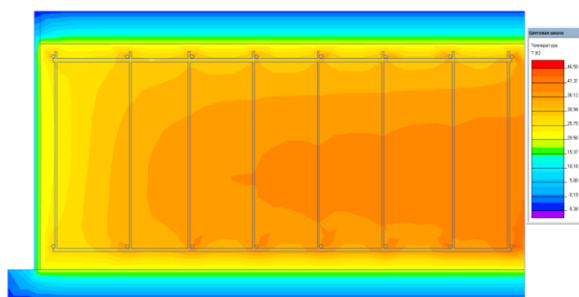
Рис. 2. Распределение температур после 46 часов прогрева при t_{н.в.} = -5 °C; t_b = 10 °C
