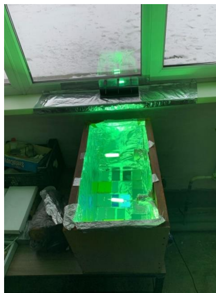
Рис. 2. Экспериментальная установка во время работы (процесса излучения)
