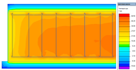
Рис. 3. Распределение температур после 46 часов прогрева при t_{н.в.} = -5 °C; t_b = 10 °C.
