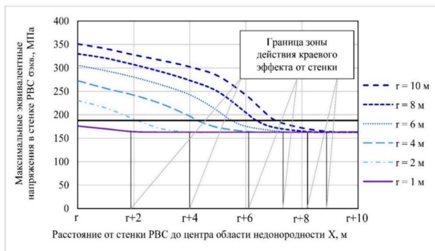
Рис. 2. Напряжения, возникающие в стенке, при максимально допустимой осадке ( \delta = 6 мм)
