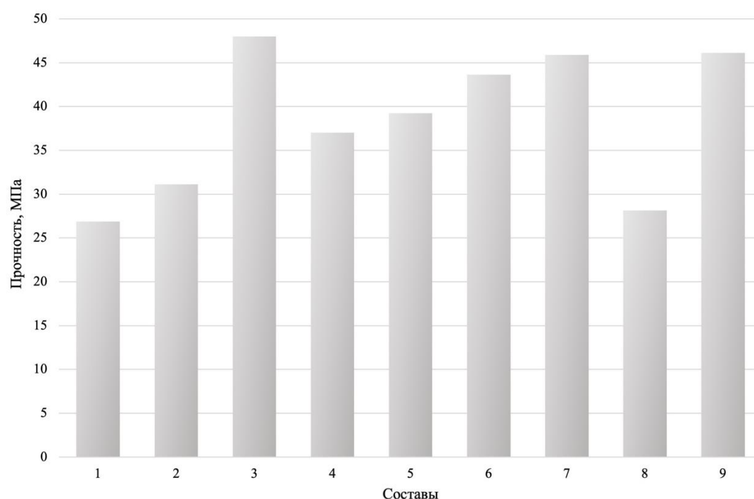
Рис. 1. Прочность бетона при сжатии в возрасте 28 суток
