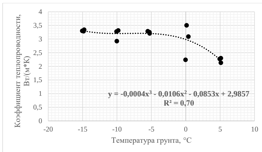
Рис. 3. Зависимость между коэффициентом теплопроводности и температурой грунта
