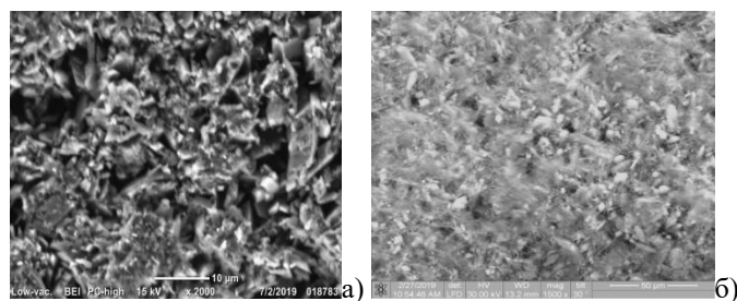
Рис. 1. Электронно-микроскопические снимки с применением фторангидрита естественной гранулометрии (а); с применением модифицированного фторангидрита (б)
