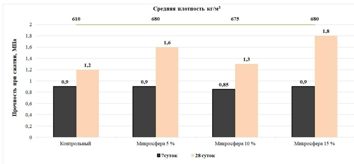
Рис. 1. Влияние микросферы на прочностные свойства газобетона
