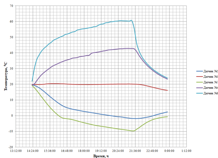
Рис. 2. Графики распределения температуры
