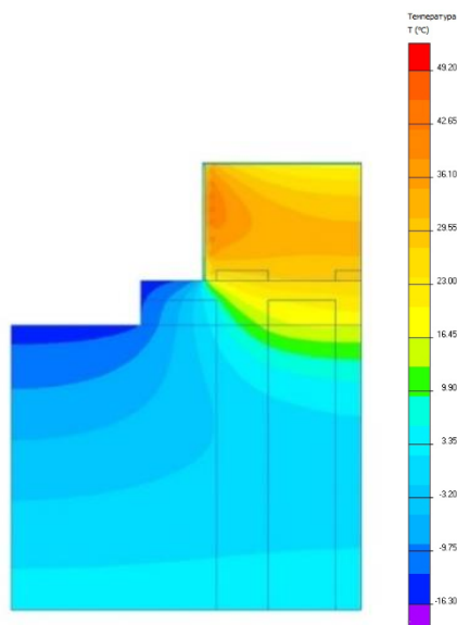
Рис. 1. Температурное поле в бетоне после 96 часов изотермического прогрева при температуре наружного воздуха -15^{\circ}\text{C} с шагом греющего провода 100 мм
