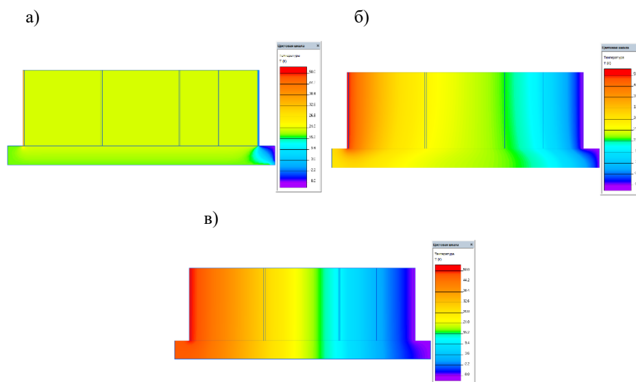
Рис. 3. Температурные поля: а) перед началом прогрева; б) после 4-х часов; в) после 7-ми часов
