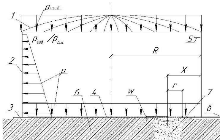
Рис. 1. Расчетная схема: 1 – крыша РВС; 2 – стенка РВС; 3 – окрайка; 4 – полотнище днища; 5 – опорное кольцо; 6 – грунтовое основание с коэффициентом постели k_2 ; 7 – зона локальной неоднородности основания с коэффициентом постели k_1 ; R – радиальный размер резервуара, м; r – радиальный размер зоны локальной неоднородности; X – расстояние от стенки до центра зоны неоднородности; \delta – толщина днища; w – осадка
