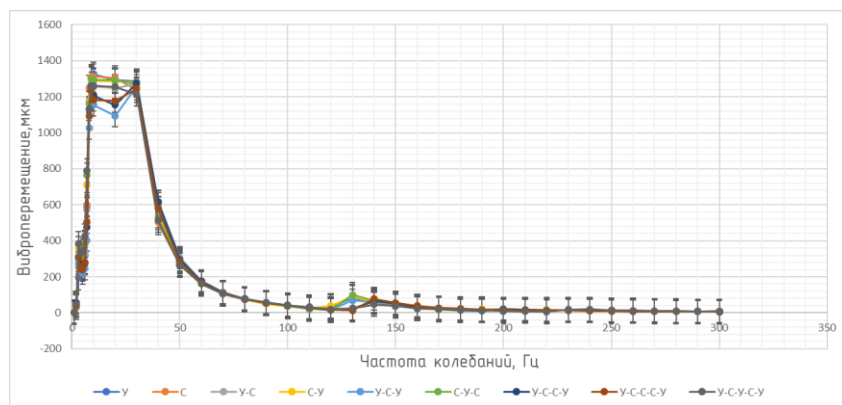
Рис. 4. График зависимости виброперемещения от частоты колебаний вибродинамика
