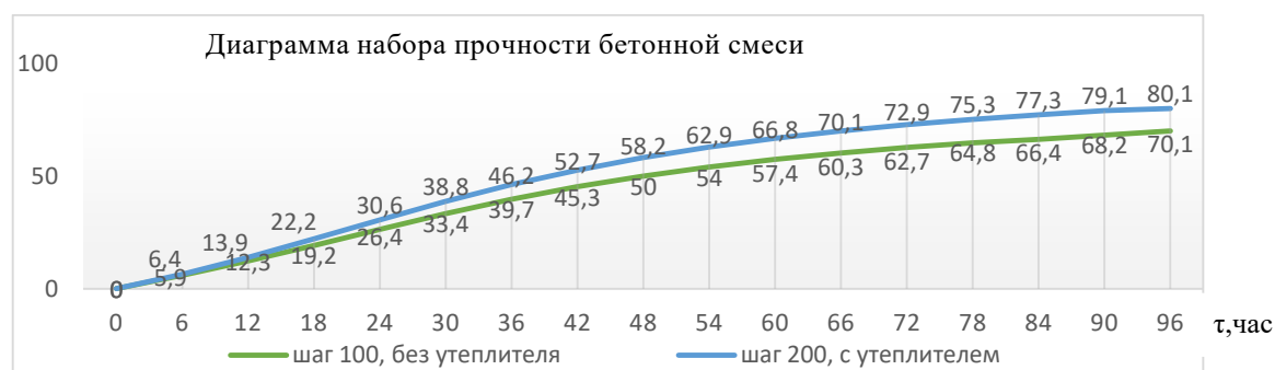
Рис. 3. Графики нарастания прочности бетона конструкции в т. 7 при разных шагах греющего провода
