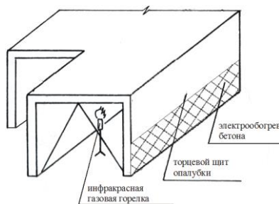
Рис. 1. Схема комплексной тепловой обработки бетона
