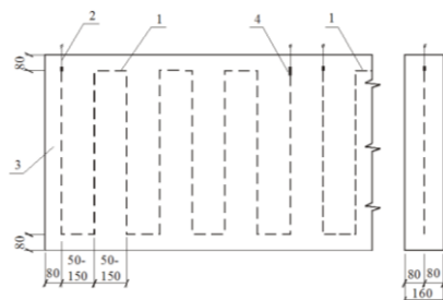
Рис. 2. Схема раскладки и подключения нагревательного провода при прогреве стен:
