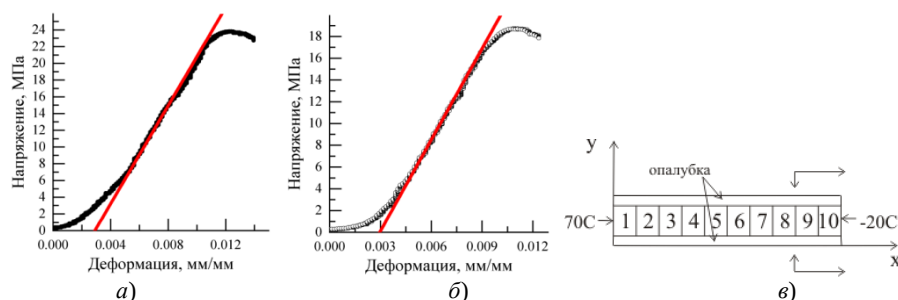
Рис.1. Кривые напряжение-деформация и схема распределения образцов в цементном стержне: а) В/Ц = 0,40, образец № 4; б) В/Ц = 0,49, образец № 4; в) схема плоского сечения твердеющего цементного стержня в условиях градиентов температуры
