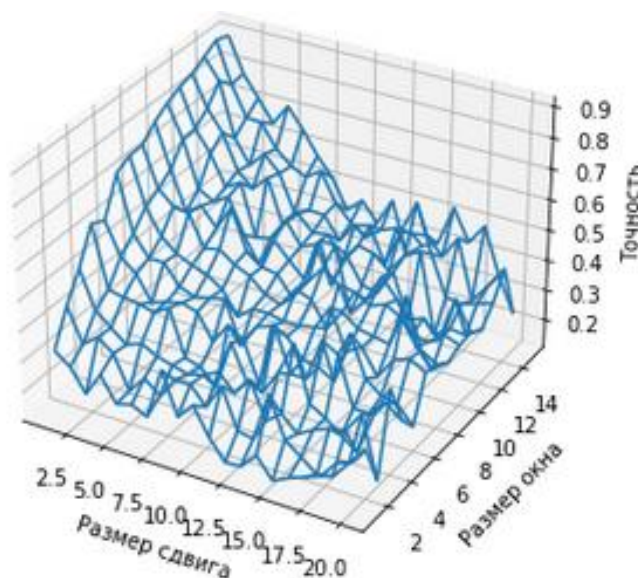
Рис. 1. Точность моделей при разных параметрах скользящего окна
