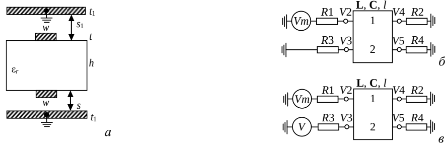
Рис 1. Поперечное сечение ПЛП с однократным МР (а), схема включения без питания на резервной цепи (б), схема включения с питанием в резервной цепи (в)
