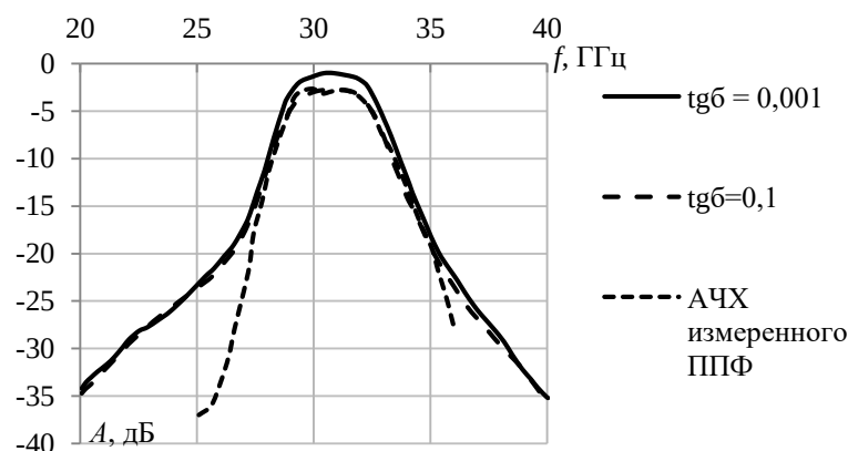
Рис. 4. График АЧХ рассчитанного ППФ на МПЛ с изменением \operatorname{tg} \delta
