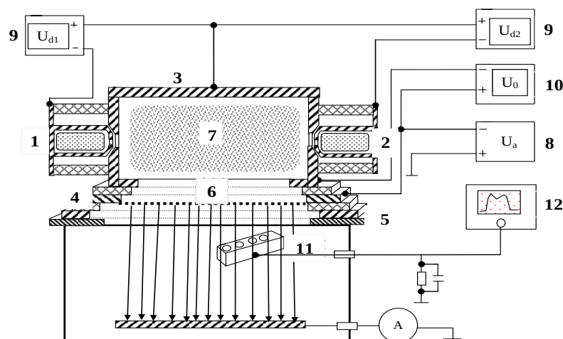
Рис. 1. Экспериментальная установка
