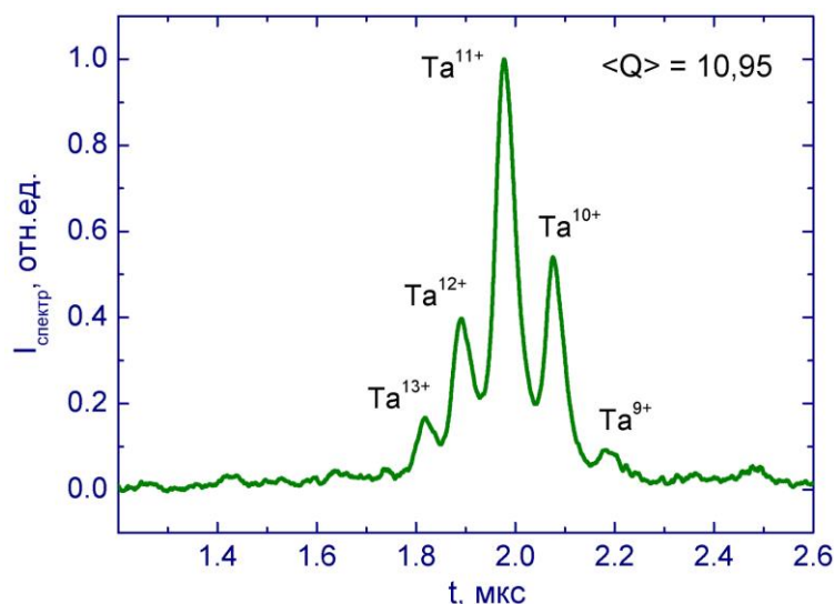
Рис. 1. Зарядовые состояния ионов тантала в ионном пучке, измеренные времяпролетным масс-спектрометром
