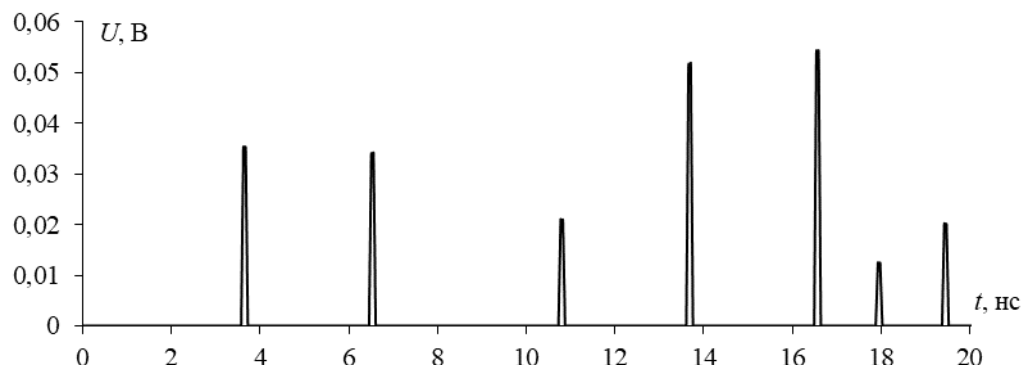
Рис. 2. Форма напряжения на выходе асимметричного МФ с лицевой связью с оптимизированными параметрами
