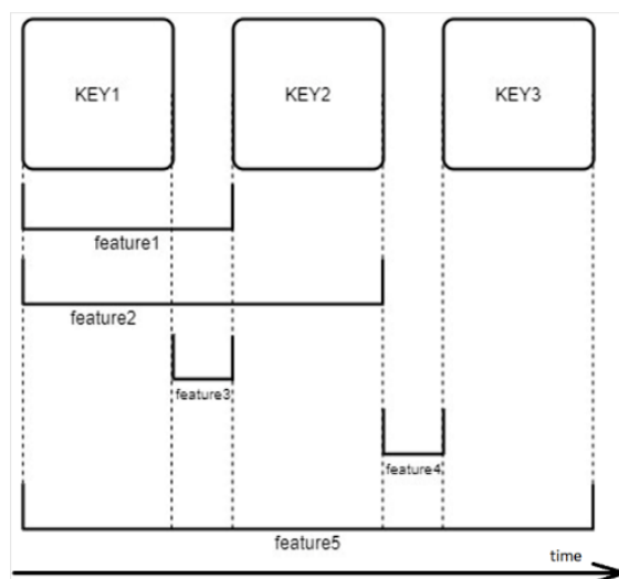
Рис. 1. Признаки, описывающие триграмму Key1-Key2-Key3
