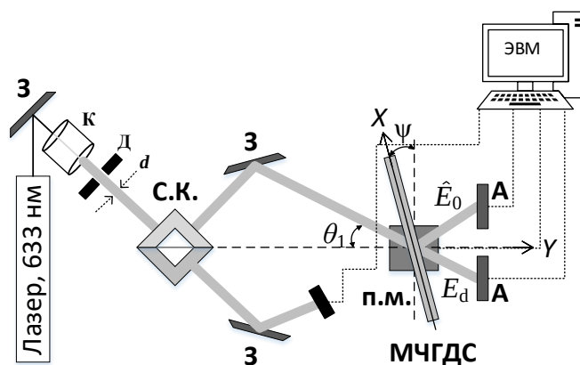
Рис. 2. Схема считывания мультиплексированной chirпированной ГДС: 3 – зеркало, С.К. – светоделительный кубик, П.М. – поворотный механизм, К – коллиматор, Ш – шторка, А – анализатор лазерных пучков, ЭВМ – электронно-вычислительная машина
