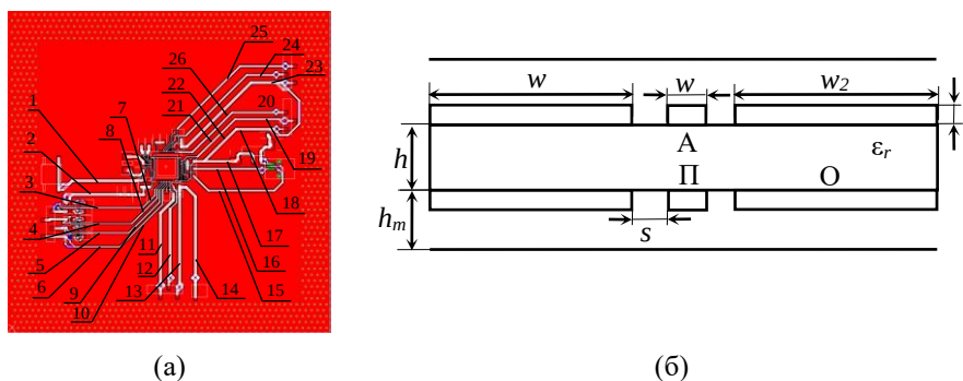
Рис. 2. Сигнальные трассы измерительной ПП с МР (а), поперечное сечение исследуемой структуры с учетом паяльной маски (б)
