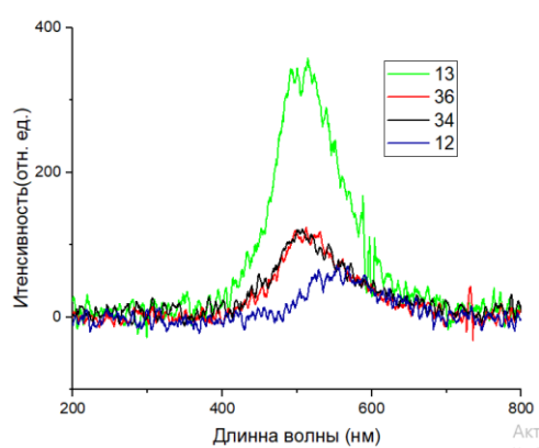
Рис. 2. Спектры электролюминесценции образцов 12, 13, 34, 36
