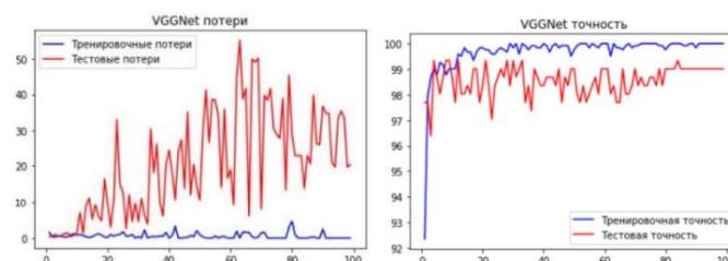
Рис. 3. Результаты VGGNet
