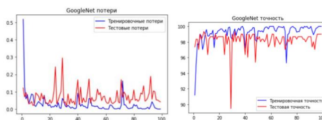
Рис. 4. Результаты GoogleNet
