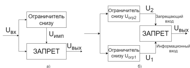
Рис. 5. Структурные схемы амплитудных селекторов: а) ограничитель сверху; б) ограничитель сверху и снизу
