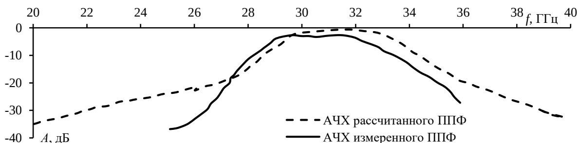
Рис. 2. АЧХ рассчитанного и измеренного МПЛ ППФ
