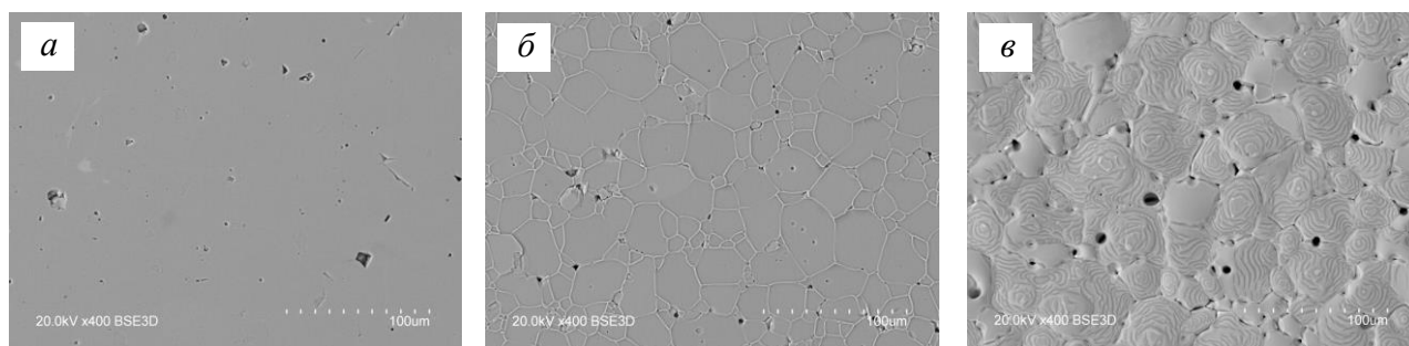
Рис. 3. Поверхность керамики ВК-100 : а – исходный образец; б – после обработки при температуре 1300 °С; в – после обработки при температуре 1500 °С
