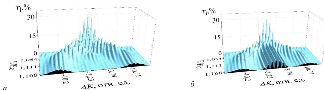
Рис. 1. Зависимость ДЭ двухслойной ГДС при (а) \theta_{\text{п}} = 0^\circ и (б) \theta_{\text{п}} = 30^\circ
