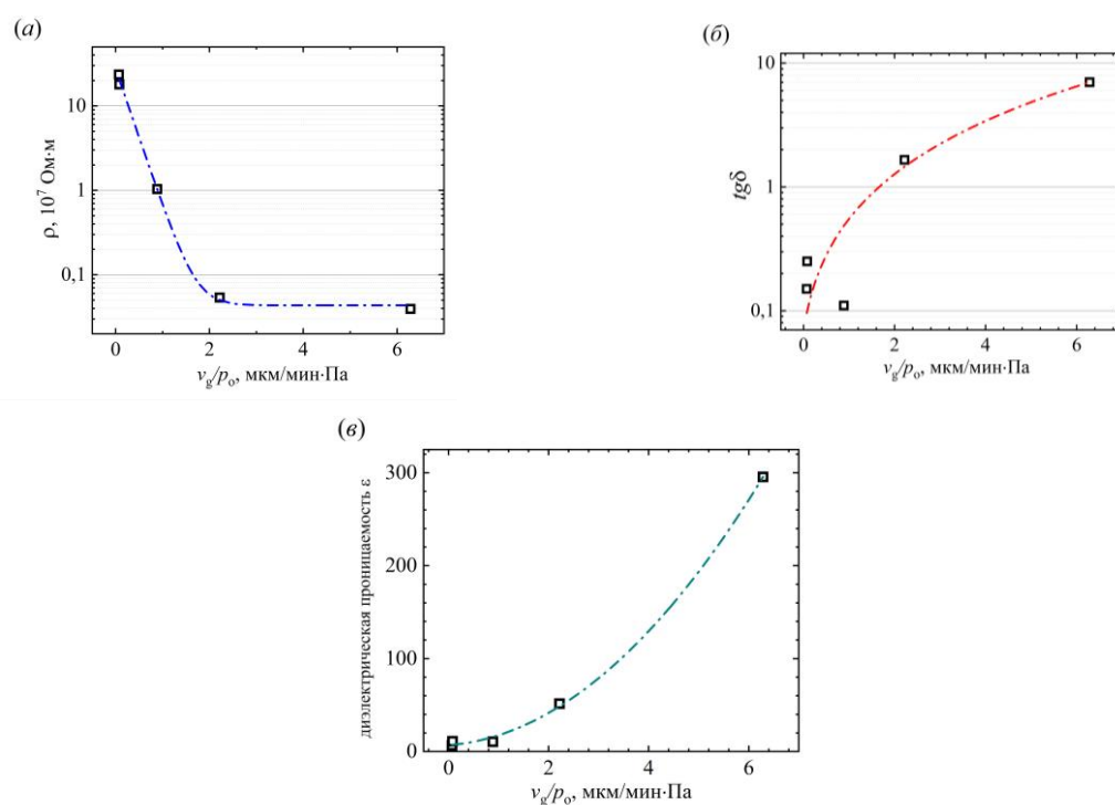
Рис. 2. Удельное сопротивление \rho (а), тангенс \operatorname{tg}\delta угла потерь (б) и диэлектрическая проницаемость \epsilon пленок (в) как функция параметра v_g/p_o
