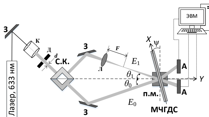
Рис. 1. Схема формирования мультиплексированной chirпированной ГДС: 3 – зеркало Л – линза, С.К. – светоделительный кубик, П.М. – поворотный механизм, К – коллиматор, А – анализатор лазерных пучков, ЭВМ – электронно-вычислительная машина
