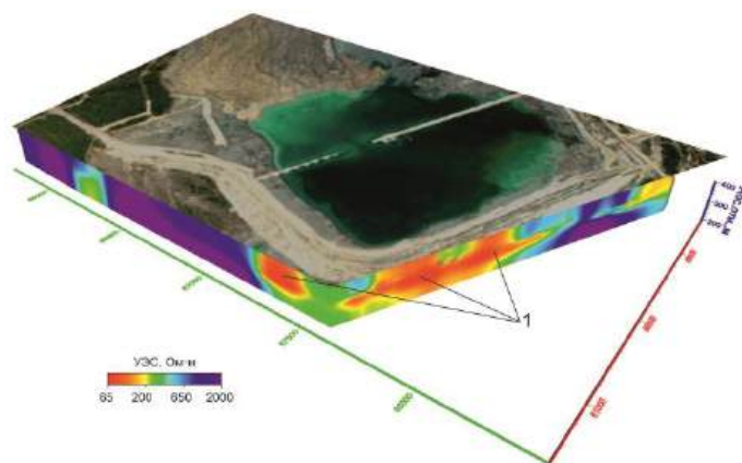
Рис. 2. Модель распределения УЭС. 1 – аномалии низкого УЭС, связанные с обводнёнными грунтами.
