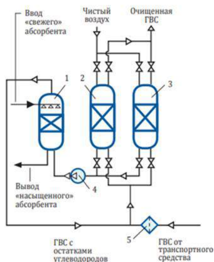
Рис. Схема адсорбционной УРП
