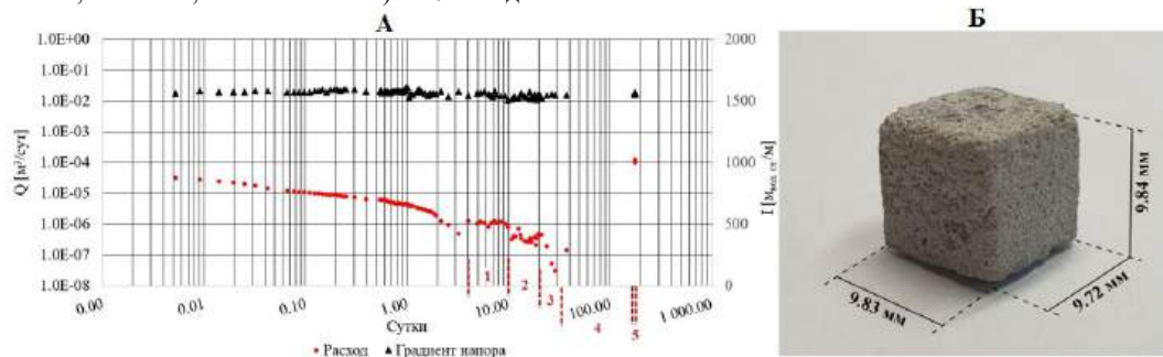
Рис. 1. Результаты фильтрации через образец № 2 (пояснения по тексту)
