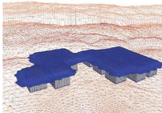
Рис. 4. Модель системы инженерных барьеров безопасности, включающей покрывающий экран, бетонные стены и основания сооружений ППЗРО
