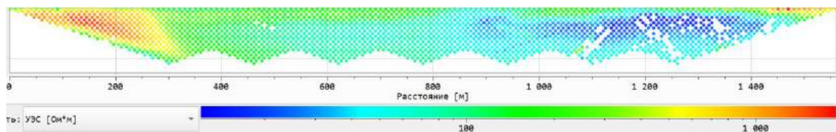
Рис. 1. Разрез кажущегося сопротивления на профиле 1 после первичной обработки.
