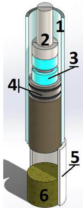
Рис. 1. Эскизный вид разработанных средств для подготовки цилиндрических образцов грунта с заданным сжатием: 1 – камера сжатия; 2 – шток; 3 – центратор; 4 – штамп; 5 – вытеснительный стакан; 6 – упругая подкладка
