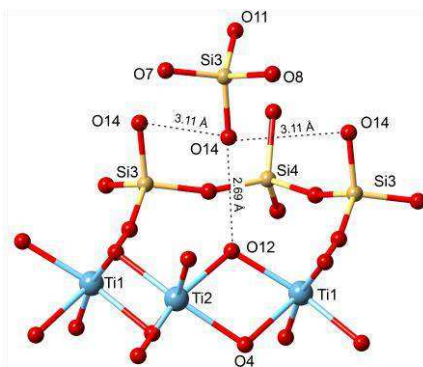
Рис. 4. Схема взаимодействия водородных связей в кристаллической структуре КЗ
