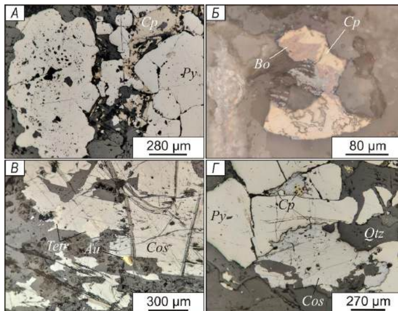
Рис. 1. Рудная минерализация. А – крупные идиоморфные кристаллы пирита в ассоциации с халькопиритом; Б – вкрапления медной минерализации (халькопирит в сростаниях с борнитом); В – крупные листоватые зерна козалита в сростании с золотом и с вкраплениями тетрадимита;
