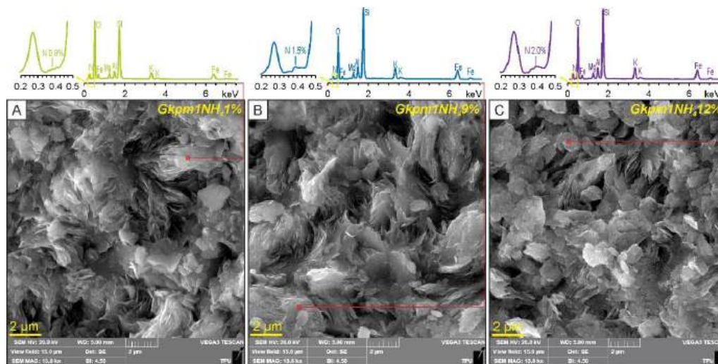
Рис. 2. СЭМ-снимки, полученные с помощью детектора вторичных электронов, демонстрирующие морфологические характеристики нанокомпозитов: (A) Gkpm1NH4 1 %, (B) Gkpm1NH4 9 % и (C) Gkpm1NH4 12 %. Спектры энергодисперсионной спектроскопии (ЭДС) представлены для минеральных микрочешуек, расположенных в ядерной части ГАН. Область анализа для каждого спектра выделена красным квадратом
