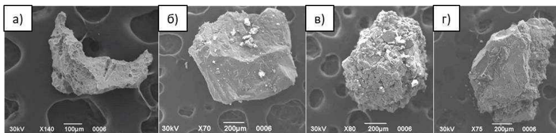
Рис. 4. Зерно пирротина (а), кристалл пирита (б), агрегат микрокристаллов (в), сросток кристаллов пирита (г)
