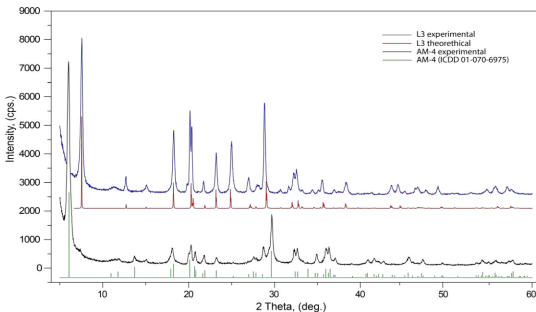
Рис. 3. Порошковые рентгеновские дифракционные картины исходных фаз AM – 4 и L3
