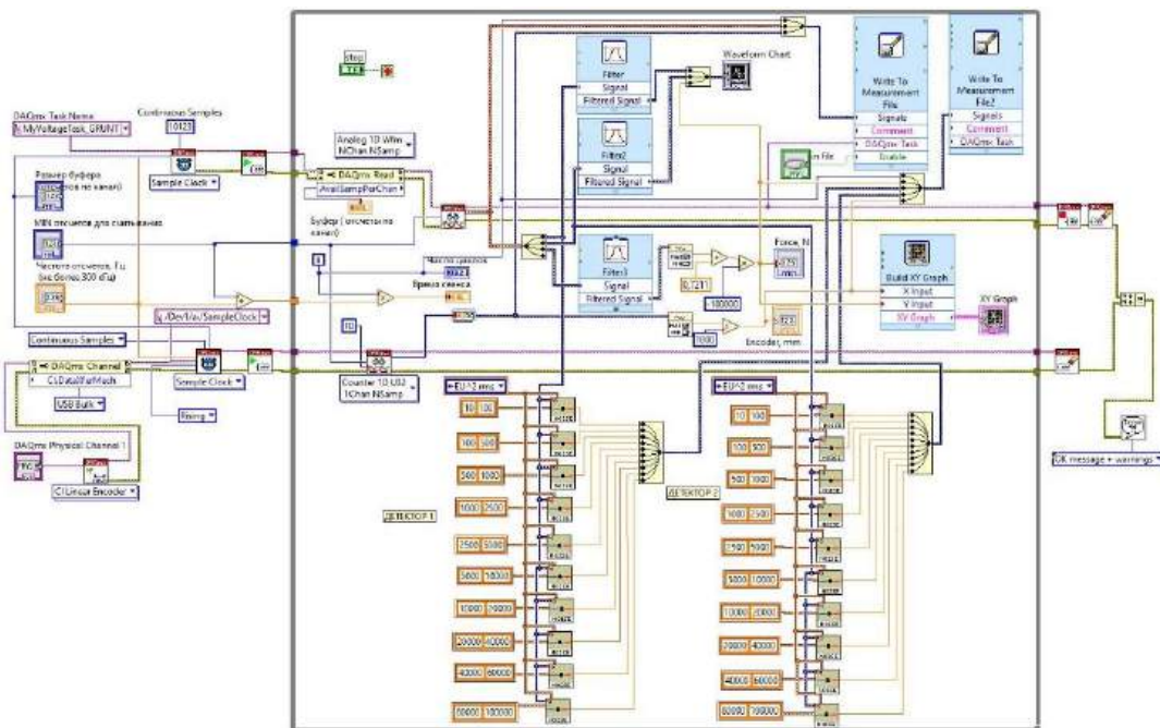
Рис. 1. G-код виртуального прибора системы регистрации сигналов дополнительного блока датчиков
