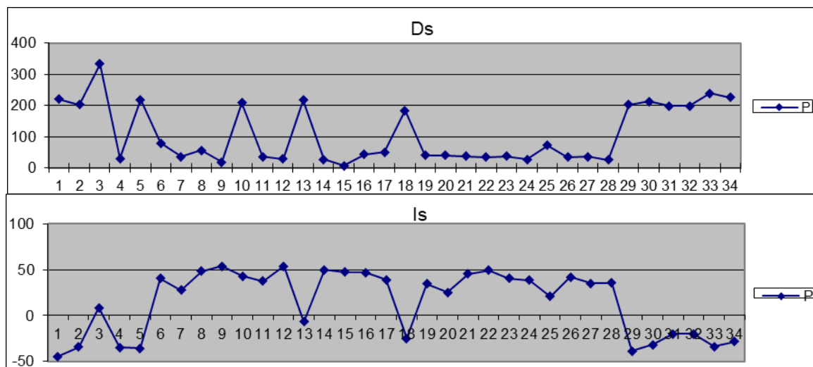
Рис. 2. Графики распределения склонения ( D_s ) и наклонения ( I_s ) в древней системе координат
