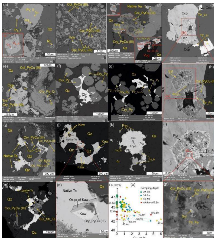
Рис. Микрофотографии (изображения SEM-BSE), демонстрирующие парагенезис сульфидов, сульфосолей и теллуридов рудной зоны Эми
