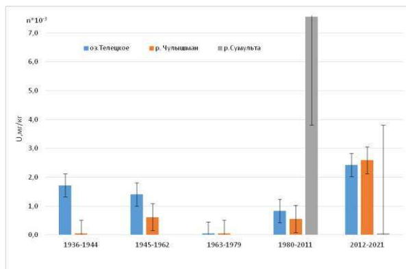
Рис. Диаграмма содержания U по периодам и точкам исследования
