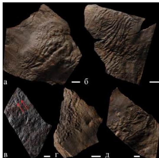
Рис. 2. Представители организмов эдиакарского типа из усть-палегской свиты рр. Мезенская Пижда и Четласс, возвышенность Четласский камень. а, б, д – Arumberia ; в – Palaeopascichnus (показаны стрелочками); г – Rameshia [5]. Длина масштабной линейки 1 см
