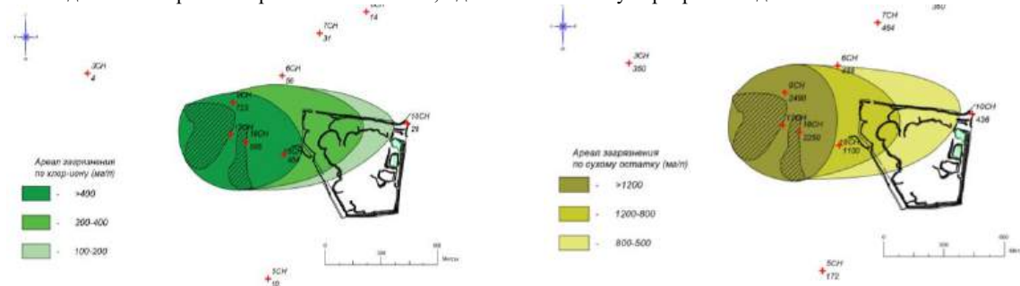
Рис. 2. Ареал загрязнения хлор-ионом слева и по сухому остатку справа вблизи Ново-Сухоложского карьера аргиллитов
