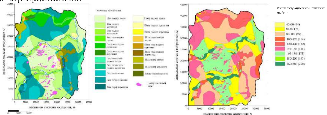
Рис. Схема районирования территории с различными условиями формирования инфильтрационного питания и карта неоднородности среднееголетнего инфильтрационного питания Пермилковского месторождения подземных вод
