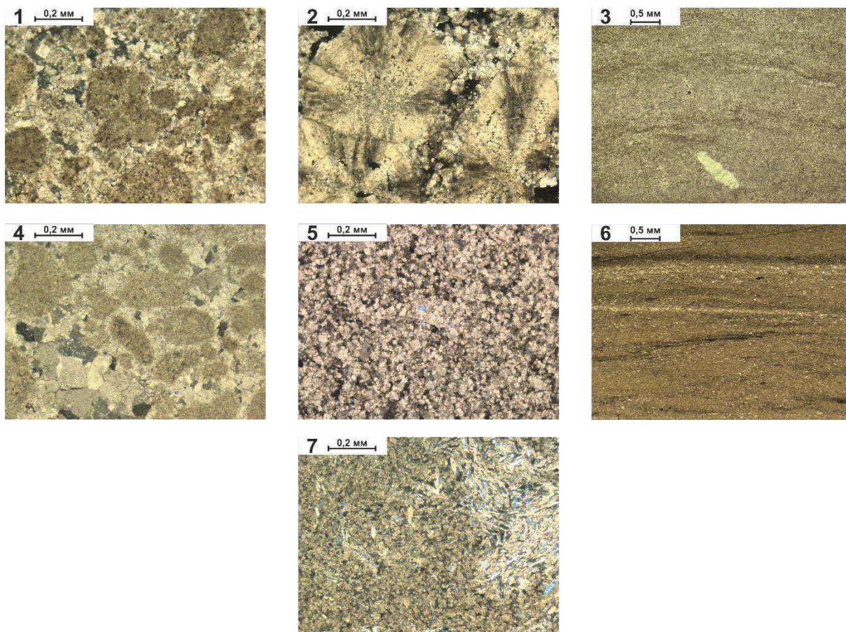
Рис. 1. Микроскопические текстурно-структурные особенности карбонатных пород юряхской свиты, никели X
