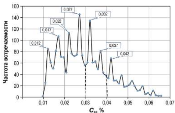
Рис. 1. Гистограмма распределения относительного содержания бора в меловых песчаных пластах углеводородных месторождений полуострова Ямал
