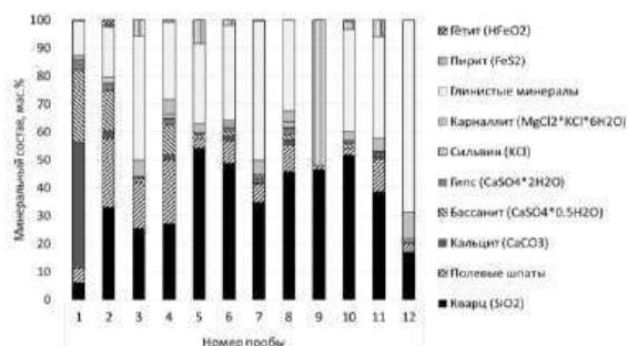
Рис. 1. Минеральный состав проб отвала Лёвихинского рудника, мас. %
