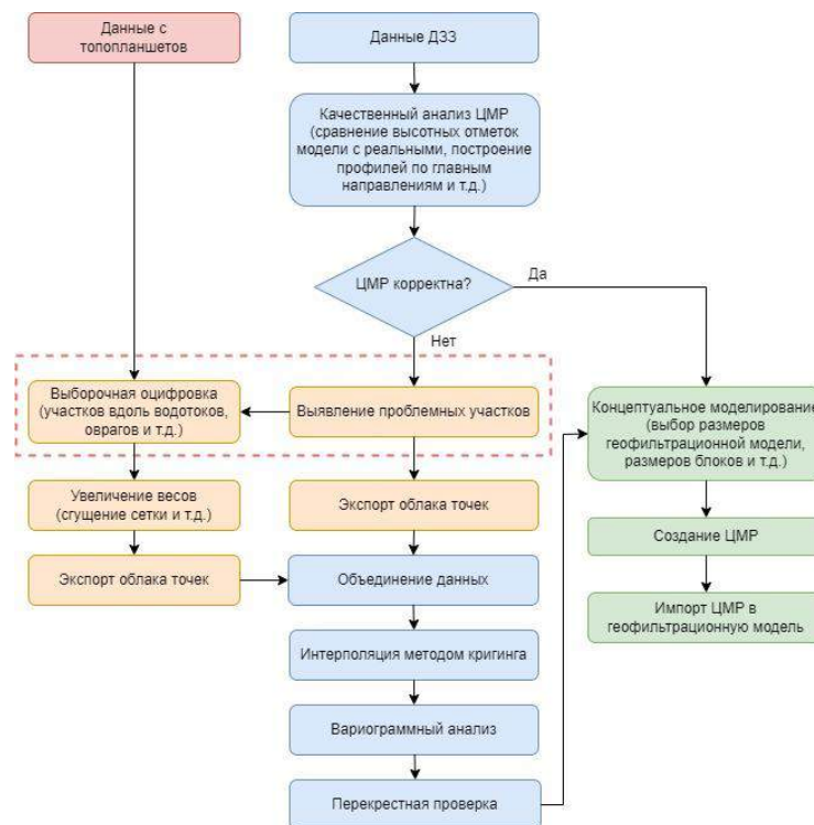
Рис. Блок-схема методики подготовки и объединения данных о поверхностях рельефа из разных источников
