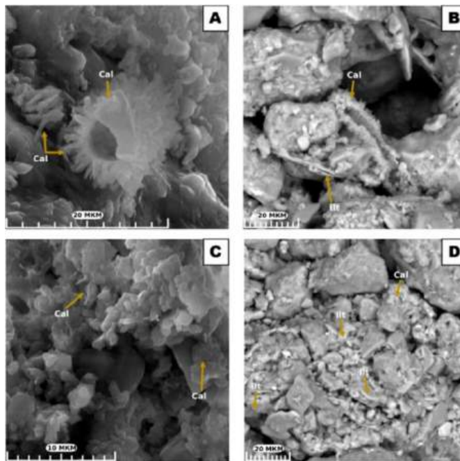
Рис. 2. Строение и состав карбонатных новообразований
