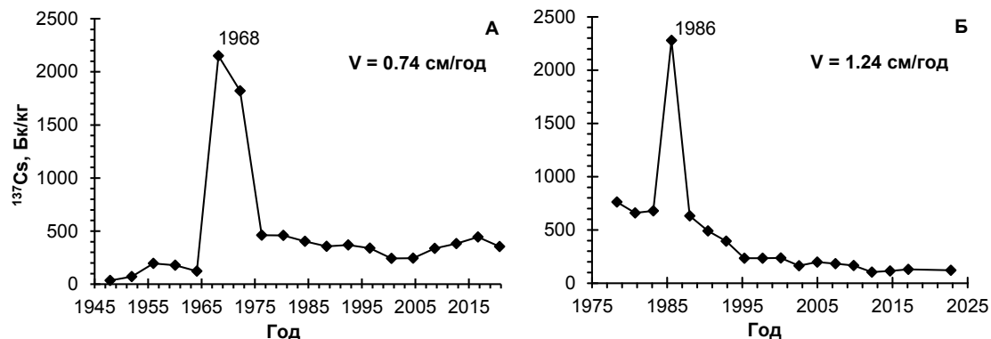
Рис. 2. Примеры хронологии поступления ^{137}\text{Cs} в донные отложения разных участков вблизи села Балчуг, относящиеся к паводку 1966 года (А) и паводку 1988 года (Б)
