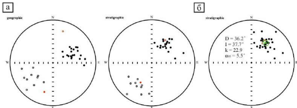
Рис. 1. а) распределение палеомагнитных направлений в географической и стратиграфической системах координат; б) осредненные палеомагнитные направления в стратиграфической системе координат
