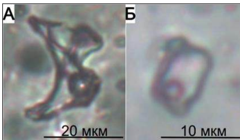
Рис. 2. Максимальный размер флюидных включений. А – двухфазное включение в пропилитах; Б – двухфазное включение в березитах
