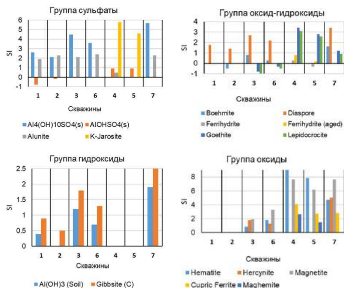
Рис. 2. Индексы насыщения воды по отношению к минералам
