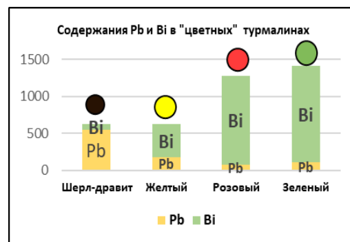
Рис. 5. Соотношение количества Pb и Bi в турмалинах жил «Иркутянка» и «Геологическая» (Малханское месторождение) (ppm, МГРИ, 2024)
