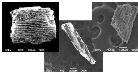
Рис. 2. Псевдоморфозы по древесине
