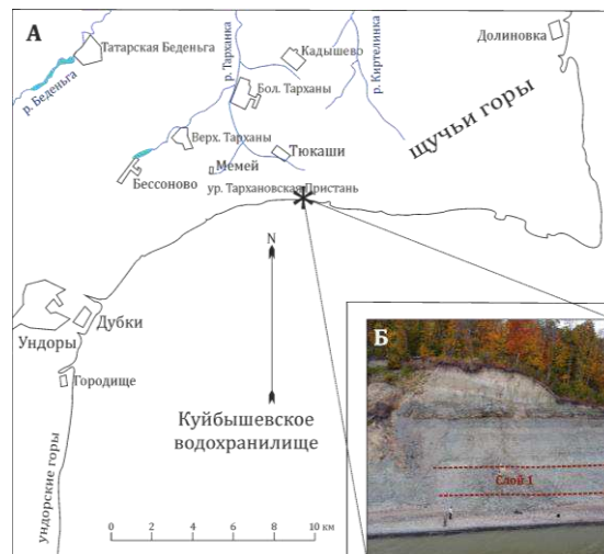
Рис. 1. Схема расположения обнажения Большие Тарханы в Ульяновском Поволжье:
