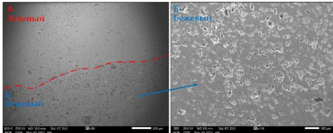
Рис. 1. Особенности микроструктур цеолитов различного типа: а – граница зеленой разности цеолита с однородной, плотной структурой и бежевой разности с пористой, туфогенной структурой; б – бежевая разность цеолита с пористой, туфогенной структурой
