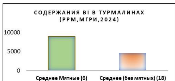
Рис. 4. Содержания Bi в турмалинах жил «Иркутянка» и «Геологическая» (Малханское месторождение) (ppm, МГРИ, 2024)
