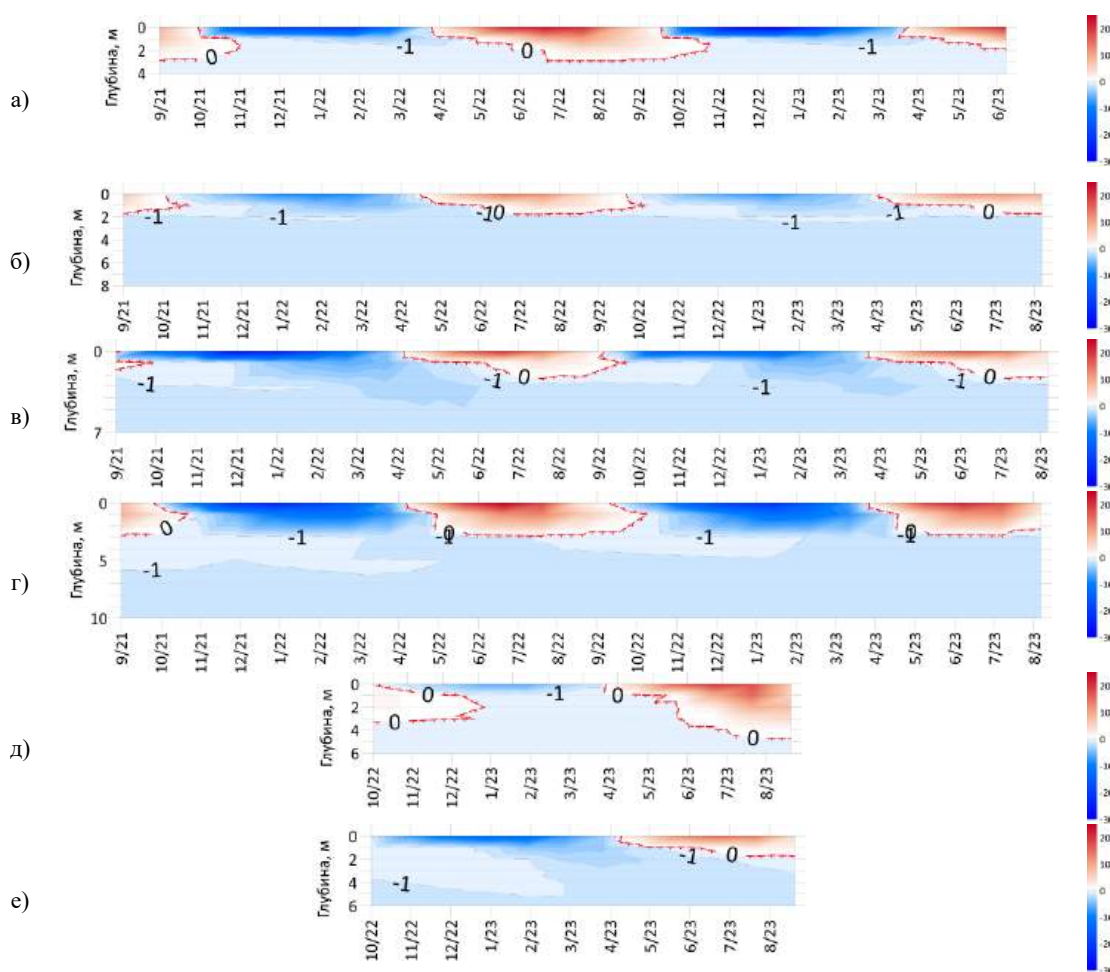
Рис. 2. Температурный режим в: а – с. Юнкюр скв. в поле (скв. 1), б – с. Юнкюр скв. в лесу (скв. 2), в – с. Амга скв. в лесу (скв. 3), г – с. Амга скв. в поле (скв. 4), д – с. Улахан-Ан скв. в поле (скв. 5), е – с. Улахан-Ан скв. в лесу (скв. 6)
