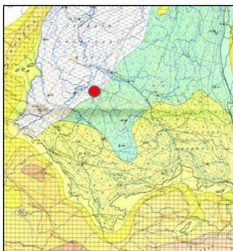
Рис. 1. Литолого-палеогеографическая карта (готеривский век) [1]: 1 – прибрежная равнина, 2 – мелкая часть шельфа
