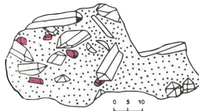
Рис. 1. Схематическое строение миаролы с камнесамоцветным сырьём в пегматите
