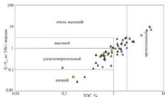
Рис. 5. Диаграмма изменения полного генерационного потенциала (S1+S2) от общего органического углерода TOC для выделенных пластов танопчинской свиты [3–5]. Условные обозначения см. на рис. 2
