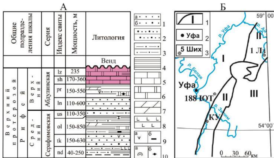
Рис. 1. Литолого-стратиграфическая колонка отложений рифея Камско-Бельского авлакогена (А) и обзорная карта (Б) с расположением изученных скважин [3, с изменениями].
