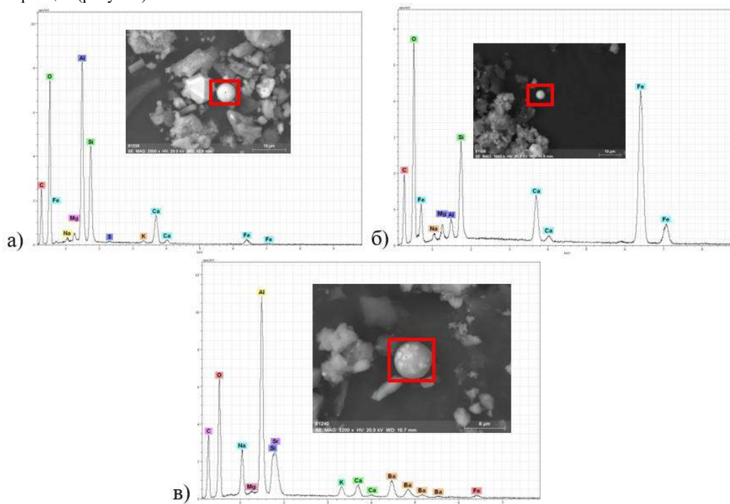
Рис. Фото и энергодисперсионные спектры микросферул в твердом осадке снежного покрова: а) алюмосиликатно-кальциевые; б) железосодержащие; в) алюмосиликатно-кальциевые с примесями бария и стронция
