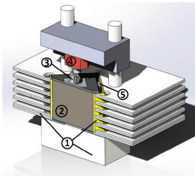
Рис. 1. лабораторного стенда для имитации процесса виброуплотнения дисперсных грунтов: 1 – станина и ребра жесткости; 2 – объем грунта в кубической клетки; 3 – дебалансный источник вибровоздействия; 4 – домкрат осевой нагрузки; 5 – плоский домкрат горизонтального сжатия
