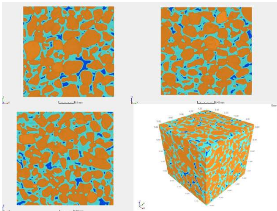
Рис. 1. Результаты микротомографии центральной части закрепленного массива (оранжевым цветом отмечены зерна песка; голубым – гель рабочего раствора; синим – свободное поровое пространство)
