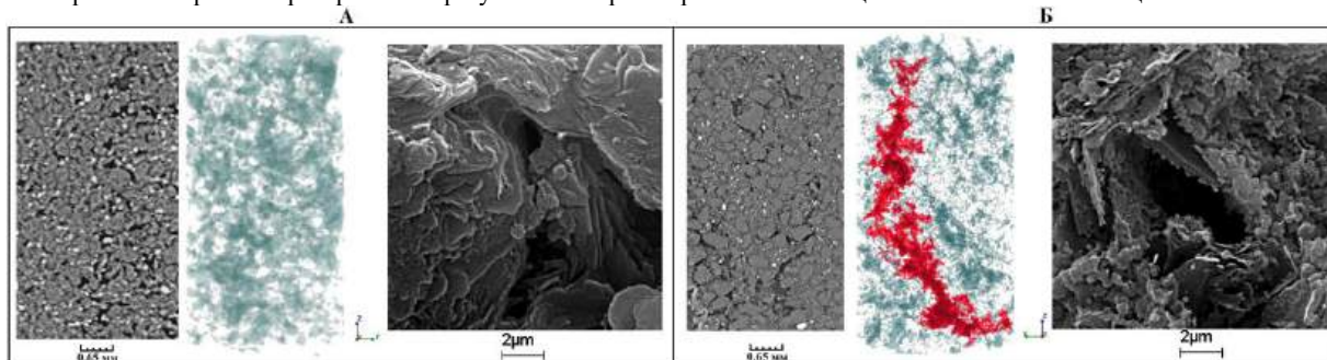
Рис. 2. Структура образцов по данным КТ и СЭМ (А – образец № 1; Б – образец № 2)
