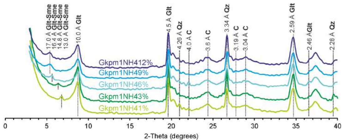
Рис. 1. РДА спектры нанокомпозитов, активированных с мочевиной (карбамидом). C – карбамид, Glt – глауконит, Qz – кварц
