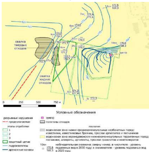
Рис. 1. Карта гидроизогипс карьерного водоотлива Ново-Сухоложского карьера аргиллитов
