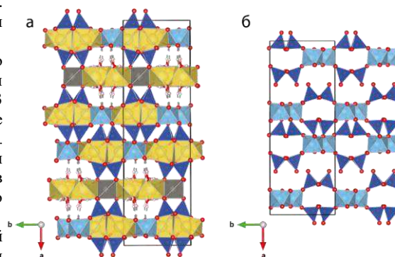
Рис. 2. Кристаллические структуры кукисвумита: а – исходного, б – декатионизированного
