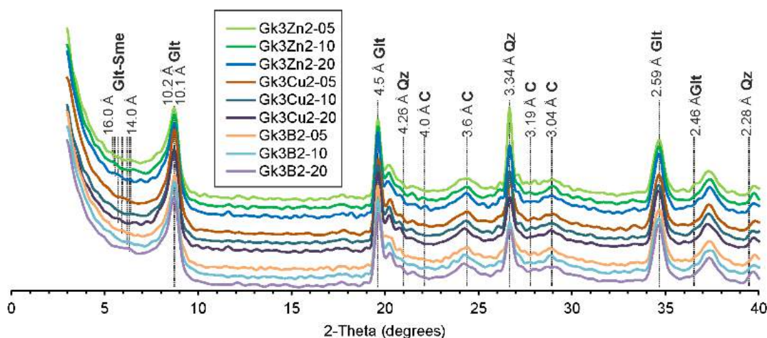
Рис. 1. Результаты интерпретации рентгенодифракционного анализа нанокompозитов
