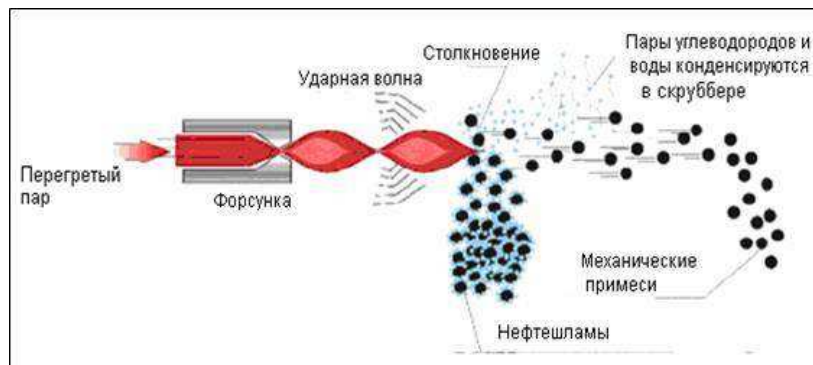
Рис. Термодесорбция буровых отходов
