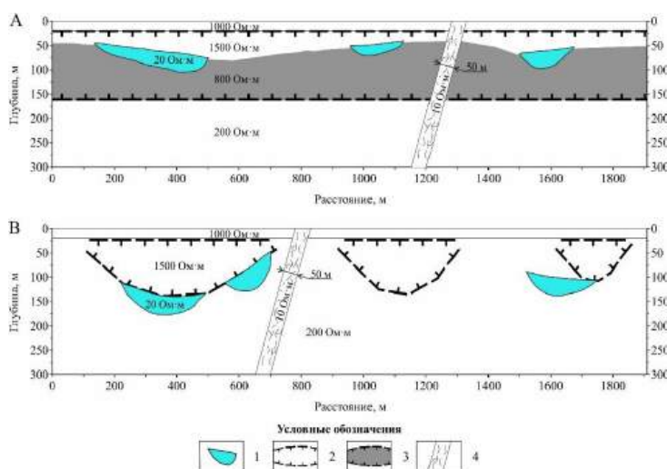
Рис. Геоэлектрические модели со сплошной мерзлотой (А) и с прерывистой мерзлотой (В): 1 – таликовая зона; 2 – высокотемпературные ММП; 3 – низкотемпературные ММП; 4 – разломная зона
