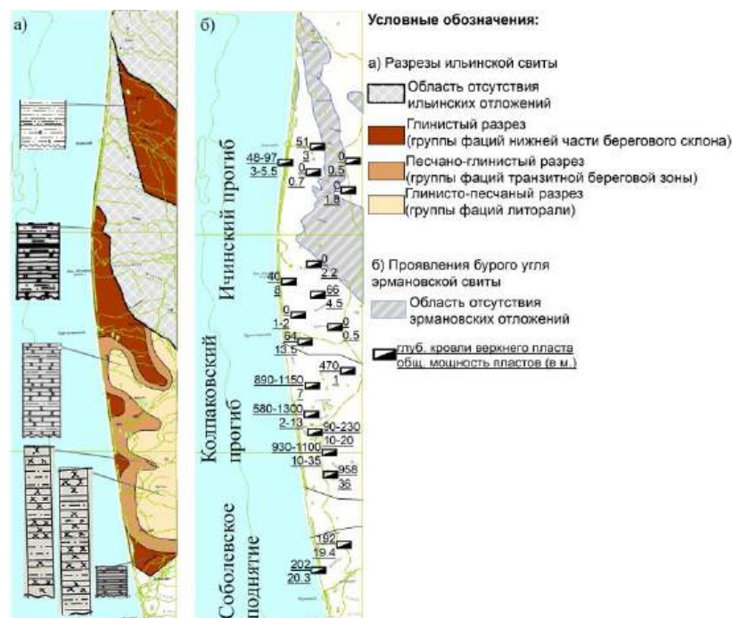
Рис. 1. Разрезы ильинской свиты (а), проявления бурого угля эрмановской свиты (б)
