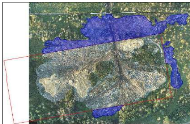
Рис. 3. Отображение частей полигона ТКО, выходящих за границы земельного участка
