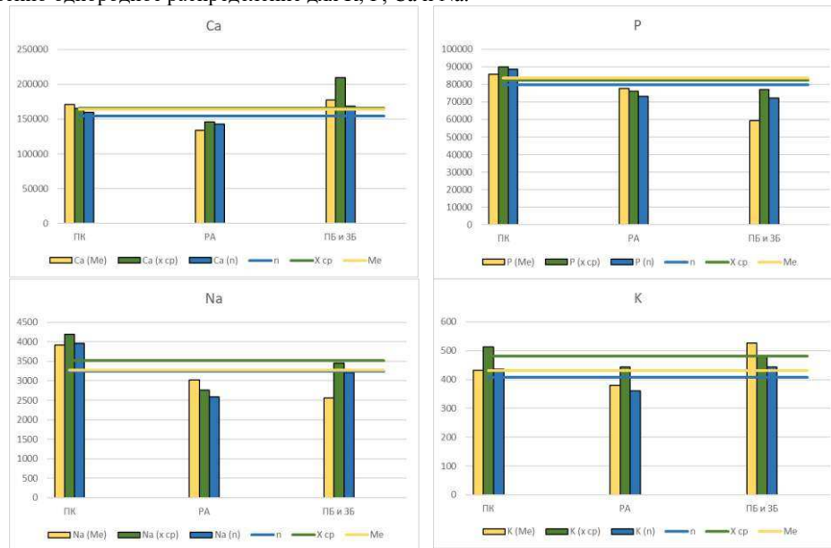
Рис. Содержание Ca, P, Na и K в бедренной кости млекопитающих Сибири и Дальнего Востока
