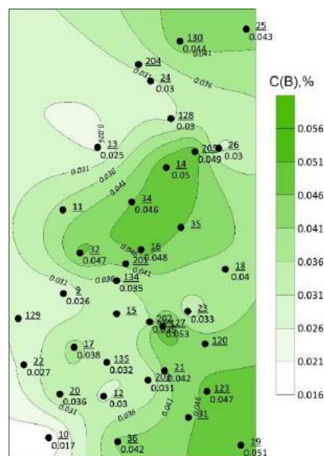
Рис. 3. Карта распределения относительного содержания бора
