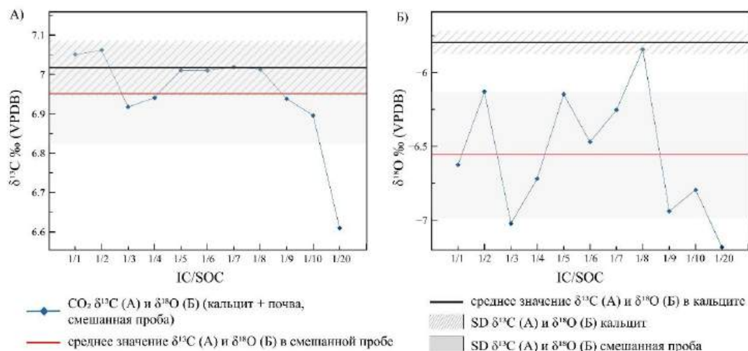
Рис. \delta^{13}\text{C} и \delta^{18}\text{O} в смешанных образцах (кальцит + почва) и образцах чистого кальцита. SD – стандартное отклонение, SIC – почвенный неорганический углерод, SOC – почвенный органический углерод
