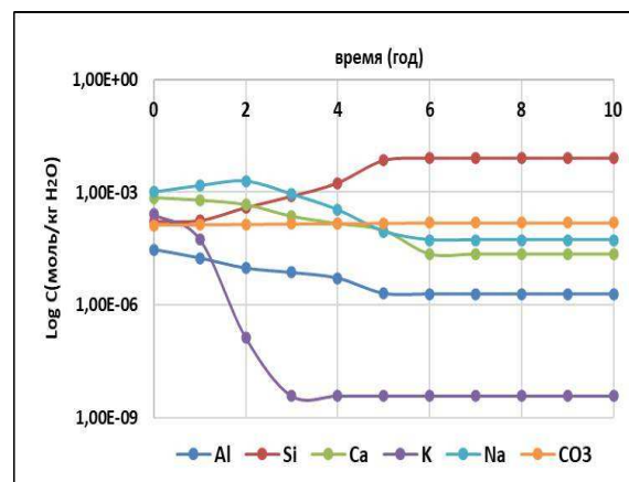
Рис. 2. Динамика концентраций ионов в растворе в течение периода моделирования
