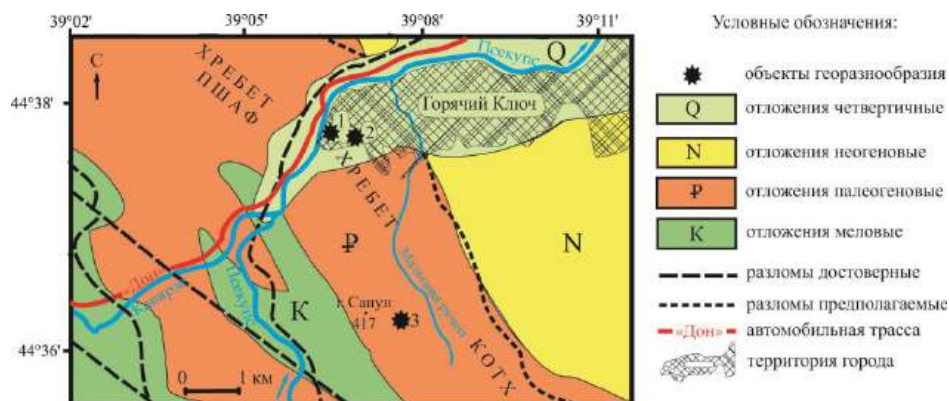
Рис. 1. Схема расположения объектов геологического наследия на хребте Котх [основа по 2 с упрощениями]: 1 – скала Петушок, 2 – Дантово ущелье, 3 – скала Зеркало
