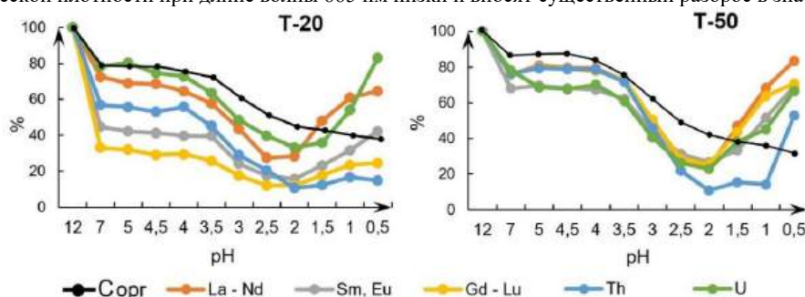
Рис. 1. Изменение концентрации органического углерода (Copr), РЗЭ, Th и U в щелочной вытяжке торфа в зависимости от pH в процентах от исходной концентрации в вытяжке; где La-Nd – сумма лёгких РЗЭ, Sm, Eu – их сумма как средних РЗЭ, Gd-Lu – сумма тяжелых РЗЭ
