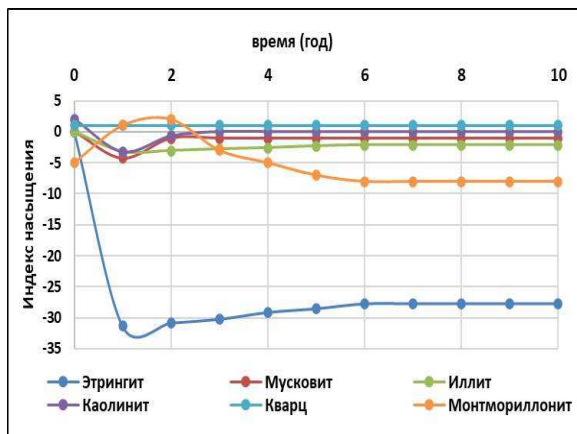
Рис. 3. Изменение индекса насыщения минералов в течение периода моделирования
