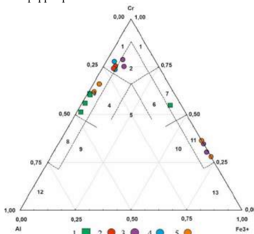
Рис. 2. Составы хромшпинелидов в ультрамафитах Кiemбаевского массива на классификационной диаграмме [3]: 1 – дуниты, 2 – лизардитовые серпентиниты, 3 – хризотилловые серпентиниты, 4 – антигорит-хризотилловые серпентиниты, 5 – лизардит-хризотил-антигоритовые серпентиниты. Поля на диаграмме: 1 – хромиты, 2 – субферрихромиты, 3 – алюмохромиты, 4 – субферриалюмохромиты, 5 – ферриалюмохромит, 6 – субалюмофер-рихромиты, 7 – феррихромиты, 8 – хромшпинелиды, 9 – субферрихромшпинелиды, 10 – субалюмохроммагнетиты, 11 – хроммагнетиты, 12 – пикотиты, 13 – магнетиты
