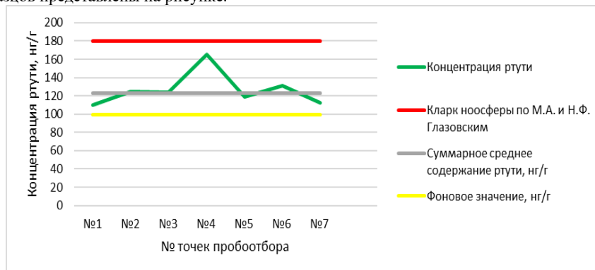
Рис. Содержание ртути в эпифитных лишайниках пгт. Зеленоборск ХМАО-Югра
