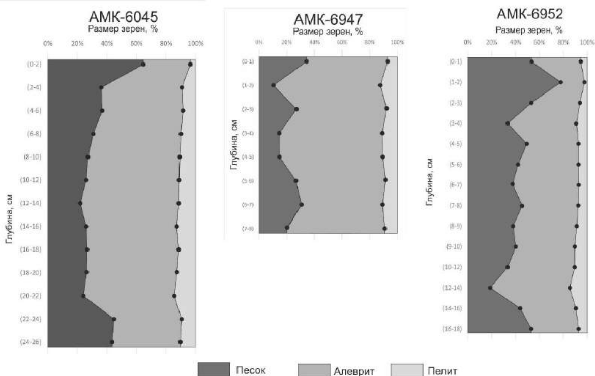
Рис. Вертикальное распределение размерных фракций донных осадков в изученных кернах
