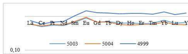
Рис. 2. Закономерности распределения нормированных РЗЭ пласта ПК 7 по РААС
