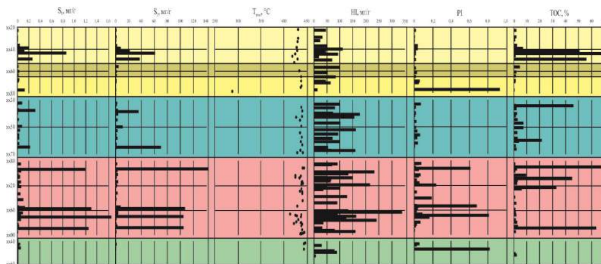
Рис. 1. Пиролитическая характеристика разреза танопчинской свиты
