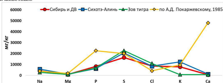
Рис. 1. Медианные концентрации макроэлементов в организме благородных оленей Приморского края в сравнении с млекопитающими Сибири и Дальнего Востока и белохвостыми оленями Северной Америки (мг/кг)
