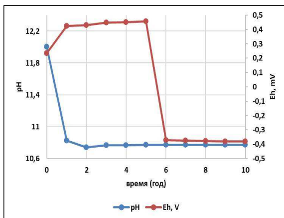
Рис. 1. Изменение значений pH и Eh раствора при взаимодействии с суглинками в течение периода моделирования
