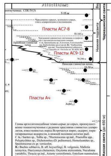
Рис. 2. Региональная стратиграфическая схема Приобско-Надымский район [3]
