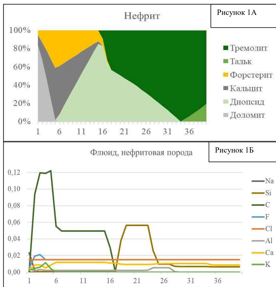
Рис. 1. Результаты моделирования нефритовой породы и флюида на ПК Селектор. На оси X отражены шаги протекания процесса, условное время. 1А – изменения минерального состава мрамора, содержание минералов в весовых %; 1Б – изменение состава водного флюида (значения компонентов в молях)
