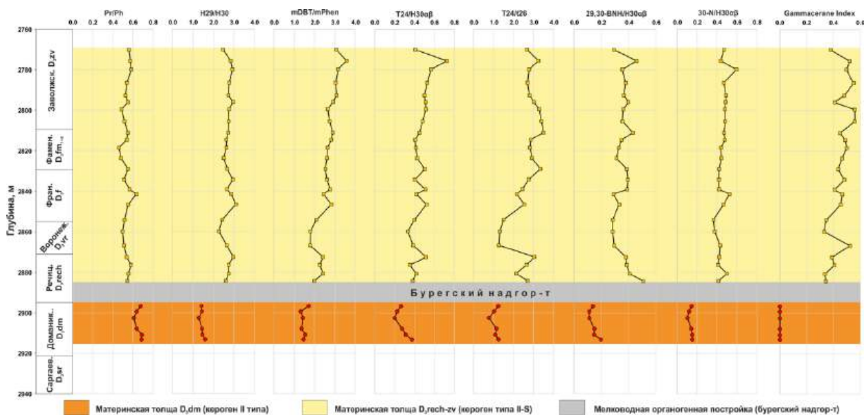
Рис. 1. Изменение фациально-генетических молекулярных параметров в разрезе доманиковых отложений одной из скважин Мухано-Ероховского прогиба
