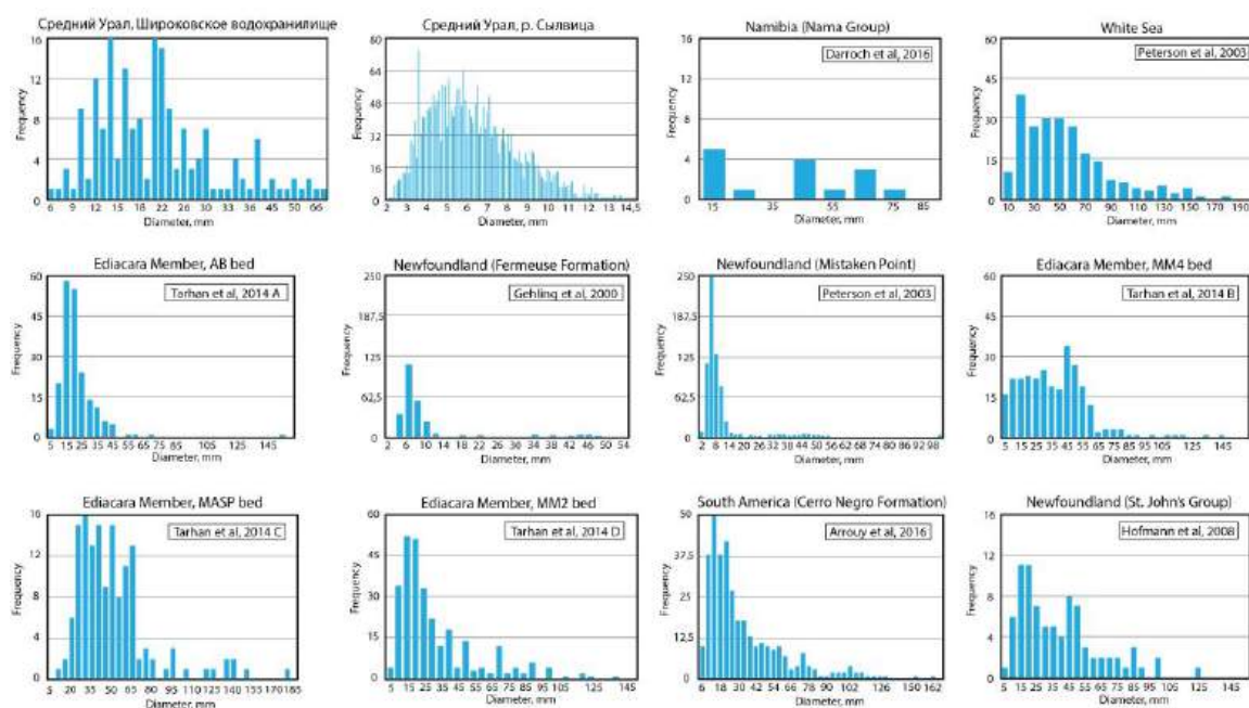
Рис. 2. Распределения размеров, полученные по данным из местонахождений на Среднем Урале (Широковское водохранилище и р. Сыльвица), а также из других регионов (Южная Австралия, Южная Америка, Ньюфаундленд, Намибия, Белое море)
