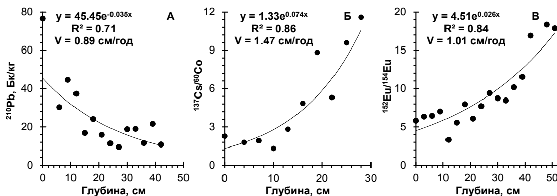
Рис. 1. Примеры расчёта скорости осадконакопления разными радиоизотопными методами: А) неравновесный ^{210}\text{Pb} ; Б) ^{137}\text{Cs}/^{60}\text{Co} ; В) ^{152}\text{Eu}/^{154}\text{Eu}
