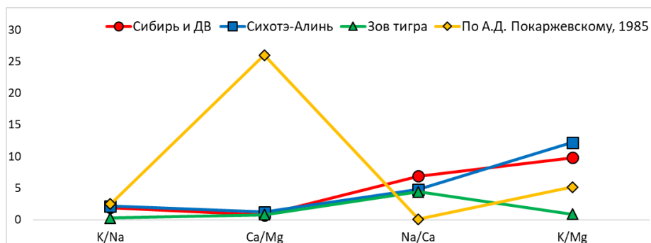
Рис. 2. Парные отношения некоторых макроэлементов в организме благородных оленей Приморского края в сравнении с млекопитающими Сибири и Дальнего Востока и белохвостыми оленями Северной Америки
