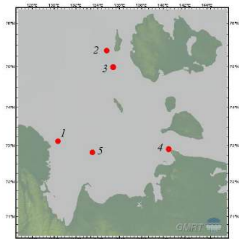
Рис. Расположение станций в юго-восточной части моря Лаптевых
