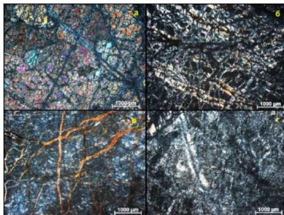
Рис. 1. Ультрамафиты Киембаевского массива: а – дуниты; б, в, г – серпентиниты: б – лизардитовые, в – хризотилитовые с жилками хризотил-асбеста, г – антигортитовые
