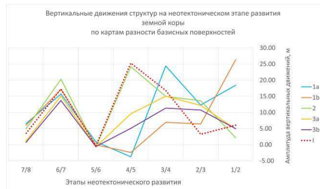
Рис. 2. Вертикальные движения структур на неотектоническом этапе развития земной коры по картам разности базисных поверхностей
