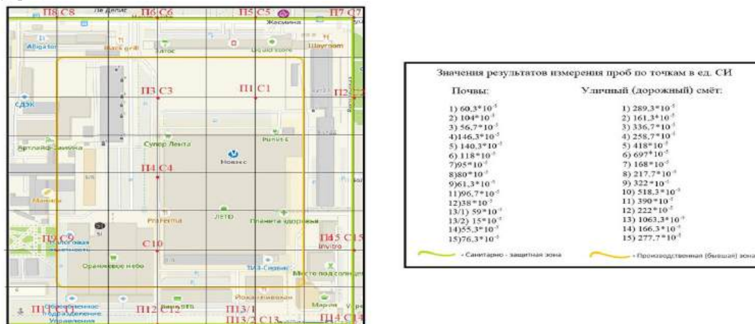
Рис. Схема отбора проб почво-грунтов и дорожной пыли на территории бывшего Томского инструментального завода
