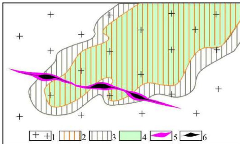
Рис. 1. Схема пространственных взаимоотношений метасоматитов и золотого оруденения в Центральном рудном поле: 1 – гранодиориты; кварцево-калийпат-биотитовые метасоматиты; 2 – калишпатизация; 3 – биотитизация; 4 – кварцево-эпидот-хлоритовые пропилиты; 5 – березиты; 6 – кварцево-золото-сульфидные жилы
