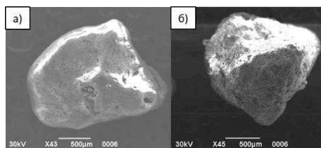
Рис. 3. Охра (а) и охристое образование (б)
