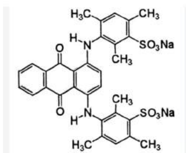
Рис. Структура красителя «Кислотный ярко-синий»
