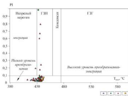
Рис. 2. Диаграмма соотношения индекса продуктивности PI и максимальной температуры пиролиза Tmax [3–5]. Примечание: 1 – ТП1-2; 2 – ТП6-8; 3 – ТП16-21; 4 – ТП24-27
