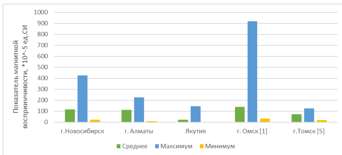
Рис. Сравнительная диаграмма значений показателя магнитной восприимчивости почв и почвогрунтов изученных территорий
