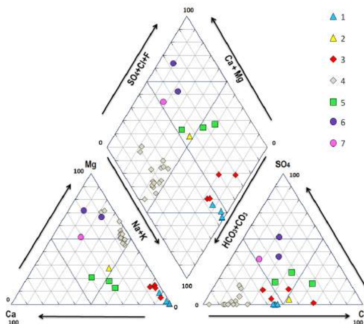
Рис. Пайпер-диаграмма химического состава поверхностных и подземных вод в районе исследования: 1 – подмерзлотные воды кембрийских отложений, 2 – воды четвертичных отложений подруслового талика р. Лены, 3 – воды озер на территории г. Покровск, 4 – воды озер в окрестностях п. Мохсоголлох, 5 – воды р. Лены, 6 – расплав повторно-жильных льдов, 7 – источник подземных вод
