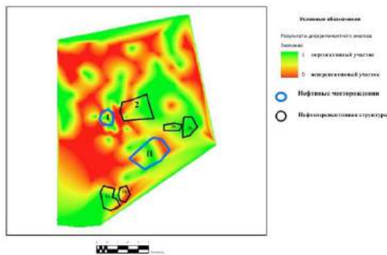
Рис. 1. Распределение территории по нефтеперспективности
