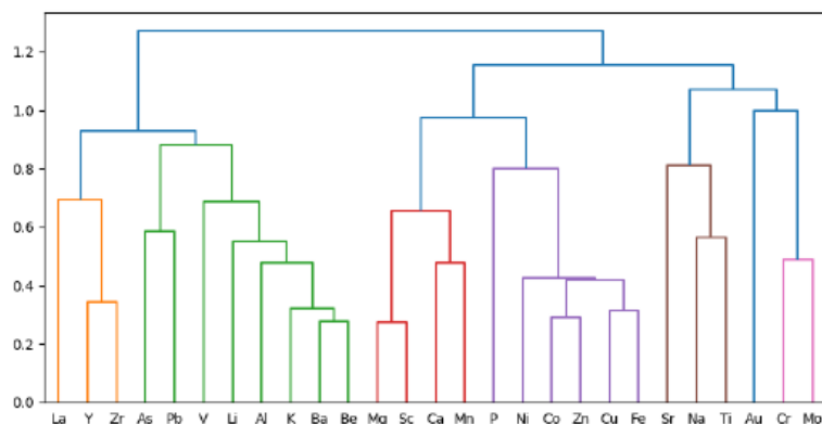
Рис. 1. Дендрограмма иерархической кластеризации нормированных данных ЛГХ
