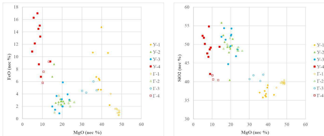
Рис. Бинарные диаграммы для ультрамафитов и мафитов Уктусского и Гальмознанского массивов Уктусский массив: У-1 – дуниты, У-2 – клинопироксениты, У-3 – верлиты, У-4 – габбро; Гальмознанский массив: Г-1 – дуниты, Г-2 – клинопироксениты, Г-3 – верлиты, Г-4 – габбро
