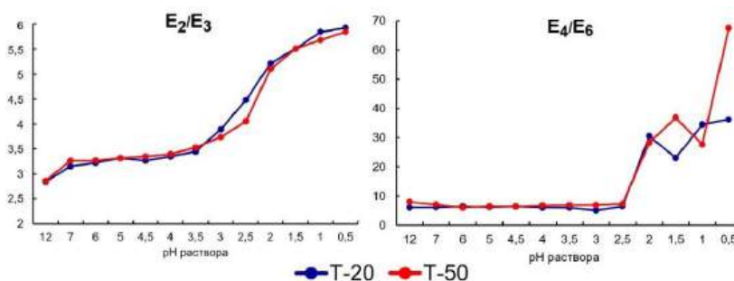
Рис. 2. Значения оптических дескрипторов гуминовых веществ при кислотном фракционировании
