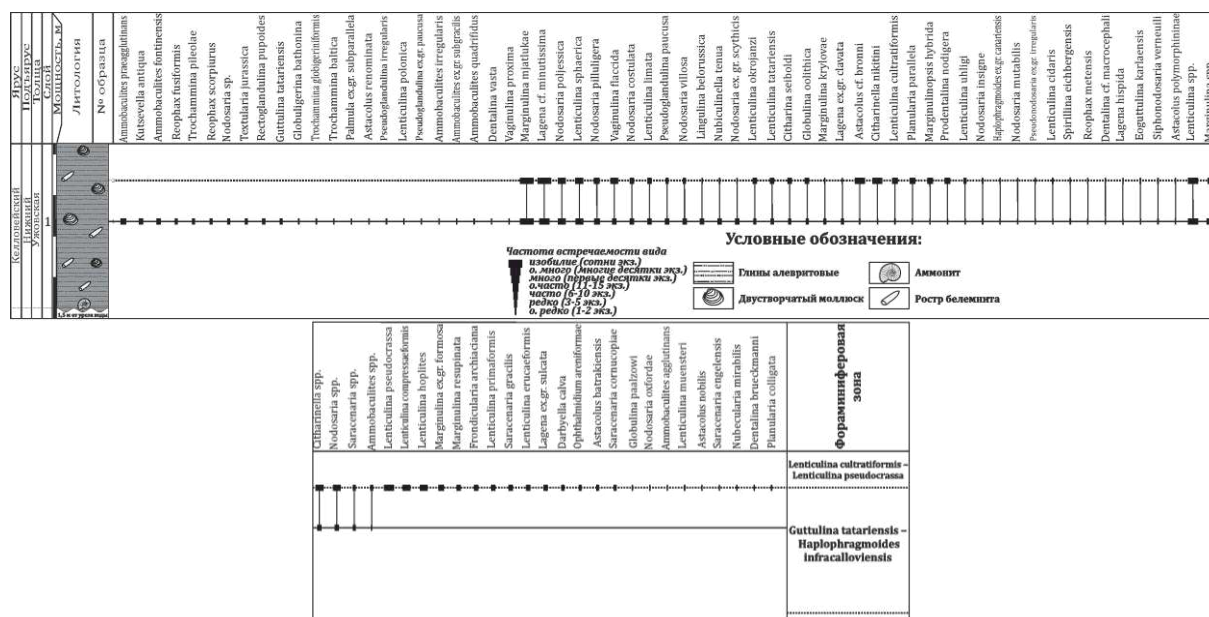
Рис. 2. Распределение фораминифер в нижнем – среднем келловее нижней части разреза Большие Тарханы, ур. Тархановская Пристань
