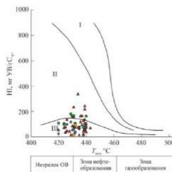
Рис. 3. Модифицированная диаграмма Ван-Кревелена зависимости водородного индекса HI от максимальной температуры пиролиза Tmax [3–5]. Усл. обозначения см. на рис. 2
