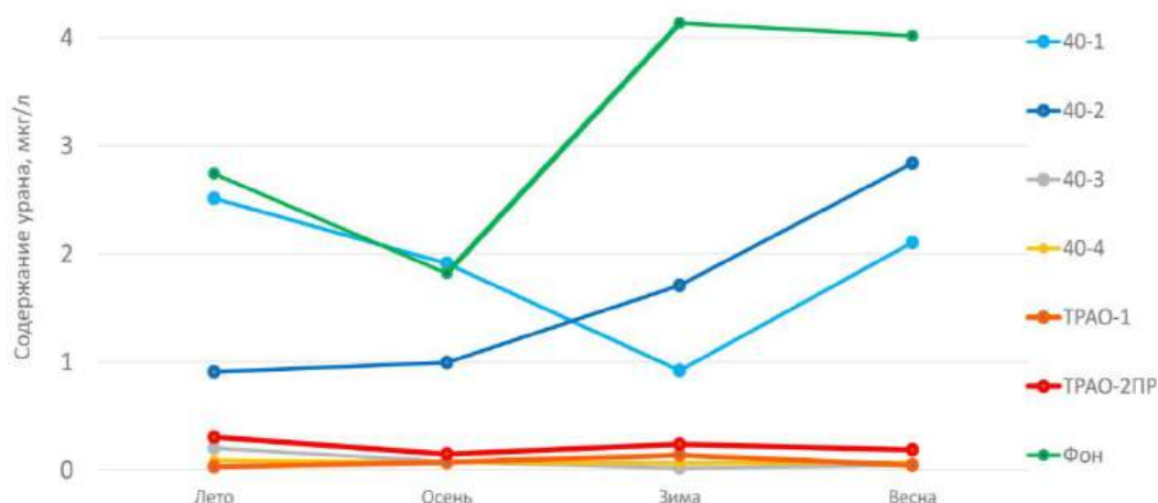
Рис. Сезонная динамика содержания U (мкг/л) в грунтовых водах в районе размещения хранилищ твердых радиоактивных отходов
