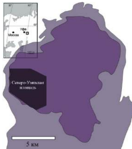
Рис. Расположение Северо-Уральской площади в пределах массива Северный Край
