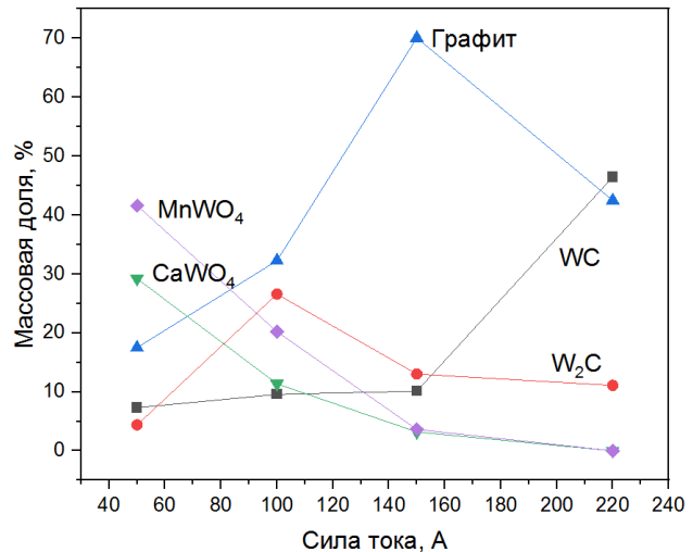
Рис. 2. Зависимость массовой доли фаз, содержащихся в продукте синтеза, от силы тока разрядного контура
