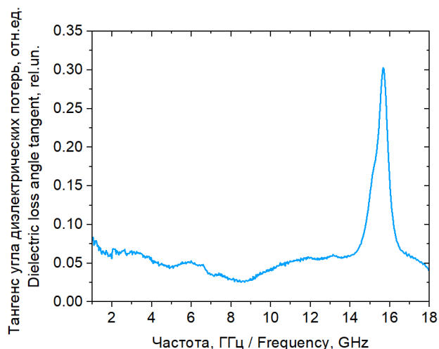
Рис. 3. Тангенс угла диэлектрических потерь в зависимости от частоты излучения
