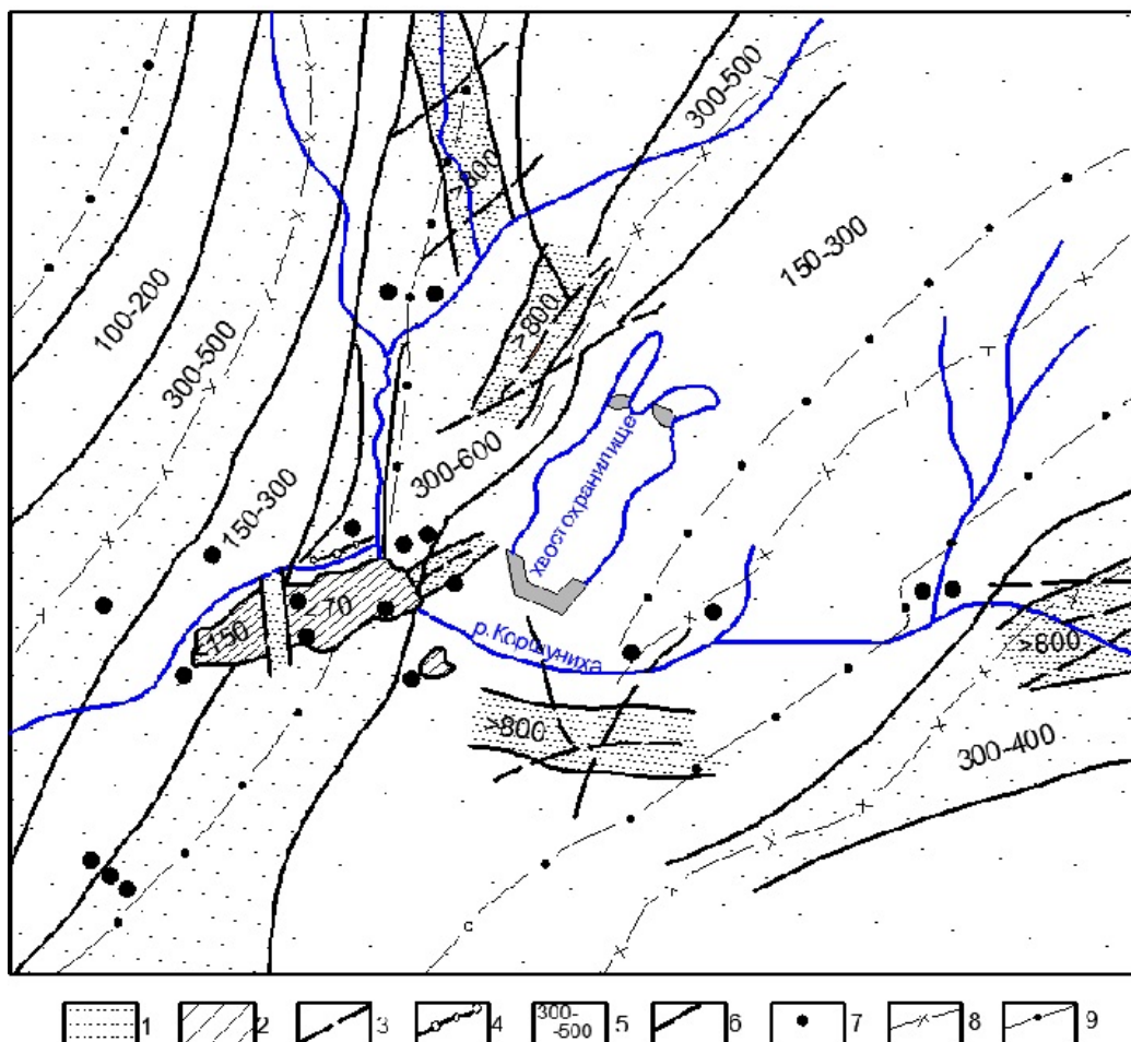
Рис. 2. Структурно-гидрогеологическая схема района Коршуновского железорудного месторождения (масштаб: 1:150000) [3]: 1 – гидрогеологические бассейны, интенсивность крапа характеризует степень водопроницаемости горных пород (максимальную в приосевых частях и минимальную на крыльях структур); 2 – кольцевые гидрогеологические массивы; 3, 4 – зоны разломов: 3 – обводненных, 4 – экранирующих; 5 – коэффициенты водопроводимости, м 2 /сут.; 6 – границы зон различной проводимости; 7 – точки наблюдения – эталоны (гидрогеологические скважины); 8, 9 – оси брахиформных структур: 8 – антиклинальных, 9 – синклинальных Fig. 2. Structural-hydrogeological diagram of the Korshunovskoye iron ore deposit area (map scale 1:150000) [3]: 1 – hydrogeological basins, speckle intensity characterizes water permeability degree of rocks (maximum degree in near-axial parts and minimum on structure flanks); 2 – ring hydrogeological massifs; 3, 4 – fault zones: 3 – flooded, 4 – screening; 5 – permeability coefficients, m 2 /day; 6 – boundaries of variable permeability zones; 7 – reference observation points (hydrogeological wells); 8, 9 – axes of brachiform structures: 8 – anticlinal, 9 – synclinal
