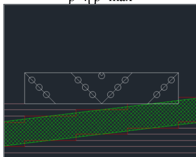
Рис. 1. Технологические схемы образования потерь и засорения полезного ископаемого при отработке слабонаклонных залежей фрезерным комбайном [27]
