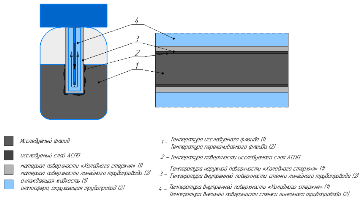
Рис. 1. Принцип работы лабораторной установки «Холодный стержень»
