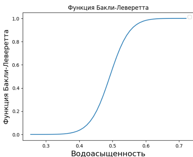
Рис. 2. Функция Баклея–Лeverетта Fig. 2. Buckley–Leverett function
