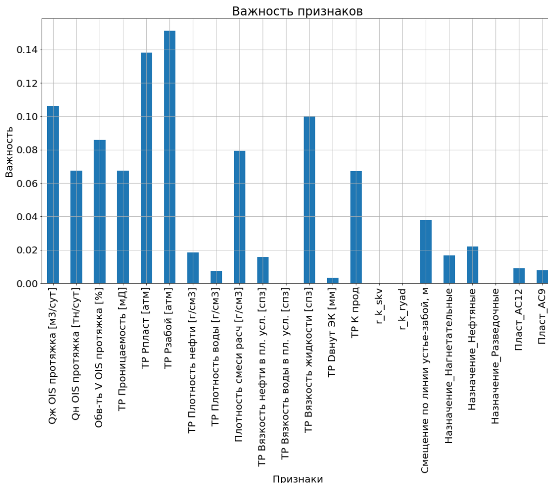
Рис. 2. Исследование важности признаков Fig. 2. Research of the importance of features
