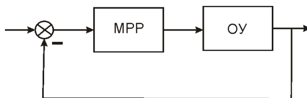
Рис. 1. Структура САУ с МРР
