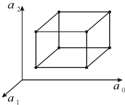
Рис. 2. Область возможных значений коэффициентов полинома
