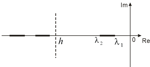
Рис. 3. Расположение отрезков вещественных корней
