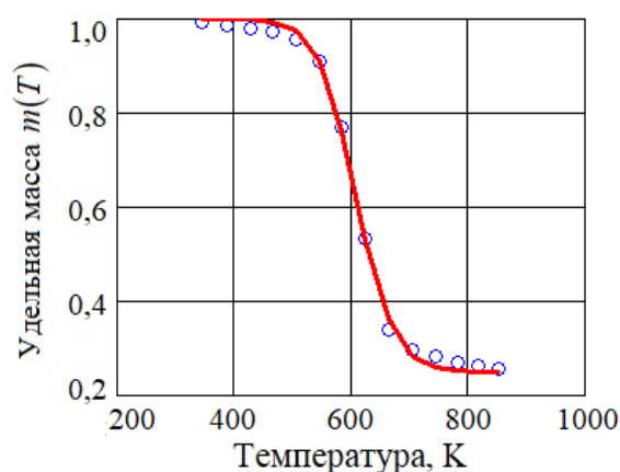
Рис. 8. Температурные зависимости удельной массы пиролизуемой пеллеты по данным ТГА, полученным авторами: кривая – расчетная зависимость с параметрами A и E (23); кружки – экспериментальные точки, снятые с кривой ТГА (рис. 2)
